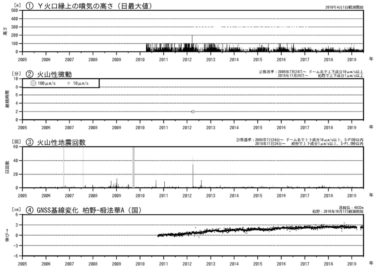
図2 恵山 火山活動経過図（2005年7月～2019年6月）
