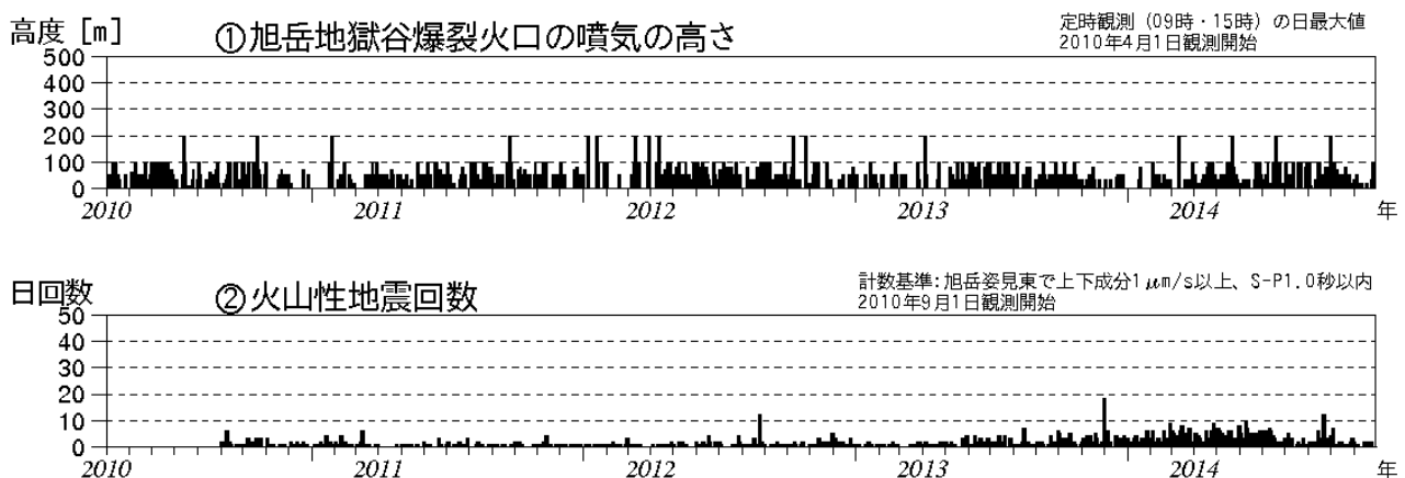
図1 大雪山 火山活動経過図（2010年4月～2014年11月）
