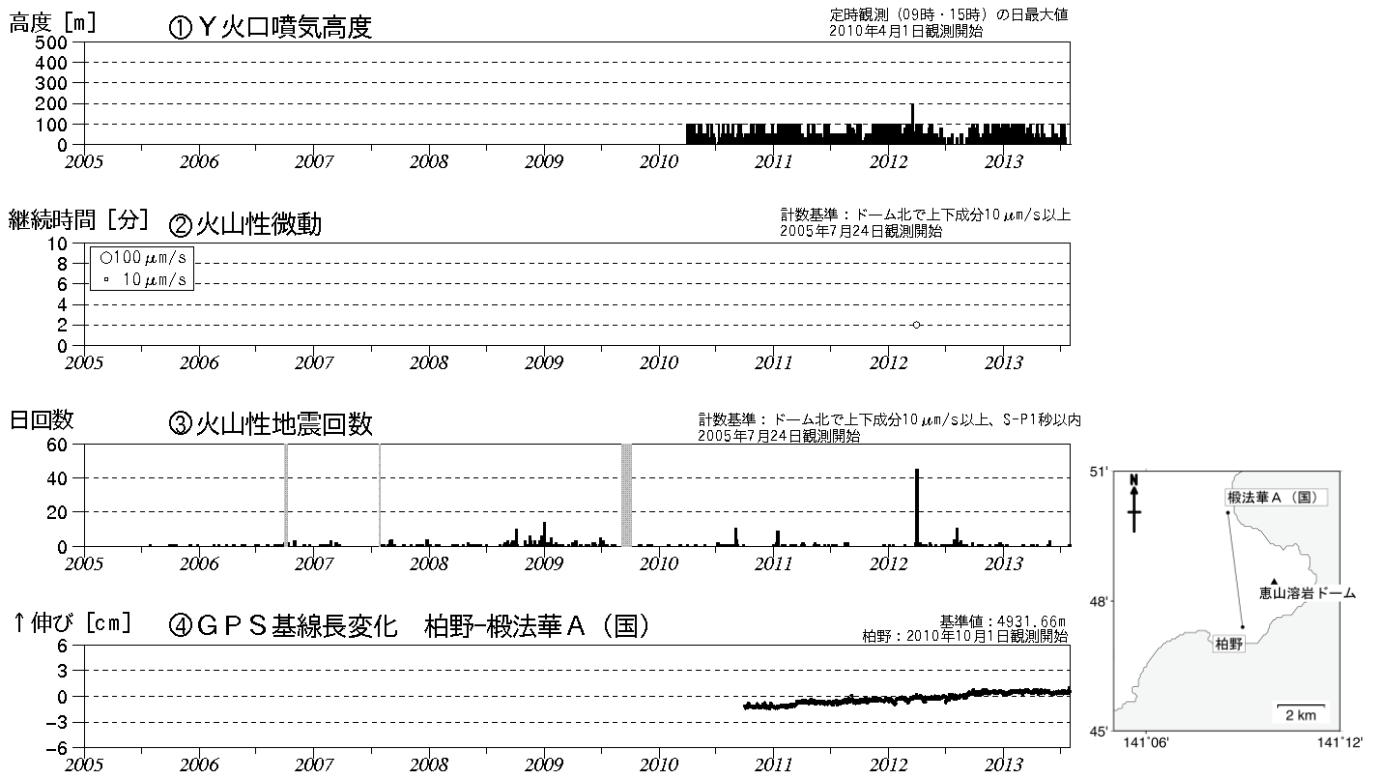
図 2 恵山 火山活動経過図（2005年 7 月～2013年 7 月）、GPS連続観測点配置図
