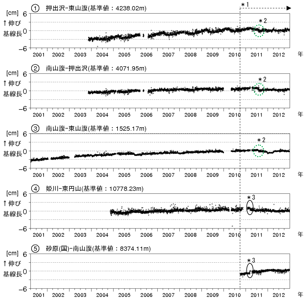
図 4 ※ 北海道駒ヶ岳 GPS連続観測による基線長変化 (2001年 4 月～2012年12月)
