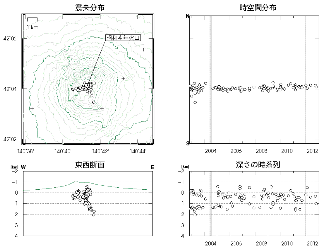
図3※ 北海道駒ヶ岳 火山性地震の震源分布（2002年11月～2012年12月） 灰色の期間は一部観測点欠測のため震源の決定数減少や精度低下が見られます ○印：2002年11月から2012年11月の震源 +印：地震観測点
