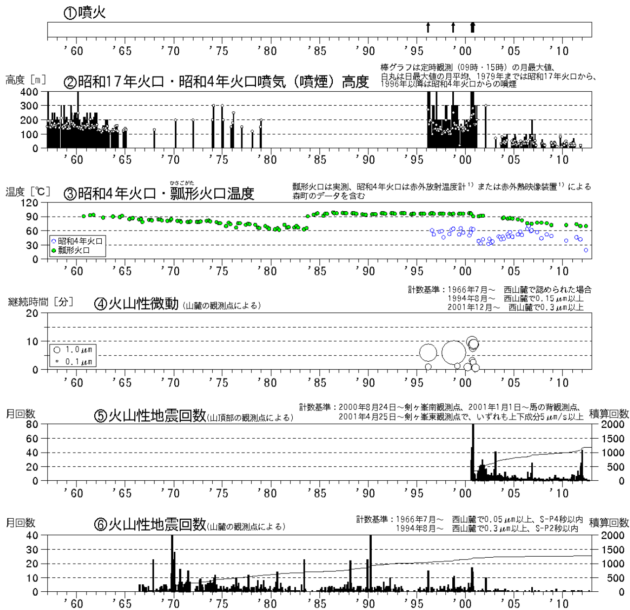
図 1 ※ 北海道駒ヶ岳 火山活動経過図（1957年 1 月～2012年12月）
