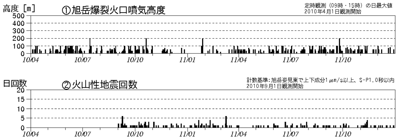
図 1 大雪山 火山活動経過図（2010 年 4 月～2011 年 12 月）
