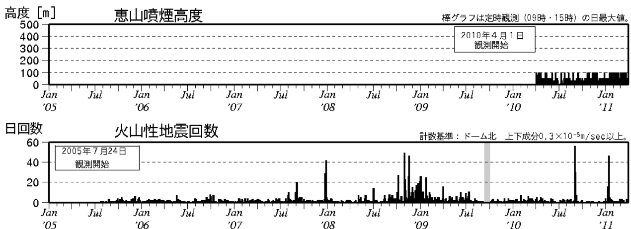
図 1 恵山 最近の火山活動経過図（2005 年 7 月～2011 年 3 月）
