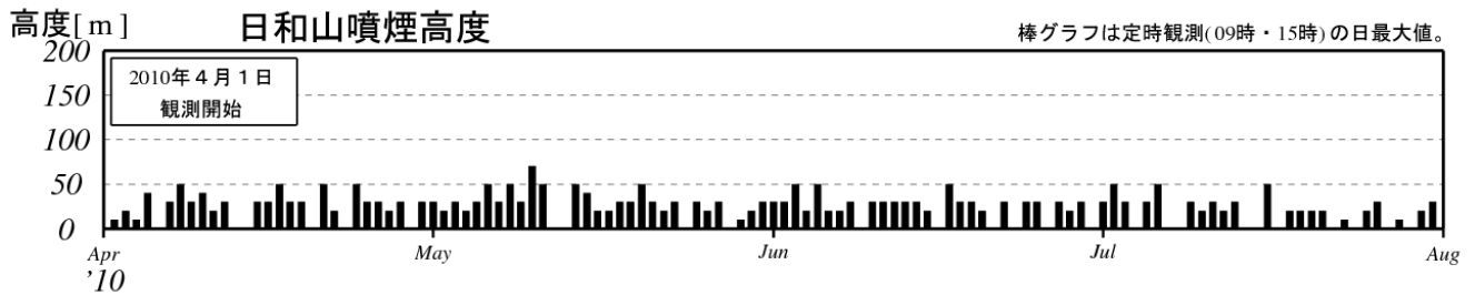
図2 倶多楽 日和山噴煙高度グラフ（2010年4月～7月）
