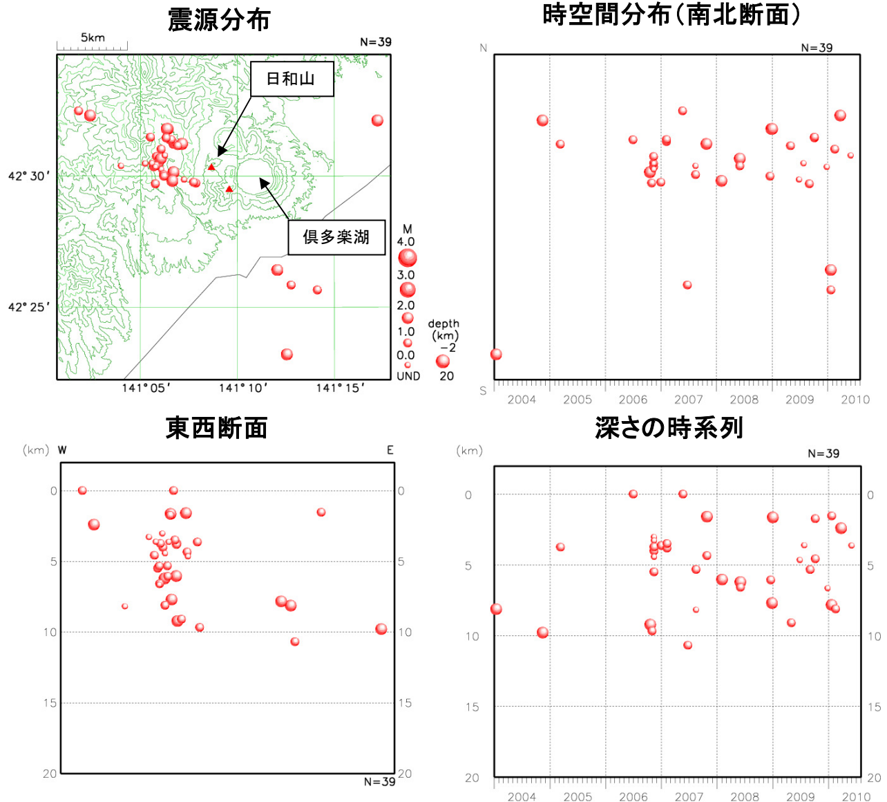
図3 広域ネットによる倶多楽周辺の地震活動（2004年1月～2010年7月）
