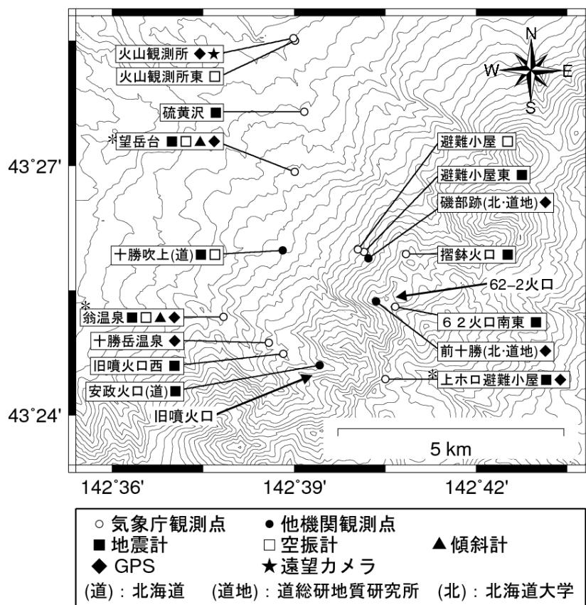
図 7 十勝岳 新しい観測点名称を使用した観測点配置図
