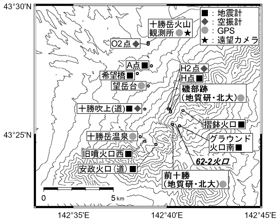
図 6 十勝岳 従来の観測点配置図
