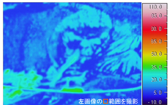
図3 ニセコ 赤外熱映像装置*により撮影した五色温泉付近の表面温度分布 (2007年5月22日 図2 ②方向から撮影)
