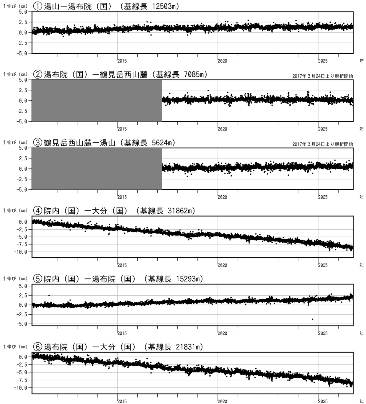
図 4 鶴見岳・伽藍岳 GNSS連続観測による基線長変化（2010 年 10 月～2026 年 9 月）
