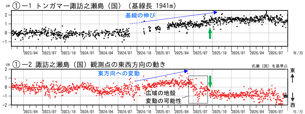
図 5-1 諏訪之瀬島 GNSS連続観測（2023 年 2 月～2026 年 9 月）
