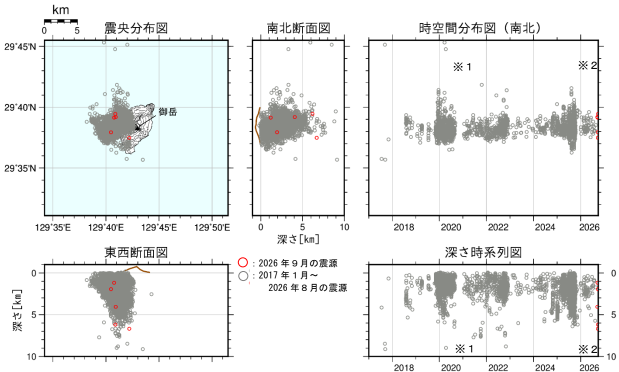
図4 諏訪之瀬島 震源分布図（2017年1月～2026年9月）
