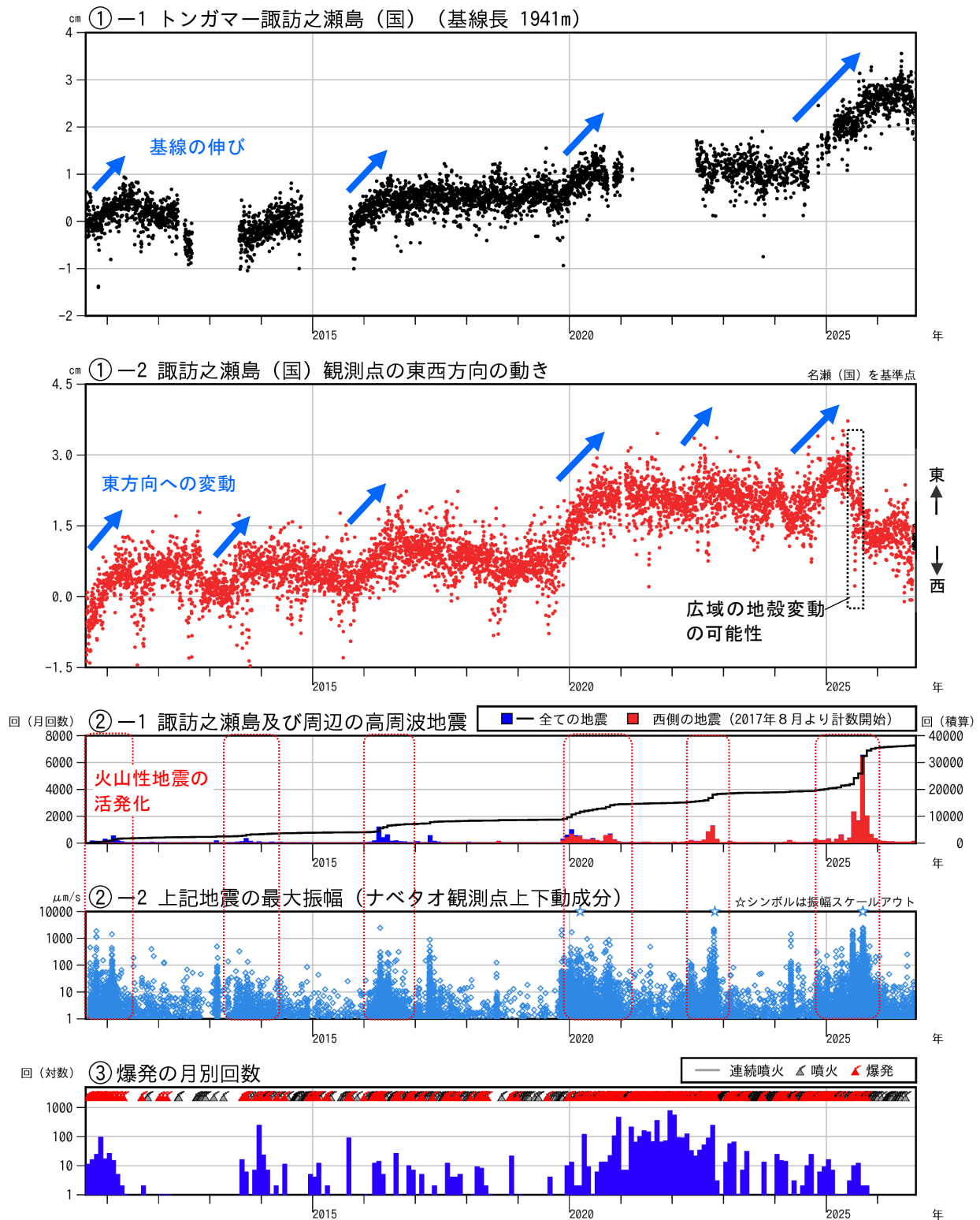
図 5-2 諏訪之瀬島 GNSS連続観測と周辺の火山性地震（2010 年 8 月～2026 年 9 月）
