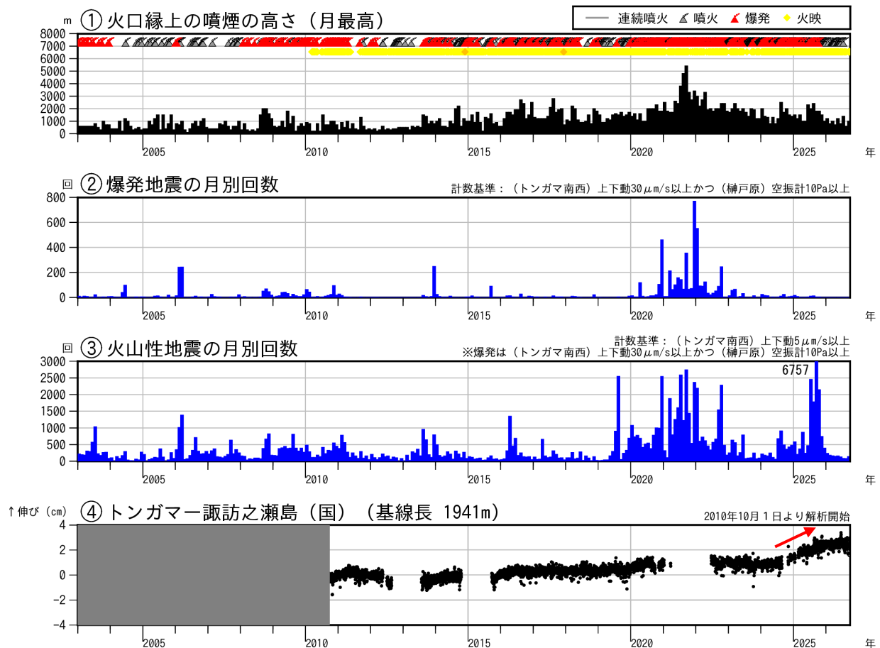
図2 諏訪之瀬島 長期の火山活動経過図（2003年1月～2026年9月）
