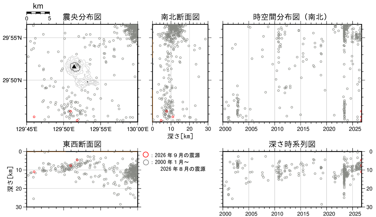
図3 中之島 中之島周辺の震源分布図（2000年1月～2026年9月）
