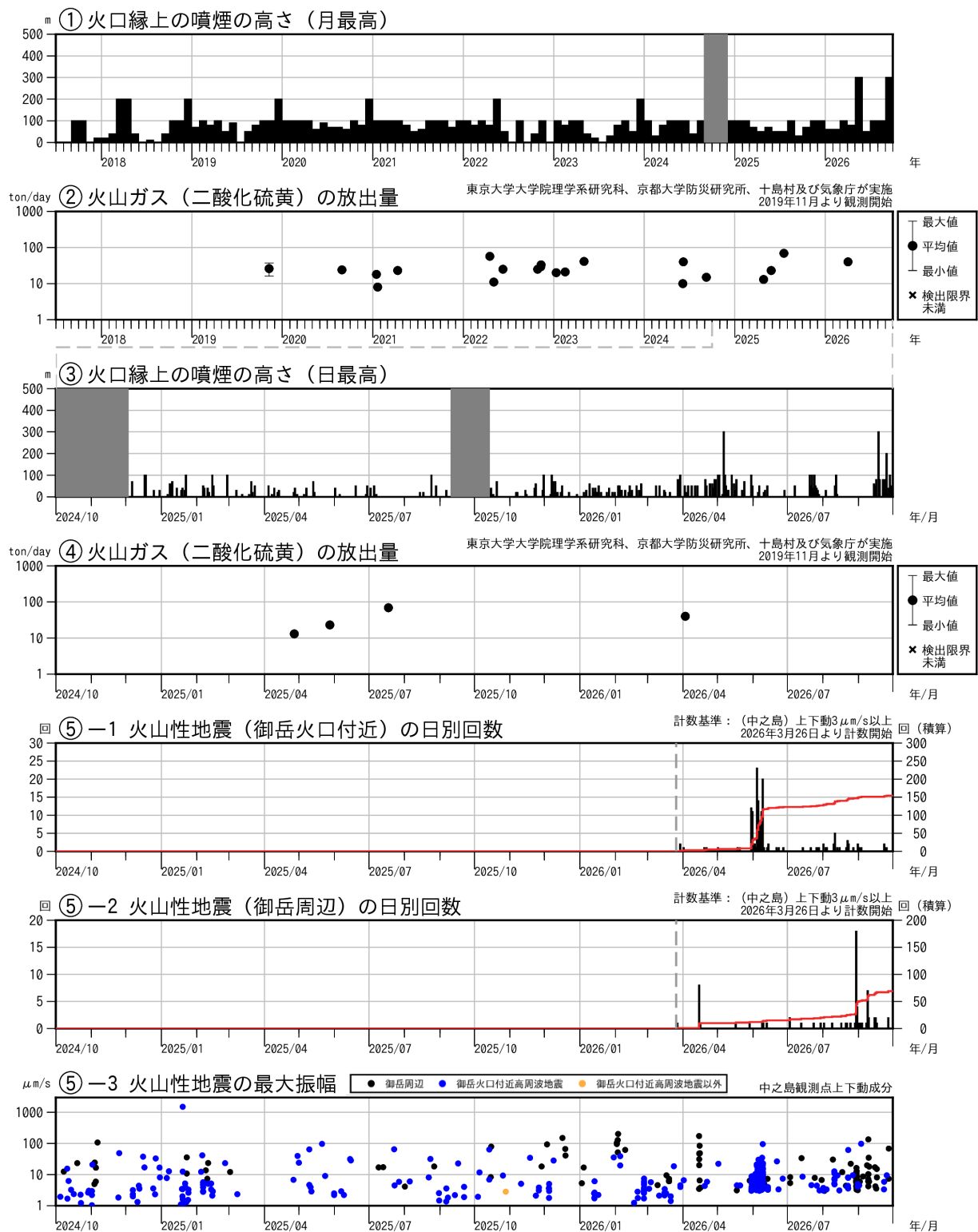
図2 中之島 火山活動経過図（2017年7月～2026年9月）
