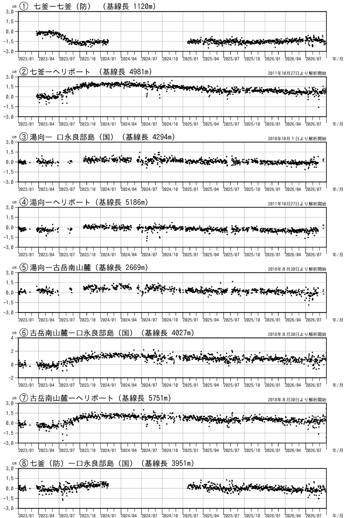
図 7-2 口永良部島 GNSS 連続観測による基線長変化（2023 年 1 月～2026 年 9 月）
