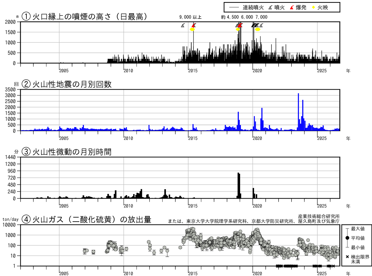
図4 口永良部島 火山活動経過図（2002年1月～2026年9月）
