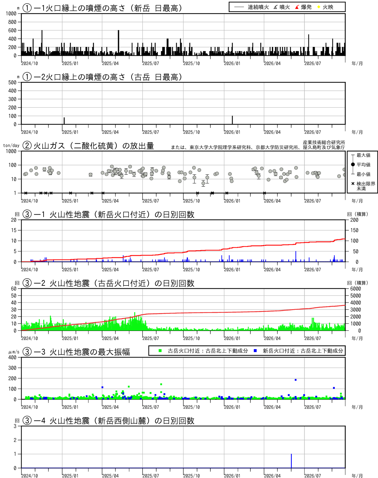
図5 口永良部島 最近の火山活動経過図（2024年10月～2026年9月）
