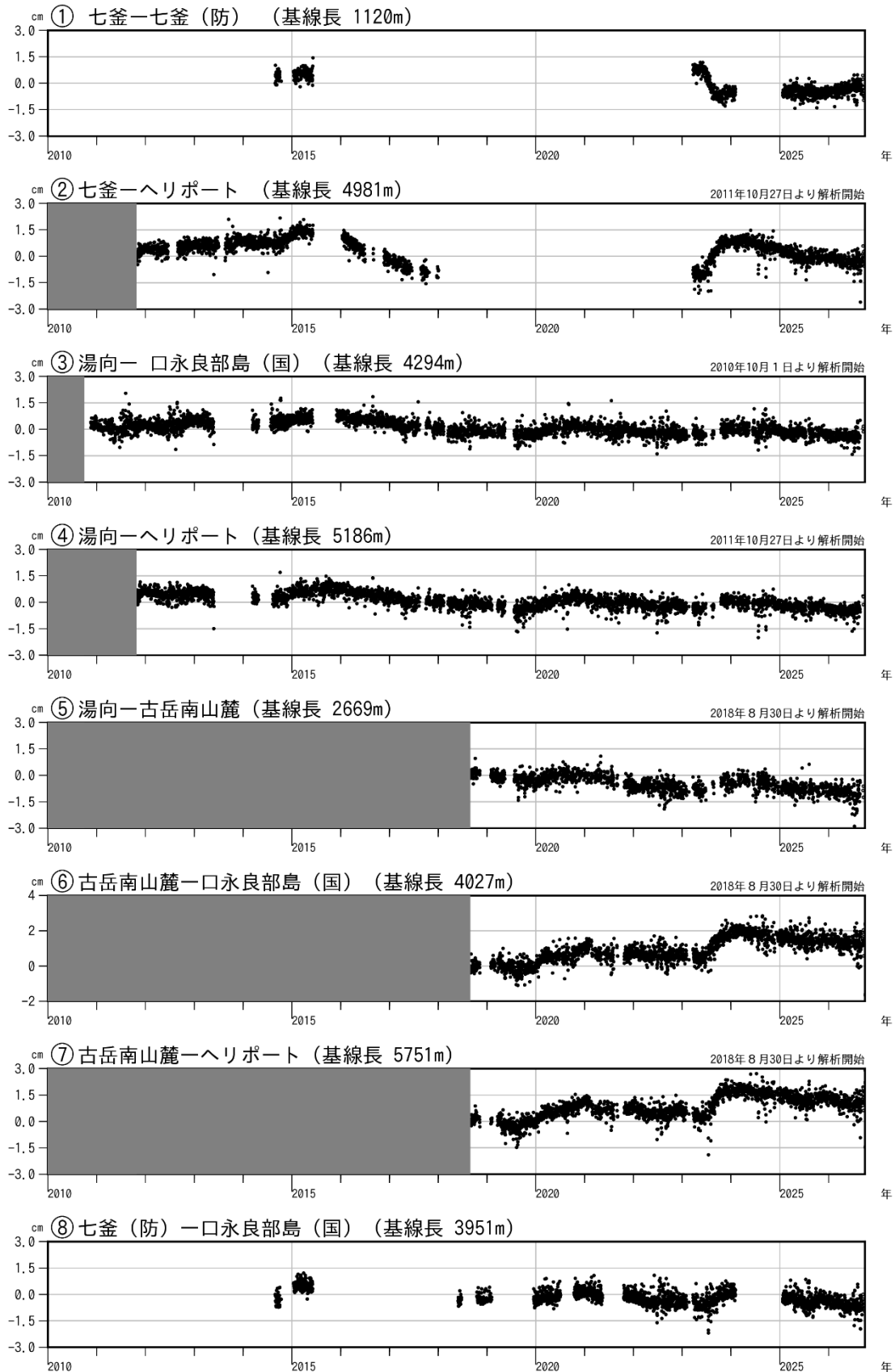
図 7-1 口永良部島 GNSS 連続観測による基線長変化（2010 年 1 月～2026 年 9 月）
