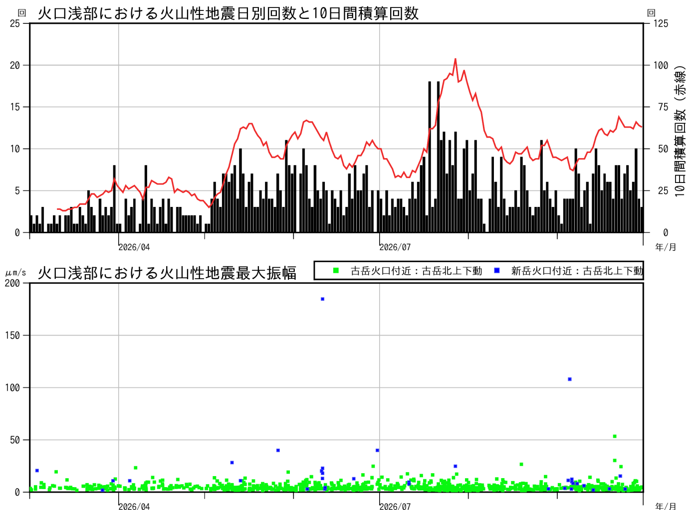
図1 口永良部島 火口浅部における火山性地震発生状況（2026年3月～9月）
