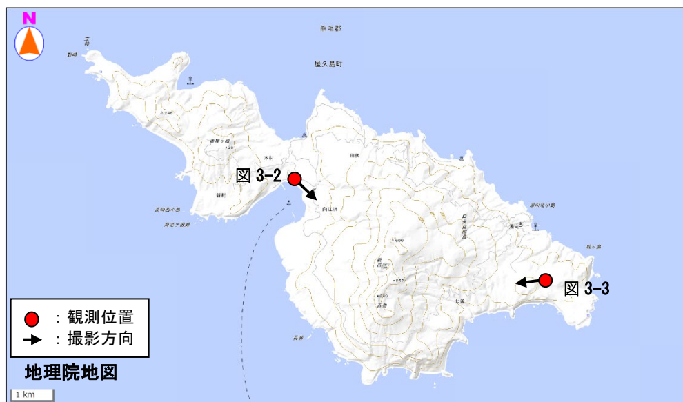
図3-1 口永良部島 観測位置及び撮影方向
