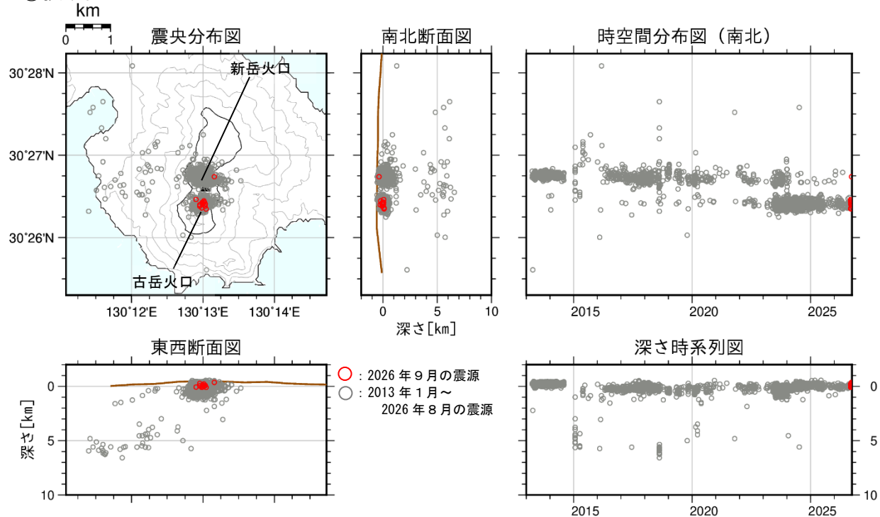
図6 口永良部島 震源分布図 ①広域図 ②狭域図（2013年1月～2026年9月）
