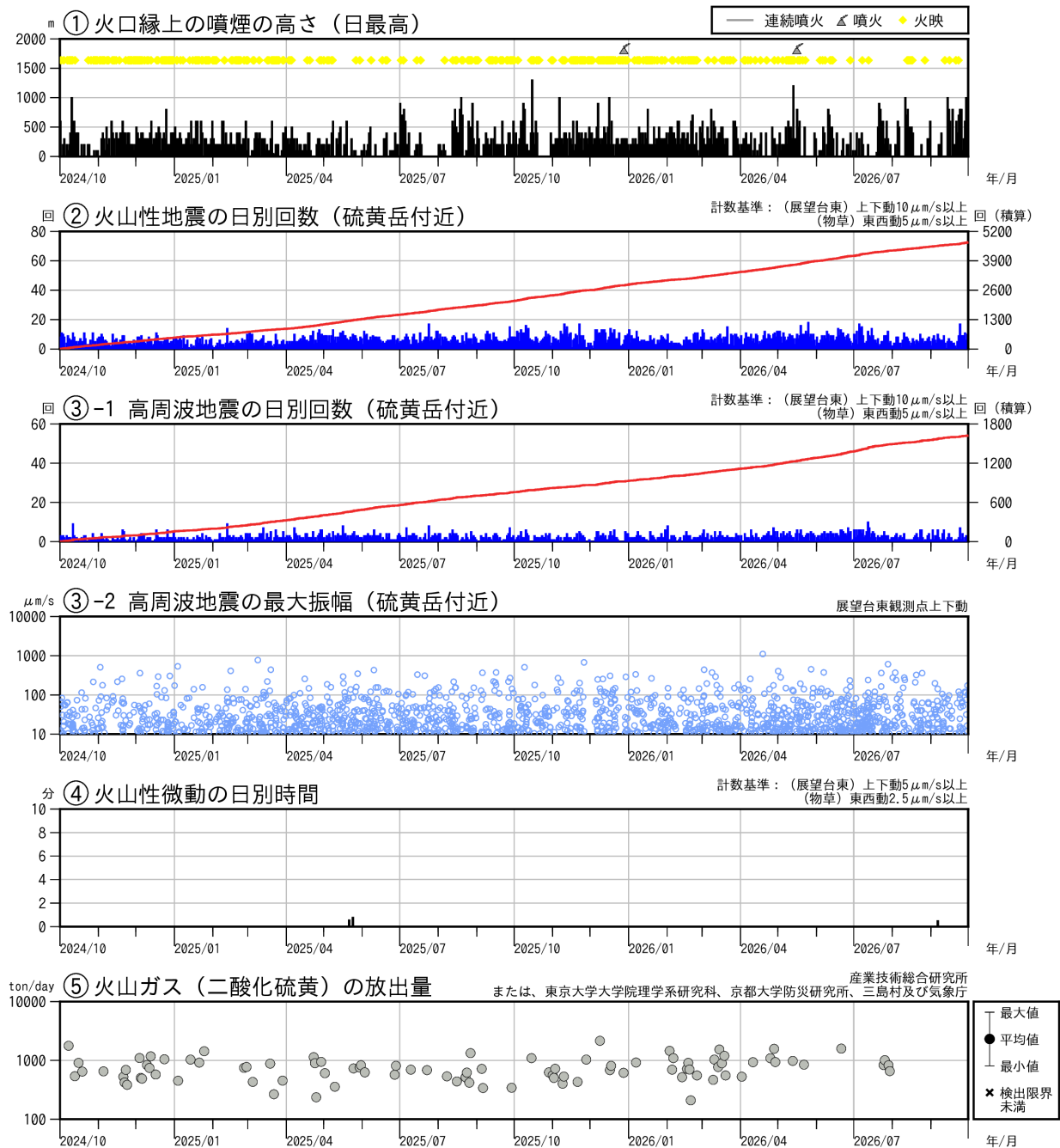
図3 薩摩硫黄島 火山活動経過図（2024年10月～2026年9月）
