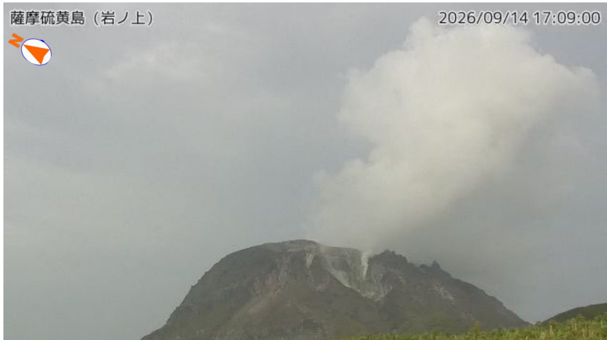
図1-1 薩摩硫黄島 噴煙の状況（9月14日、岩ノ上監視カメラ）
