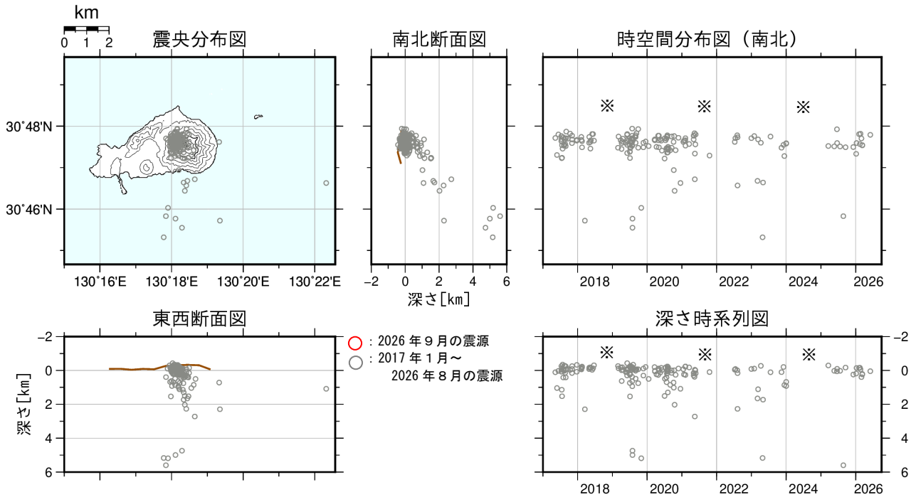
図4 薩摩硫黄島 火山性地震の震源分布図（2017年1月～2026年9月）
