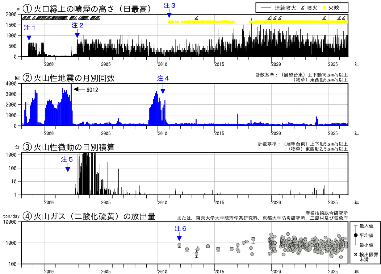
図2 薩摩硫黄島 火山活動経過図（1998年1月～2026年9月）
