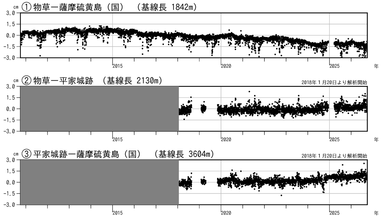
図5 薩摩硫黄島 GNSS連続観測による基線長変化（2010年10月～2026年9月）
