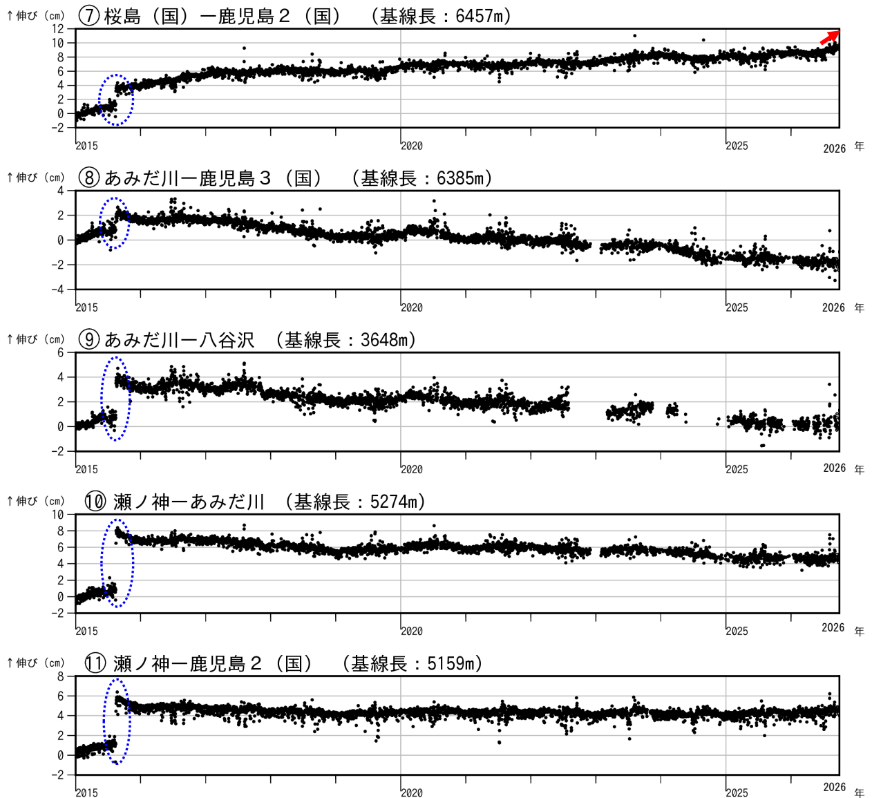
図 7-2 桜島 GNSS 連続観測による基線長変化（2015 年 1 月～2026 年 9 月）
