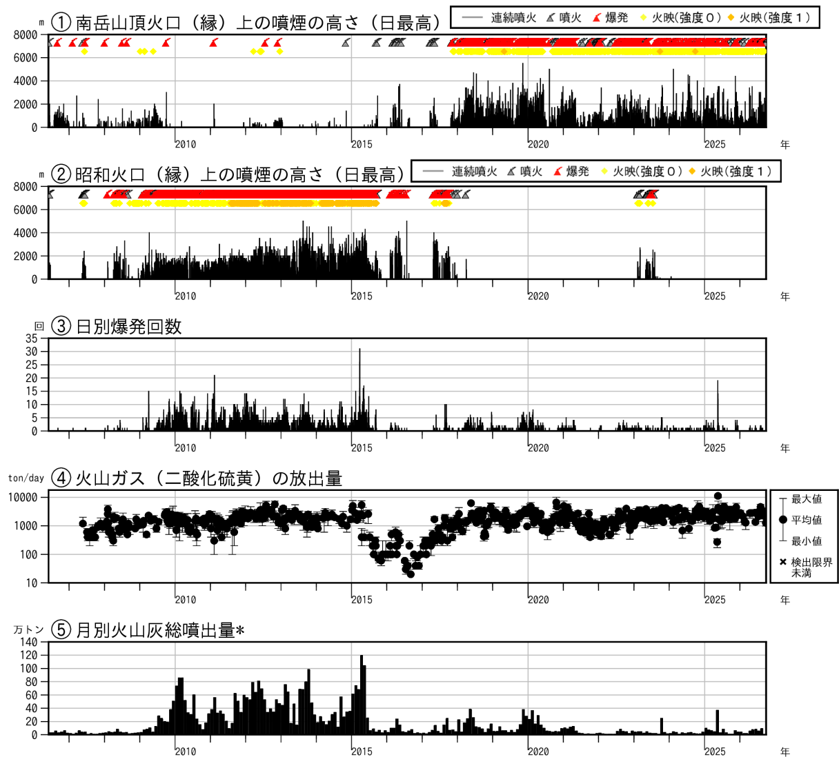
図 5-1 桜島 昭和火口噴火活動再開（2006 年 6 月）以降の活動経過図（2006 年 6 月～2026 年 9 月）
