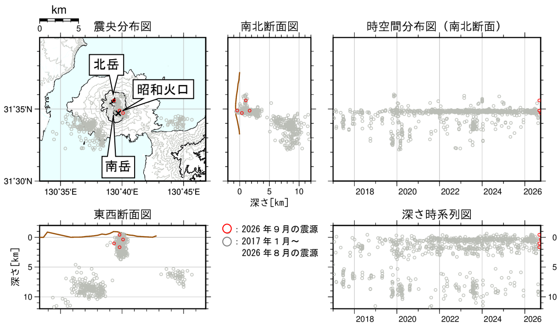
図 2-2 桜島 桜島付近の震源分布図（2017年1月～2026年9月）
