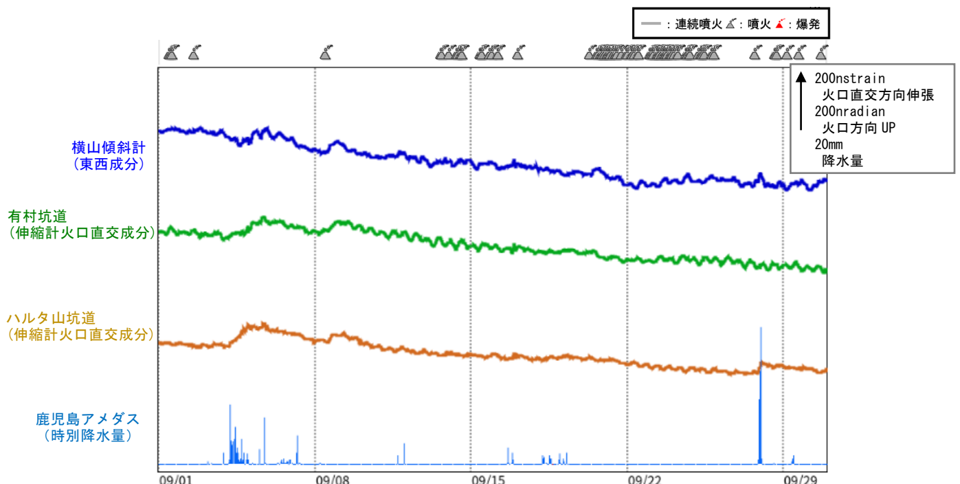
図 6 桜島 傾斜計及び伸縮計による地殻変動の状況（2026年9月1日～9月30日）
