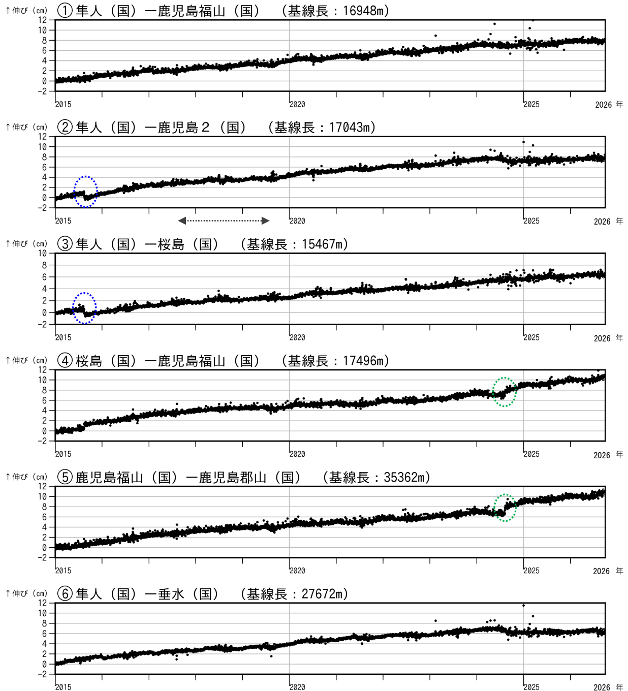
図 7-1 桜島 GNSS 連続観測による基線長変化 (2015 年 1 月～2026 年 9 月)
