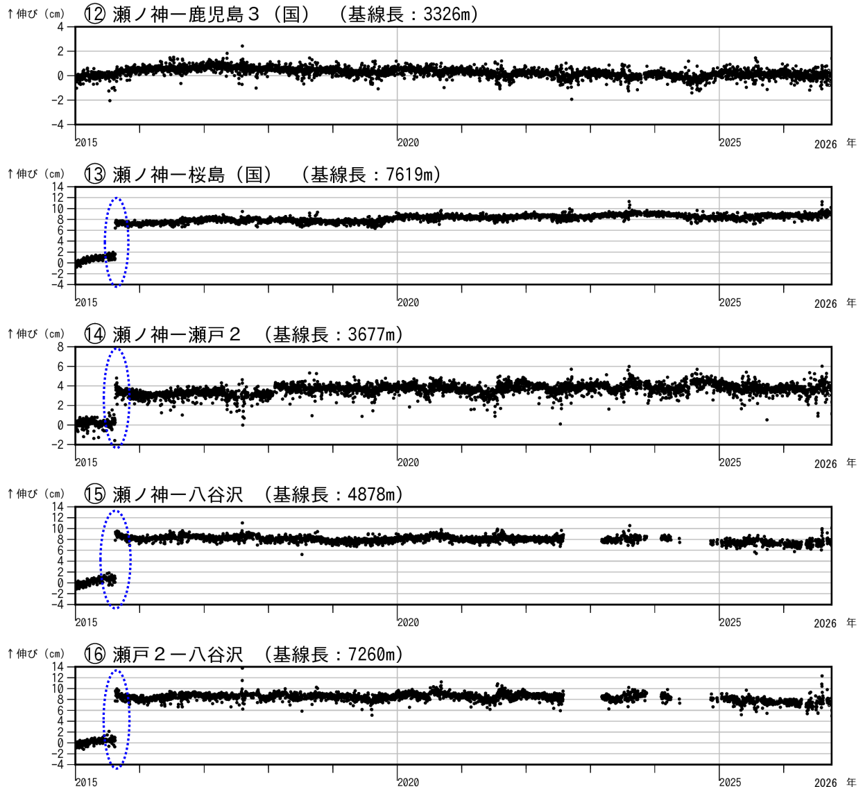
図 7-3 桜島 GNSS 連続観測による基線長変化（2015 年 1 月～2026 年 9 月）
