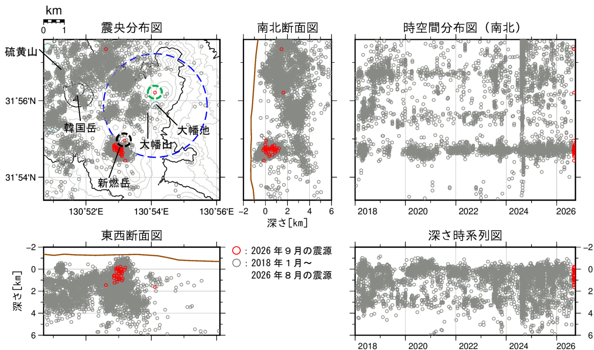
図3 霧島山（大幡池） 震源分布図（2018年1月～2026年9月）
