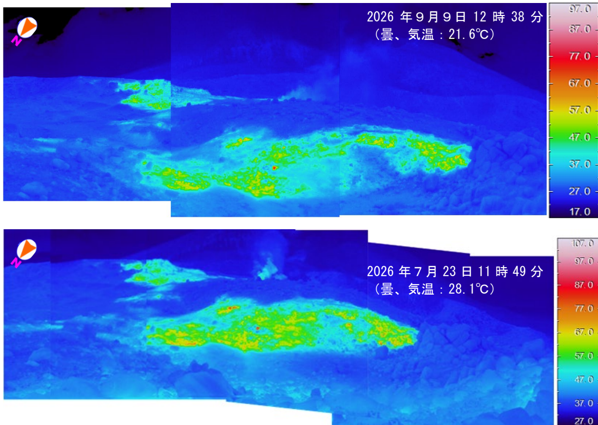
図 2-2 霧島山（えびの高原（硫黄山）周辺） 硫黄山火口内及び硫黄山南側の地熱域の状況
