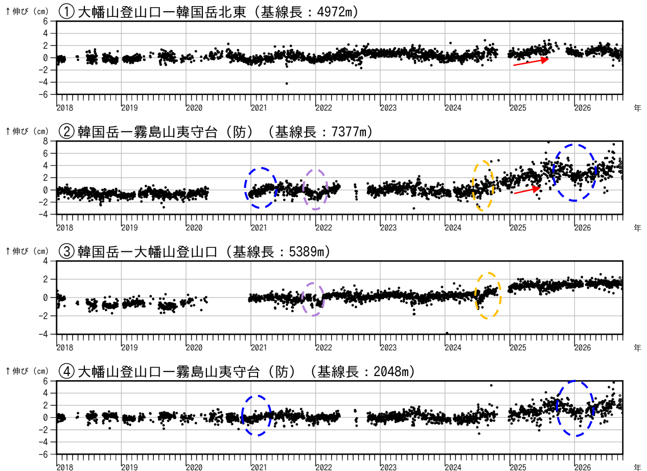
図4 霧島山（大幡池） GNSS 連続観測による基線長変化（2018年1月～2026年9月）
