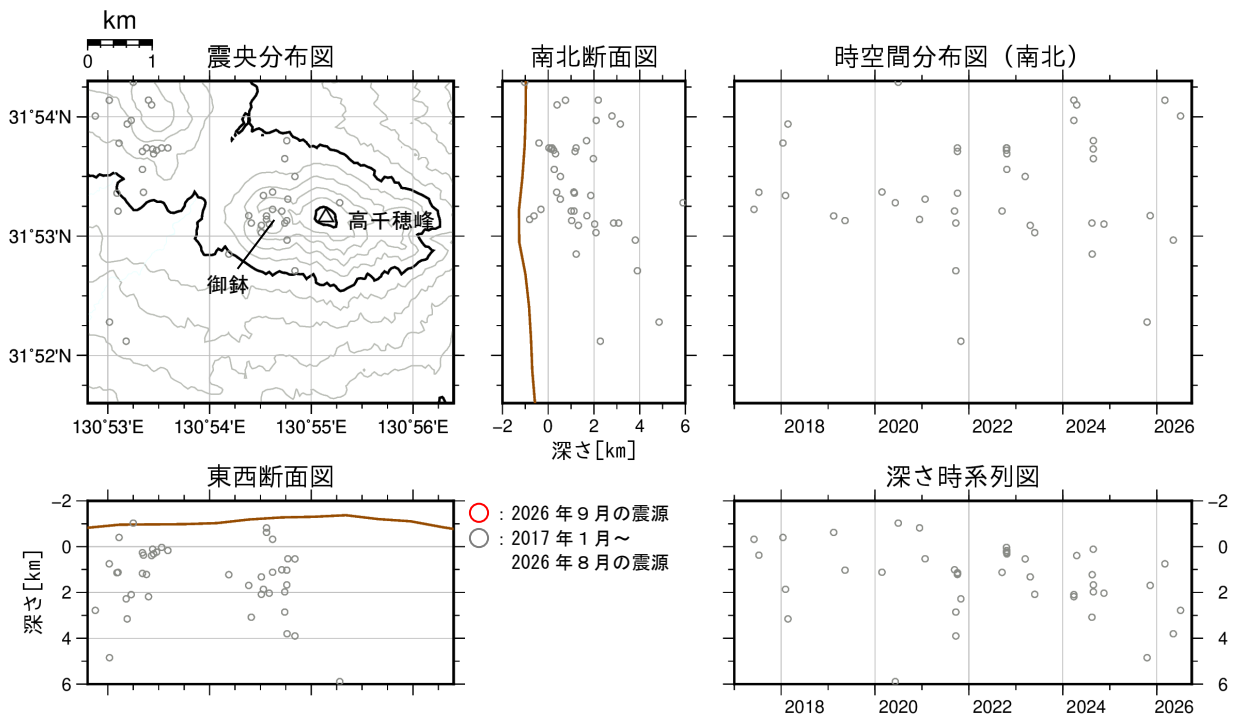
図2 霧島山（御鉢） 震源分布図（2017年1月～2026年9月）
