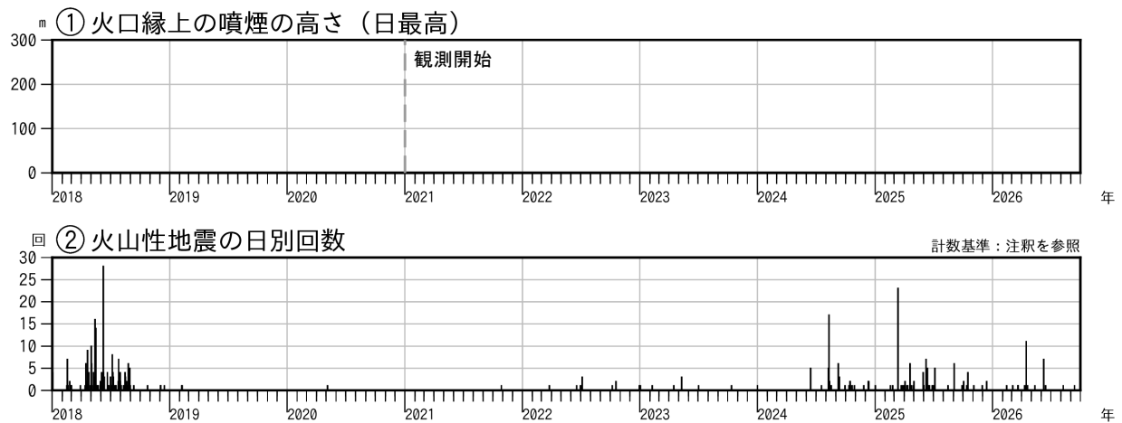
図2 霧島山（大幡池） 火山活動経過図（2018年1月～2026年9月）
