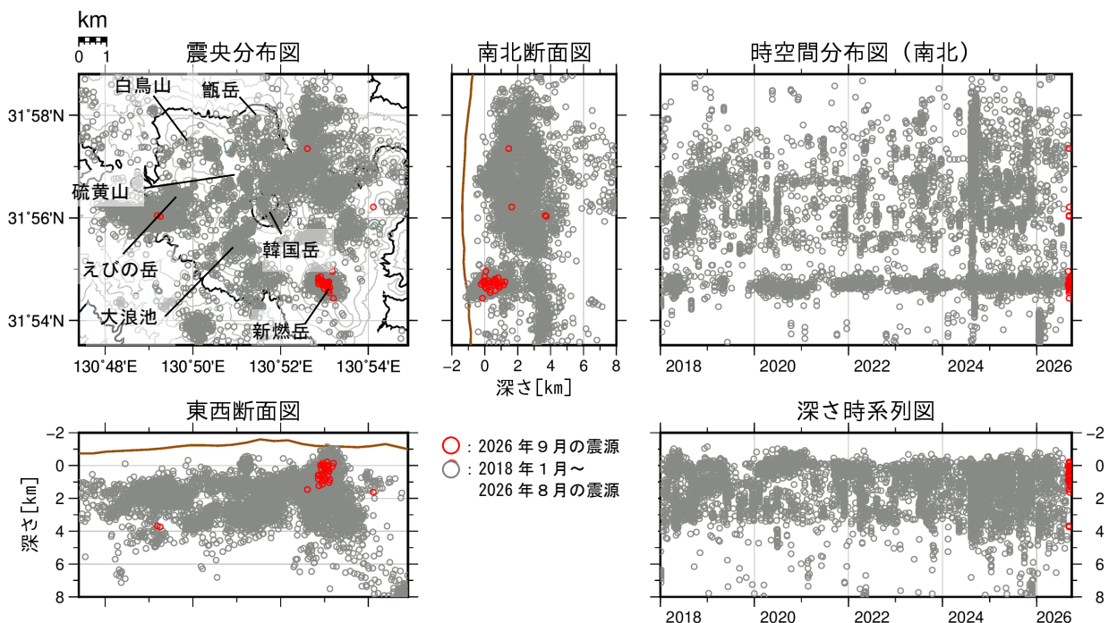
図4 霧島山（えびの高原（硫黄山）周辺）震源分布図（2018年1月～2026年9月）
