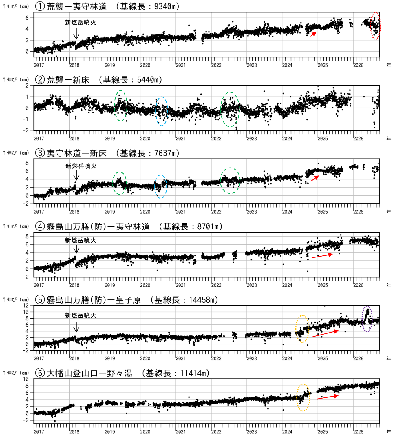
図6 霧島山（新燃岳） GNSS 連続観測による基線長変化（2017年1月～2026年9月）
