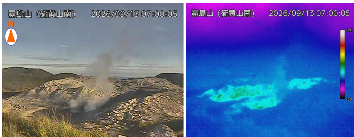
図 1-2 霧島山（えびの高原（硫黄山）周辺） 硫黄山南側の状況 （9 月 13 日、硫黄山南監視カメラ）
