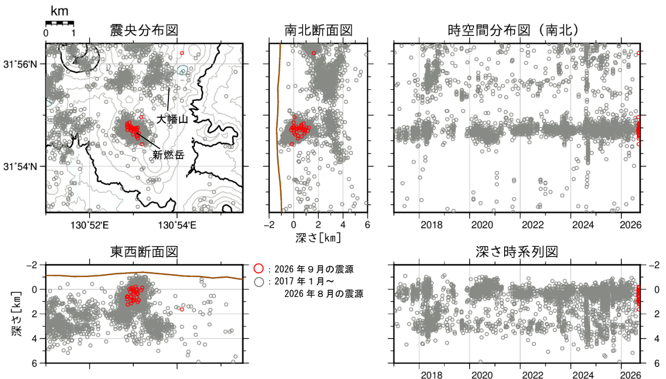
図 5 霧島山（新燃岳） 震源分布図（2017 年 1 月～2026 年 9 月）
