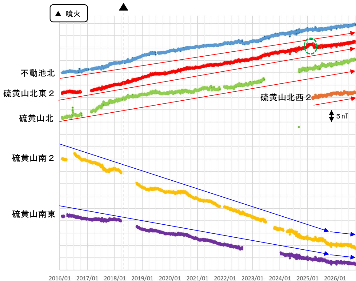
図 7-2 霧島山（えびの高原（硫黄山）周辺） 全磁力観測点で観測された全磁力変動
