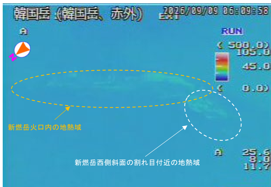
図1 霧島山（新燃岳） 噴煙及び地熱域の状況（9月9日、韓国岳監視カメラ）
