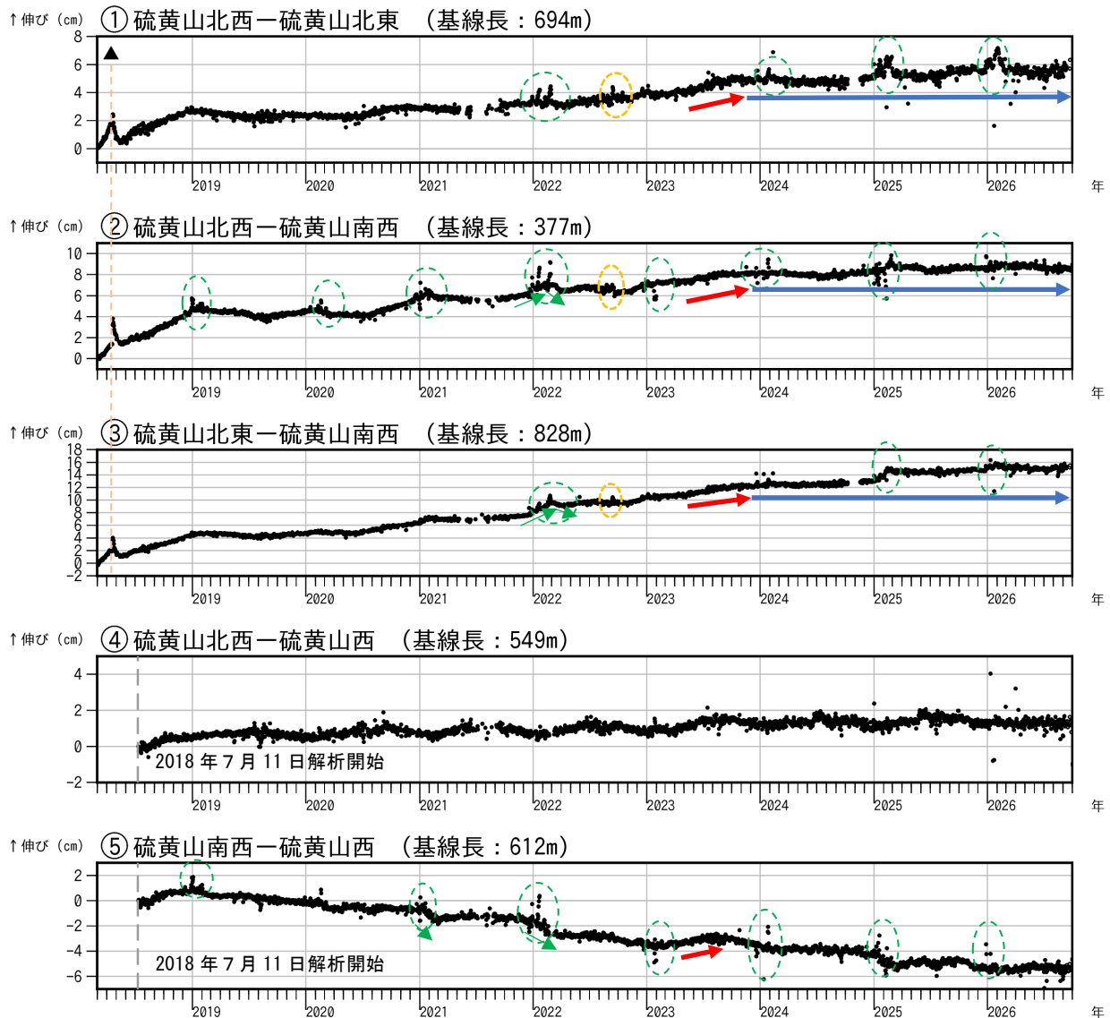
図5 霧島山（えびの高原（硫黄山）周辺） GNSS 連続観測による基線長変化（2018年3月～2026年9月）
