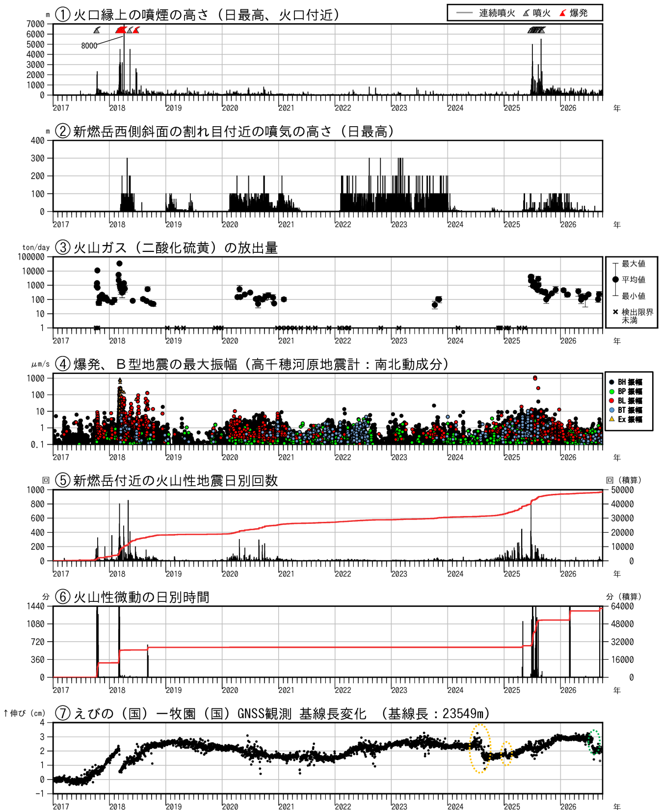
図 4-1 霧島山（新燃岳） 火山活動経過図（2017 年 1 月～2026 年 9 月）
