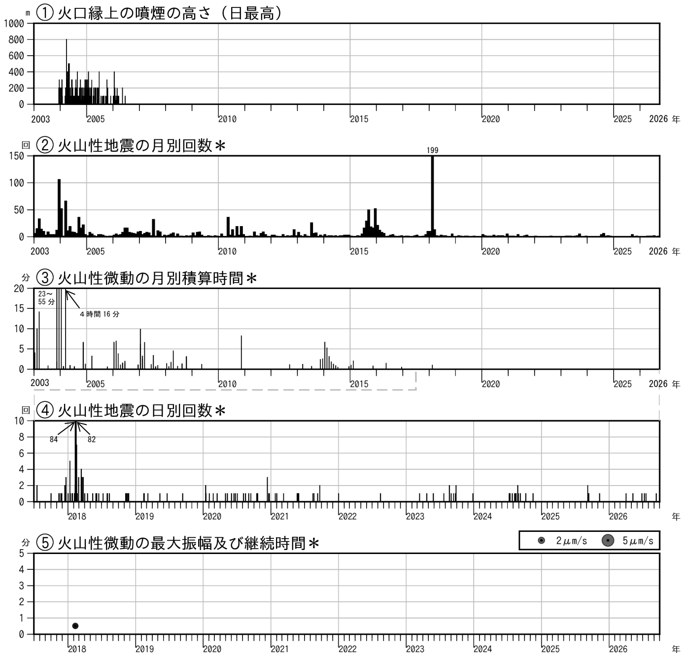
図3 霧島山（御鉢） 火山活動経過図（2003年1月～2026年9月）
