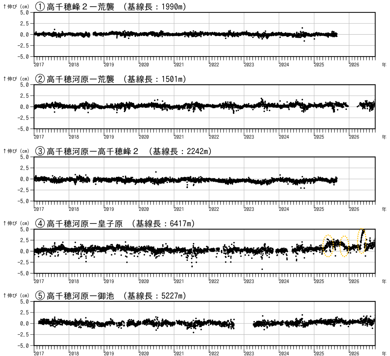
図4 霧島山（御鉢） GNSS 連続観測による基線長変化（2017年1月～2026年9月）
