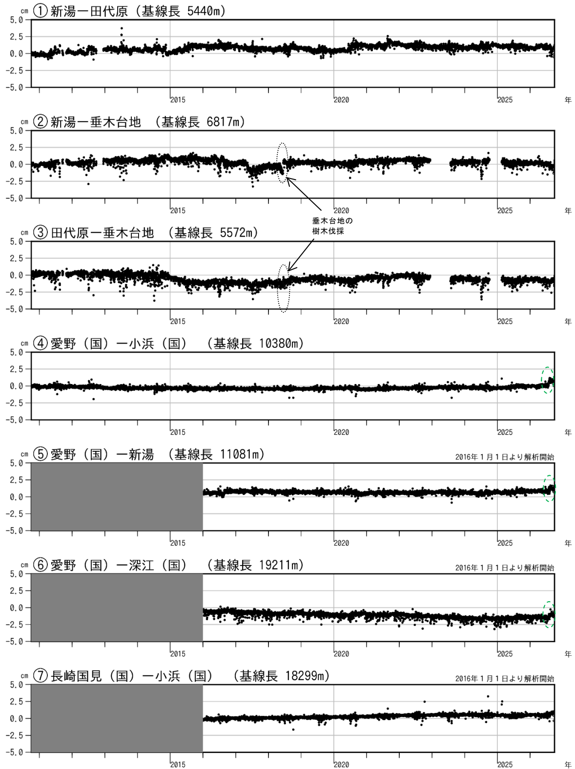
図5 雲仙岳 GNSS連続観測による基線長変化（2010年10月～2026年9月）
