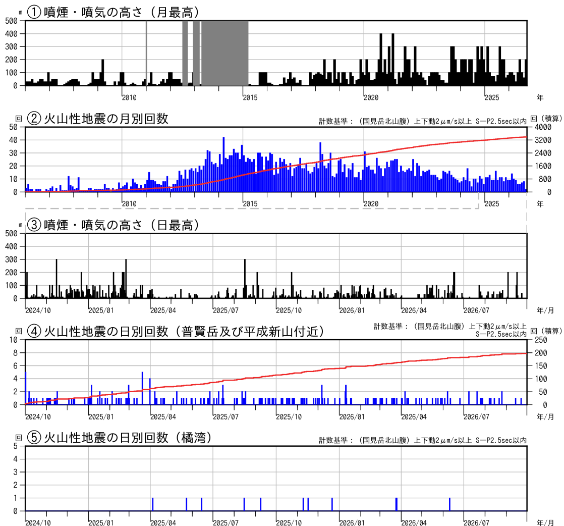
図3 雲仙岳 火山活動経過図（2006年1月～2026年9月）
