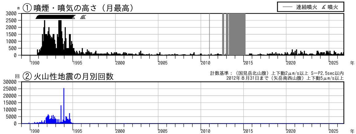
図2 雲仙岳 長期の火山活動経過図（1989年1月～2026年9月）
