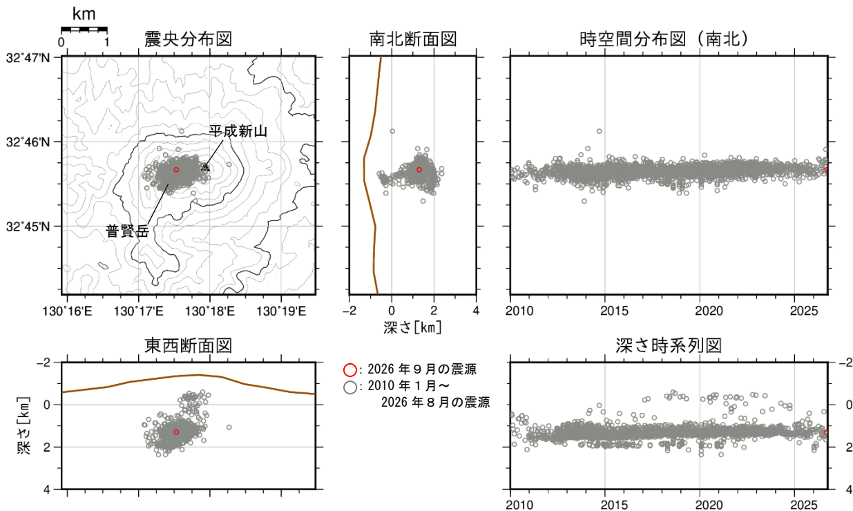
図4 雲仙岳 震源分布図 ①広域図 ②狭域図（2010年1月～2026年9月）
