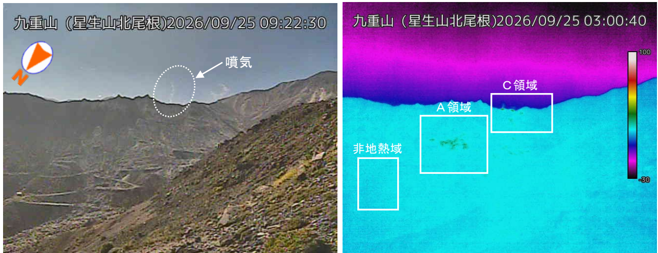
図 1-1 九重山 硫黄山の噴気及び地熱域の状況（9月25日、星生山北尾根監視カメラ）
