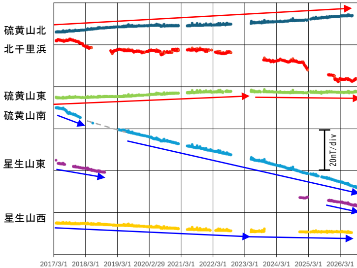
図 4-1 九重山 連続観測による全磁力の変化 (2017 年 3 月～2026 年 9 月)
