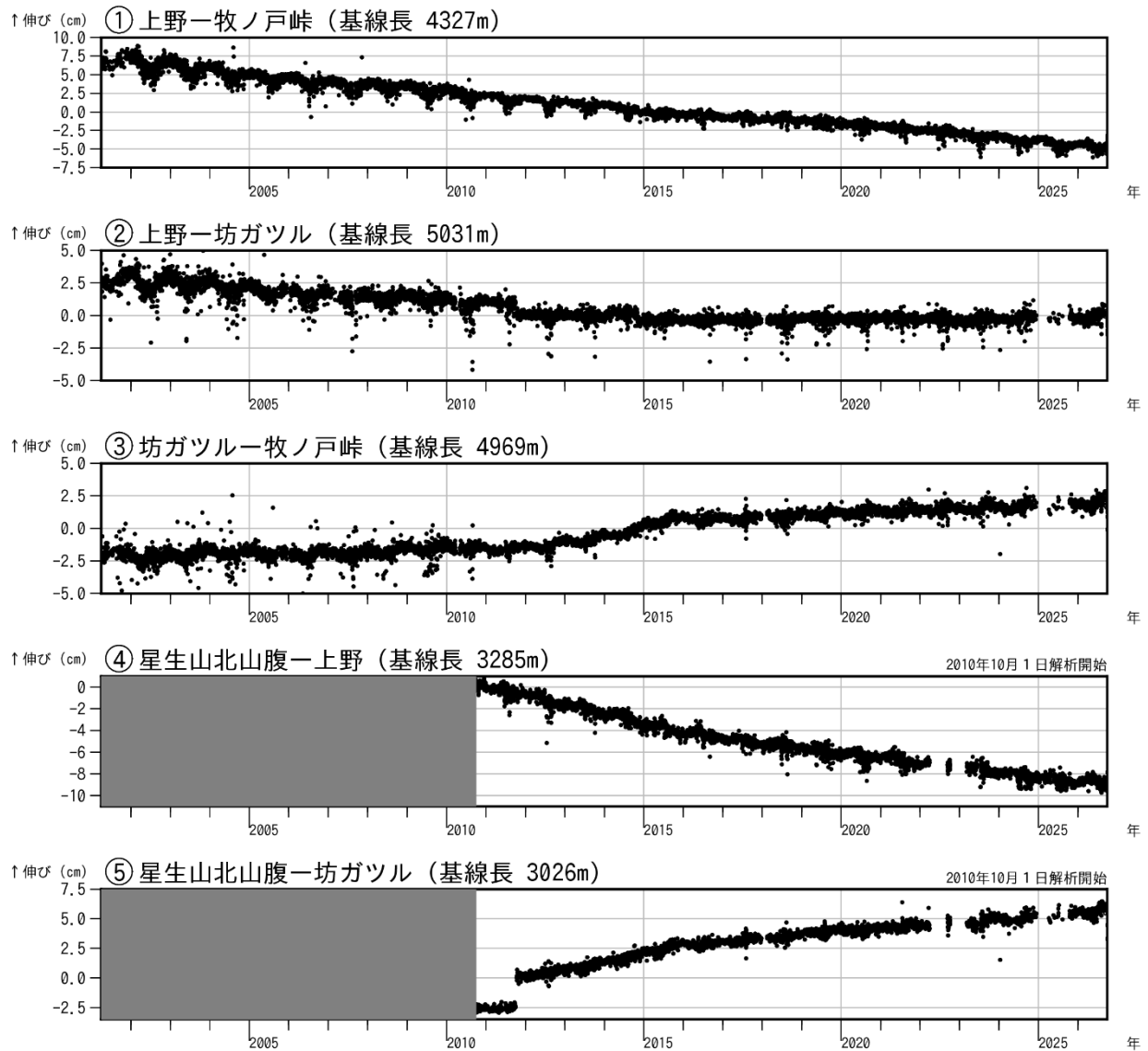
図 5-1 九重山 GNSS 連続観測による基線長変化（2001 年 4 月～2026 年 9 月）
