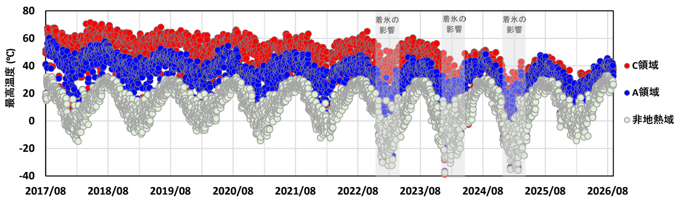
図 1-2 九重山 星生山北尾根の赤外熱映像装置による硫黄山の地熱域の日別最高温度（2017年8月～2026年9月）
