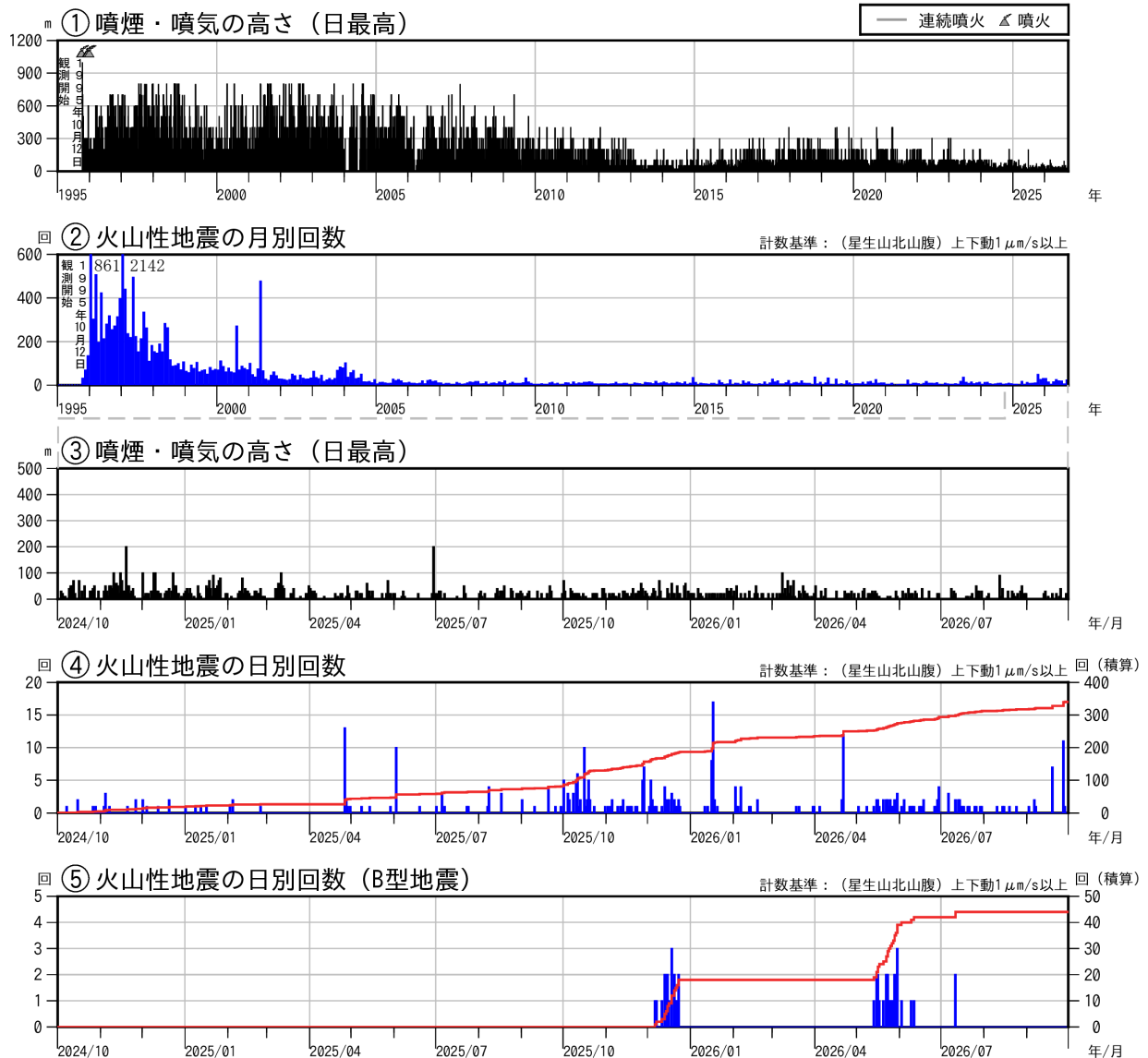
図2 九重山 火山活動経過図（1995年1月～2026年9月）
