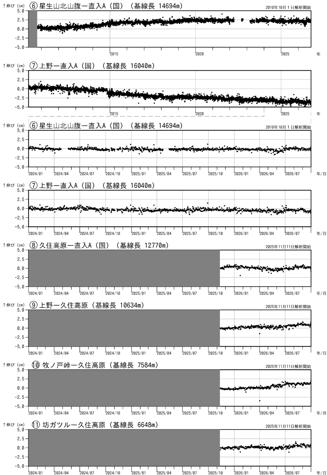
図 5-2 九重山 GNSS 連続観測による基線長変化（2010 年 1 月～2026 年 9 月）
