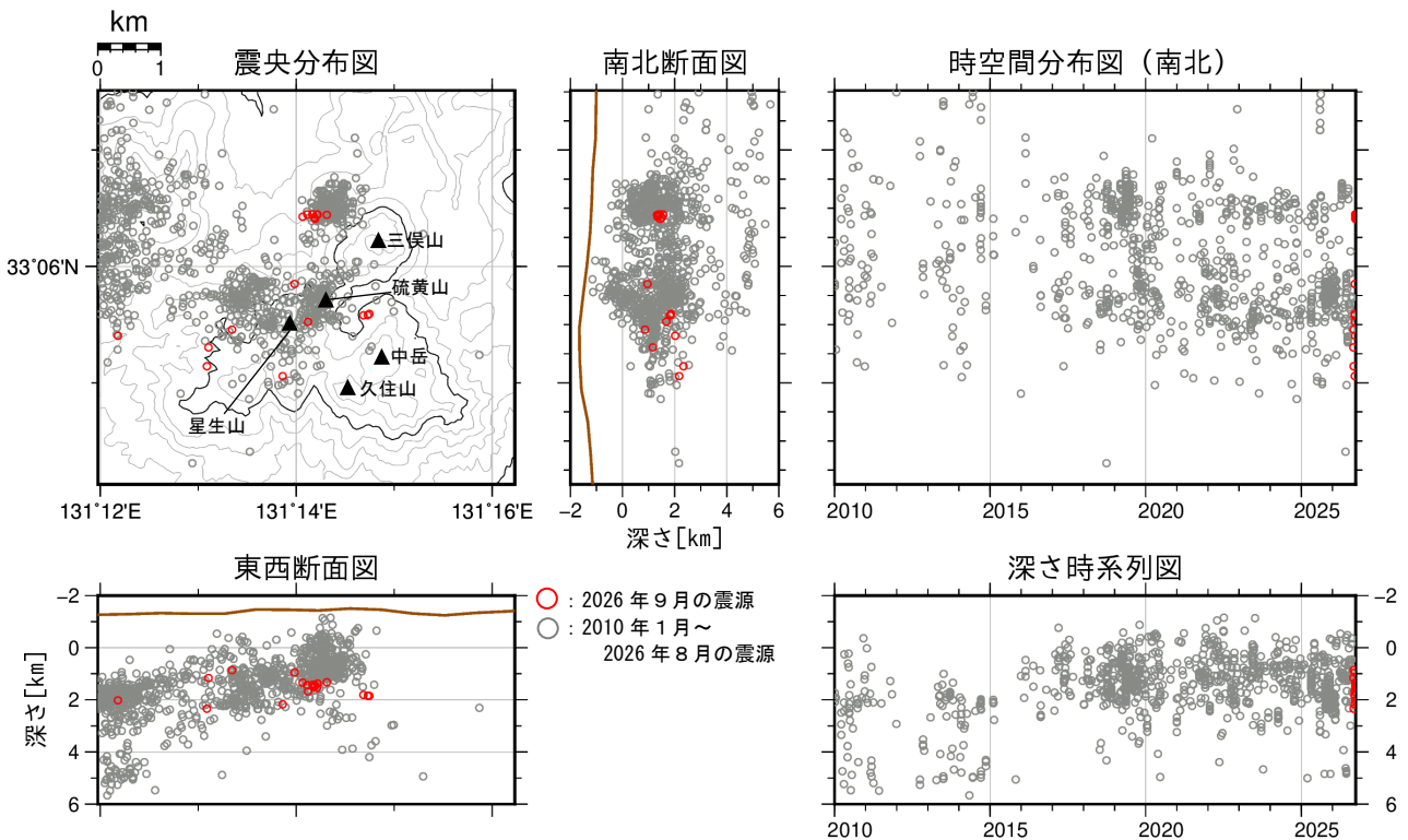
図3 九重山 震源分布図 ①広域図 ②狭域図（2010年1月～2026年9月）
