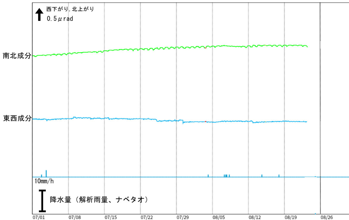
図5 諏訪之瀬島 ナベタオ観測点の傾斜変動（2026年7月～8月）
