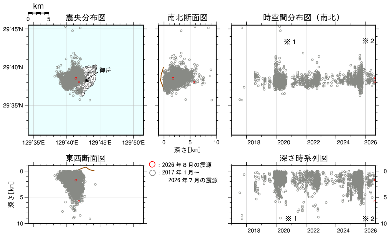
図4 諏訪之瀬島 震源分布図（2017年1月～2026年8月）
