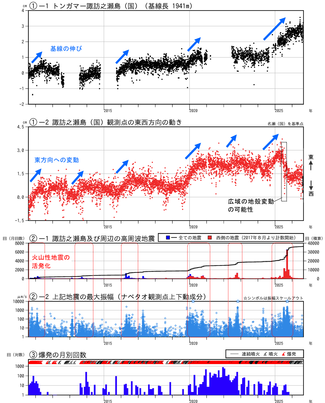
図 6-2 諏訪之瀬島 GNSS連続観測と周辺の火山性地震（2010年8月～2026年8月）
