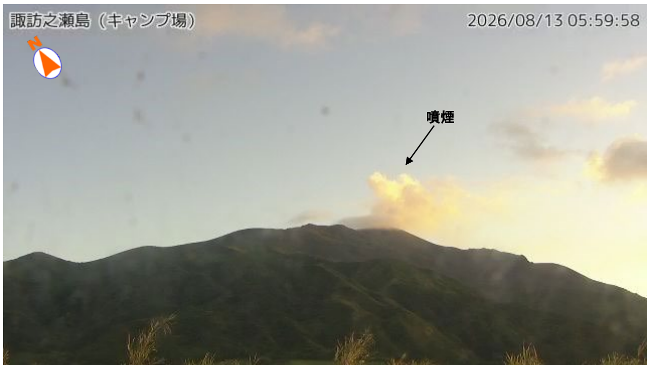
図1 諏訪之瀬島 噴火活動の状況（8月13日 キャンプ場監視カメラ）
