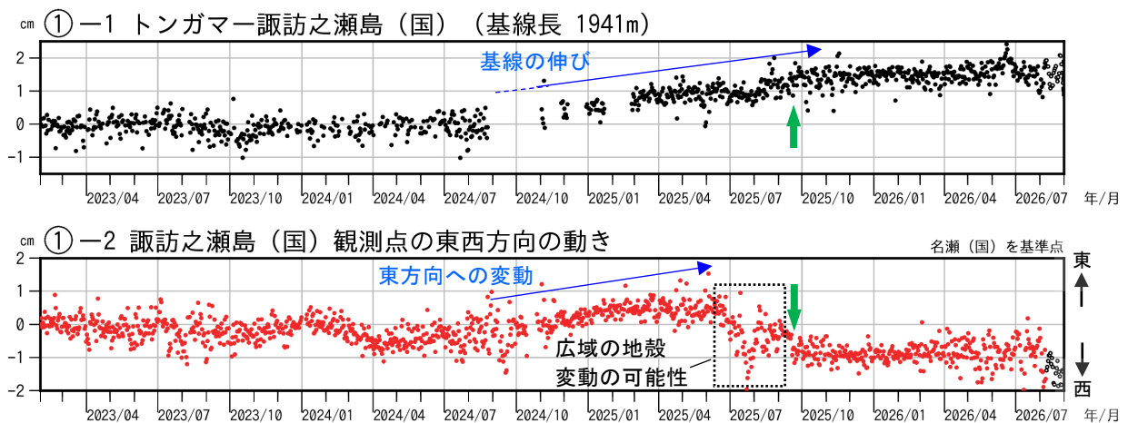
図6-1 諏訪之瀬島 GNSS連続観測（2023年2月～2026年8月）
