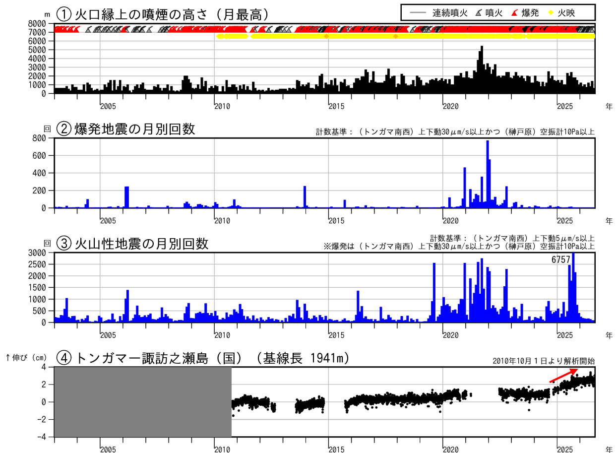
図2 諏訪之瀬島 長期の火山活動経過図（2003年1月～2026年8月）
