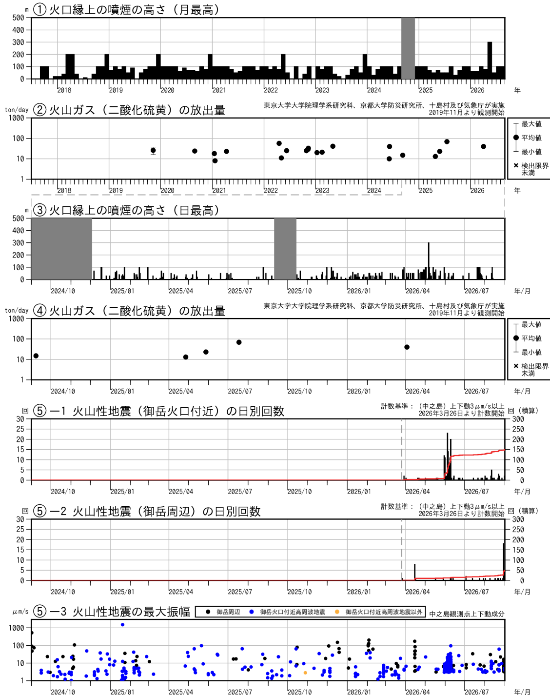
図2 中之島 火山活動経過図（2017年7月～2026年8月）
