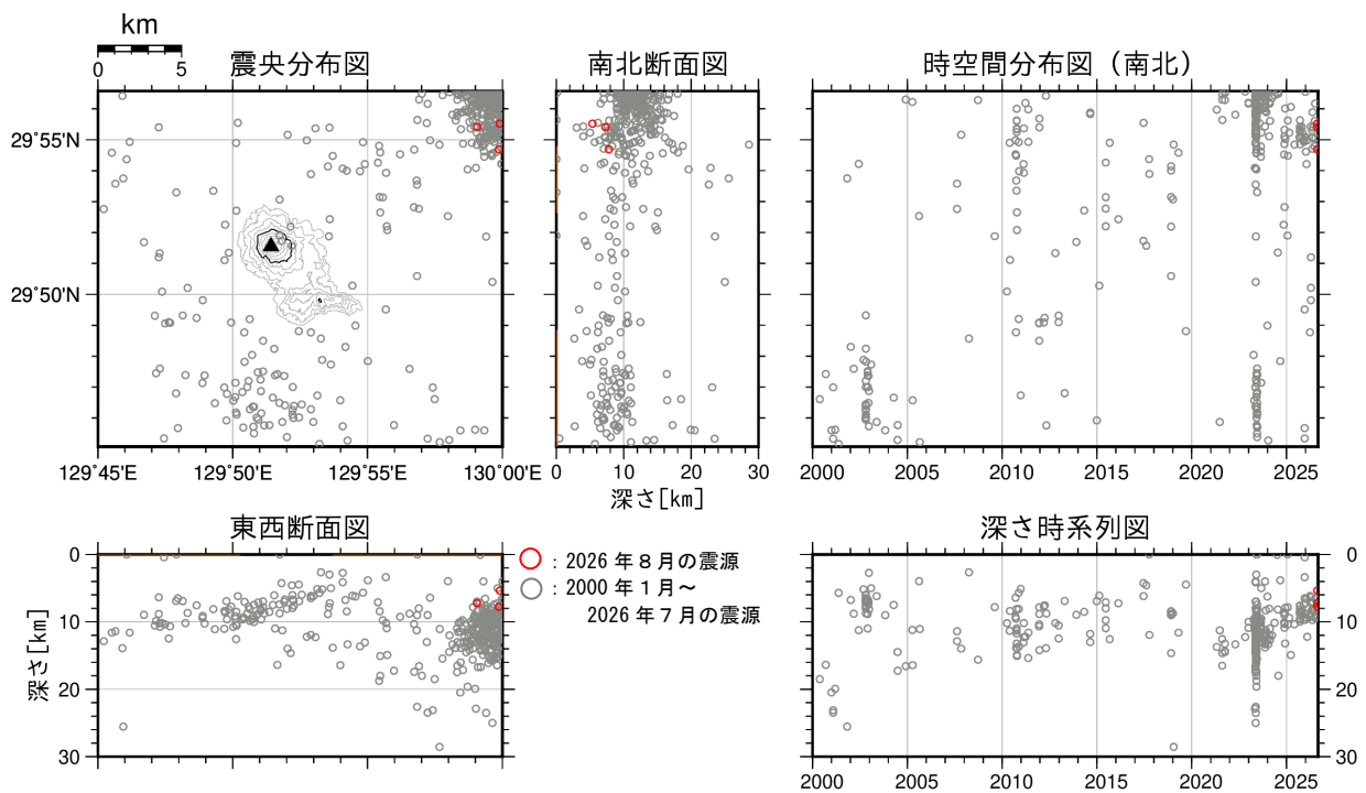
図3 中之島 中之島周辺の震源分布図（2000年1月～2026年8月）
