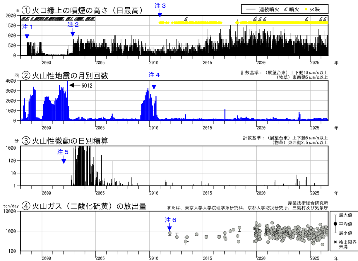
図2 薩摩硫黄島 火山活動経過図（1998年1月～2026年8月）
