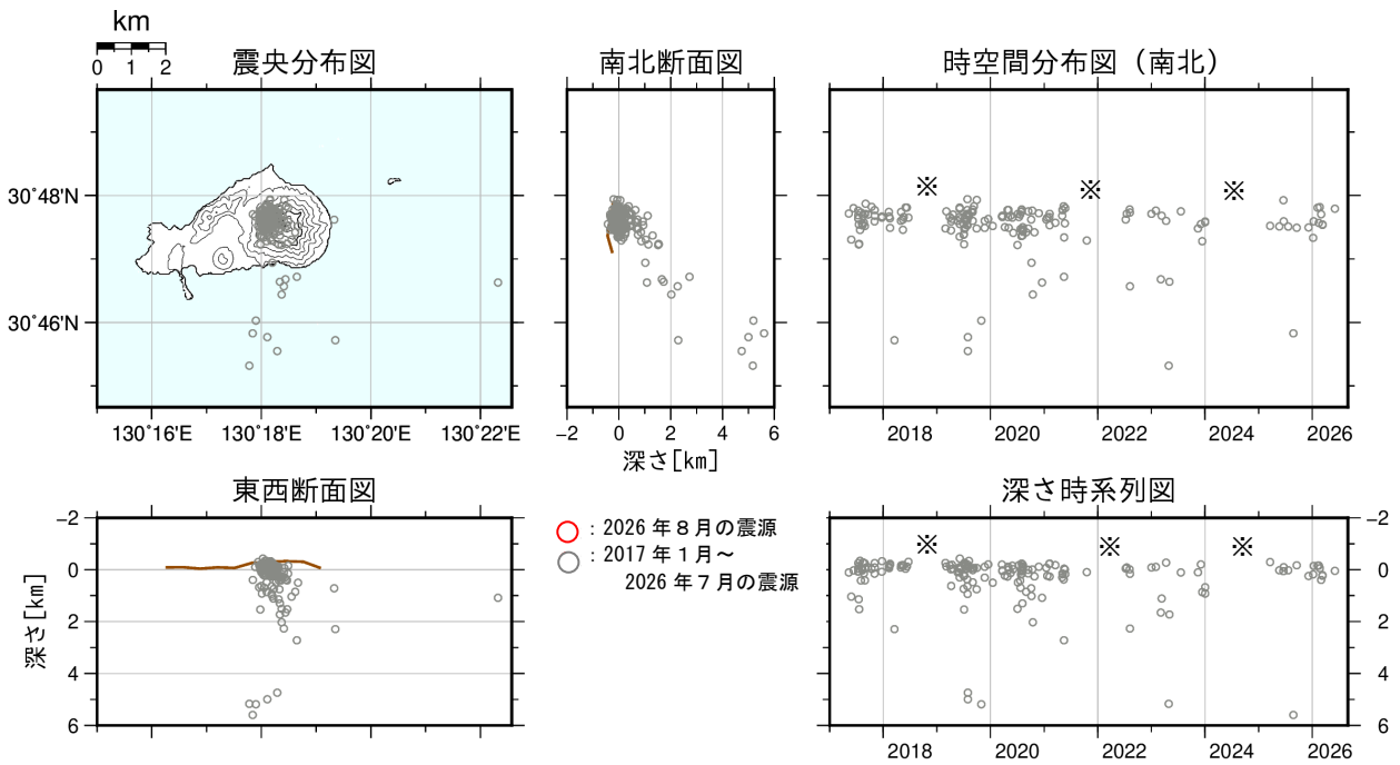
図4 薩摩硫黄島 火山性地震の震源分布図（2017年1月～2026年8月）
