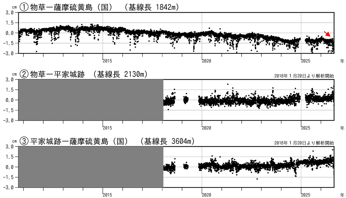
図5 薩摩硫黄島 GNSS連続観測による基線長変化（2010年10月～2026年8月）
