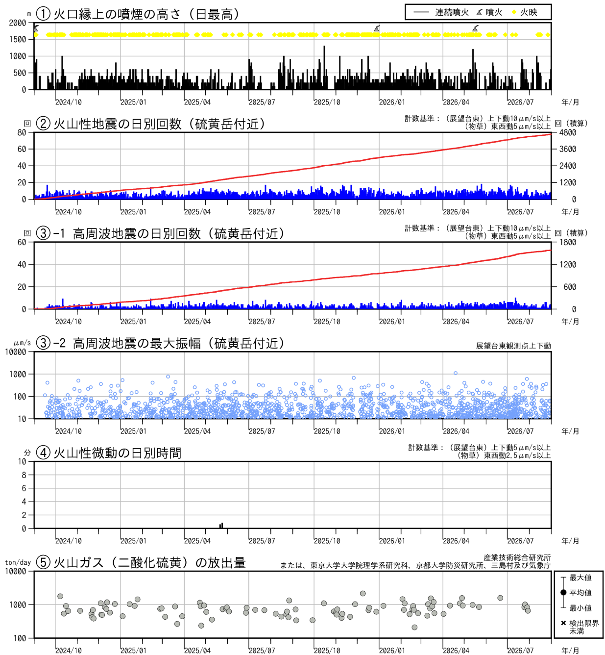
図3 薩摩硫黄島 火山活動経過図（2024年9月～2026年8月）
