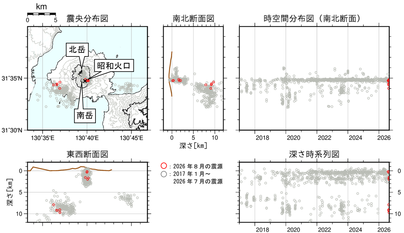
図 2-2 桜島 桜島付近の震源分布図（2017年1月～2026年8月）
