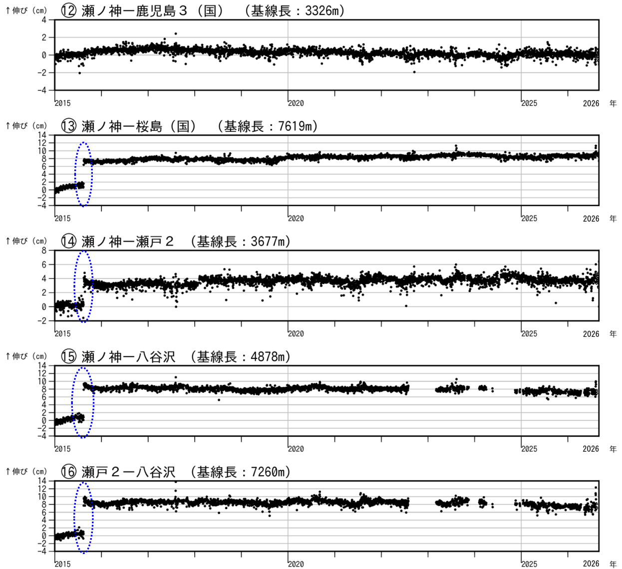
図 7-3 桜島 GNSS 連続観測による基線長変化（2015 年 1 月～2026 年 8 月）
