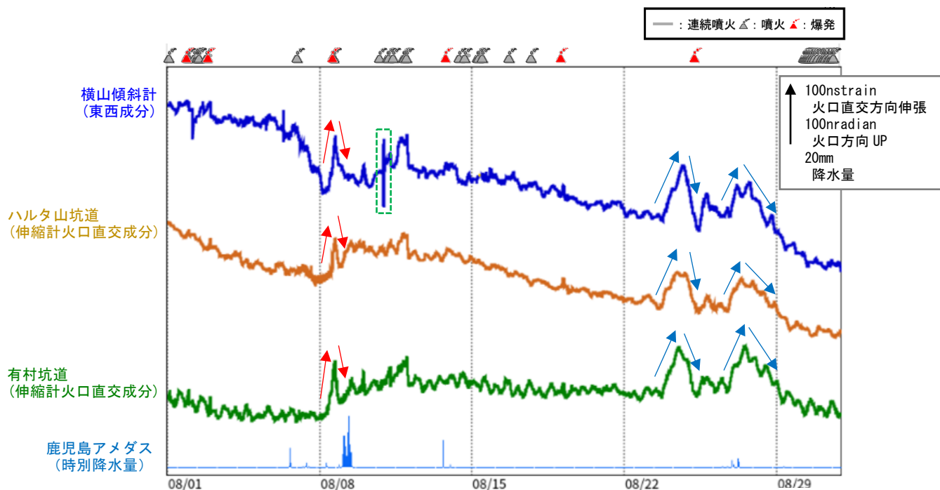
図 6 桜島 傾斜計及び伸縮計による地殻変動の状況（2026年8月1日～8月31日）
