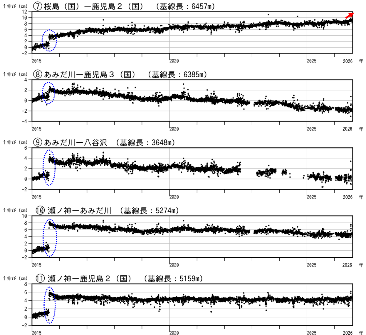
図 7-2 桜島 GNSS 連続観測による基線長変化（2015 年 1 月～2026 年 8 月）
