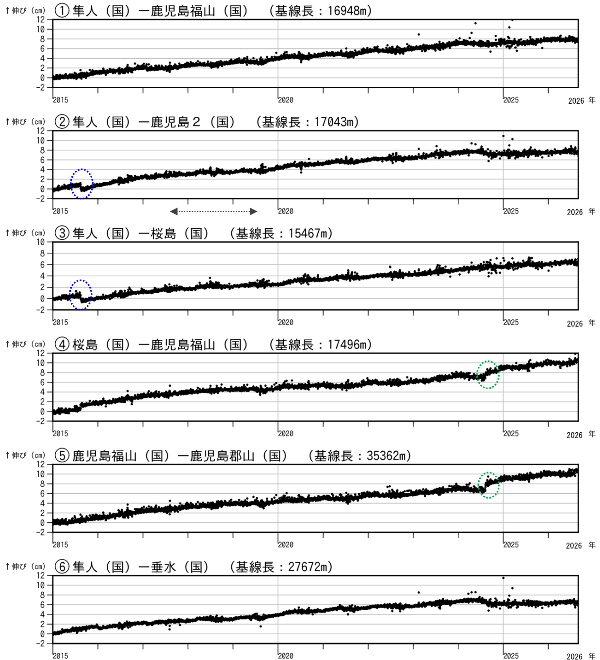
図 7-1 桜島 GNSS 連続観測による基線長変化 (2015 年 1 月～2026 年 8 月)
