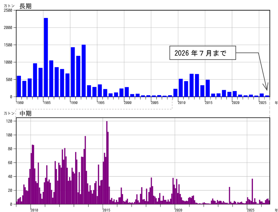
図4 桜島 鹿児島県が実施している降灰の観測データから推定した火山灰の総噴出量 （上段：1980年1月～2026年7月までの年別値、下段：2009年1月～2026年7月の月別値）
