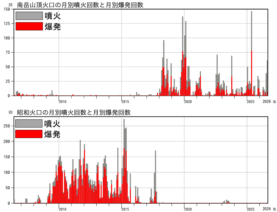
図3 桜島 南岳山頂火口（上図）と昭和火口（下図）の月別噴火回数と月別爆発回数 （2006年6月～2026年8月）
