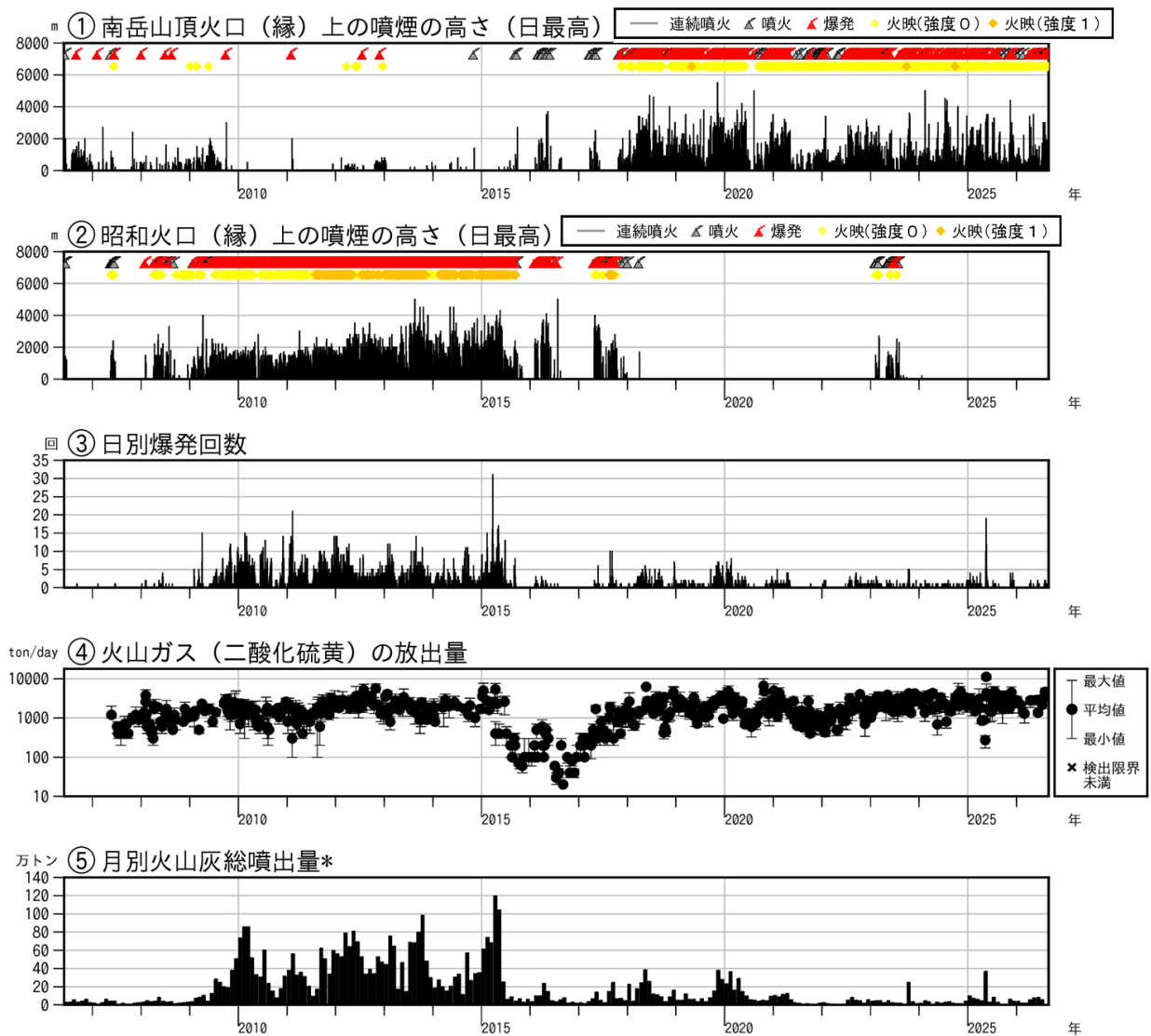
図 5-1 桜島 昭和火口噴火活動再開（2006 年 6 月）以降の活動経過図（2006 年 6 月～2026 年 8 月）
