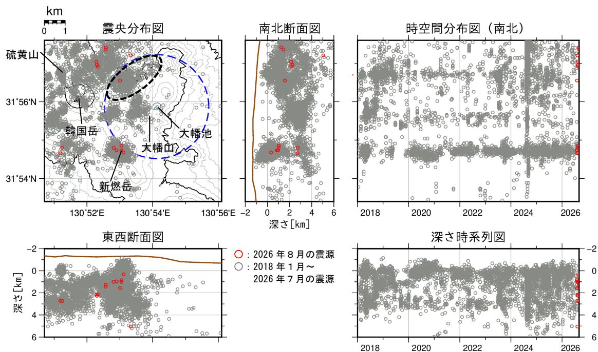
図3 霧島山（大幡池） 震源分布図（2018年1月～2026年8月）
