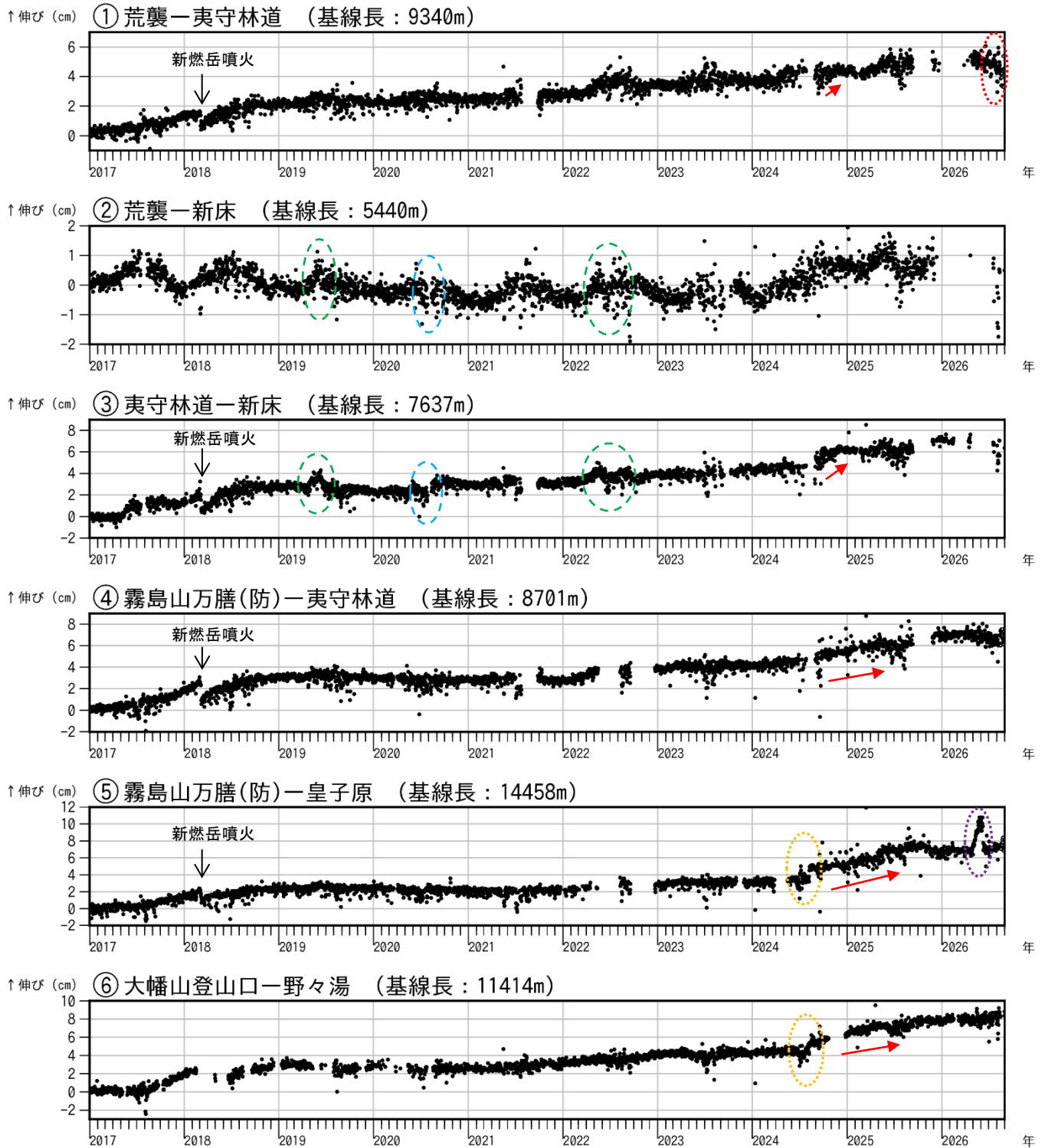
図4 霧島山（新燃岳） GNSS 連続観測による基線長変化（2017年1月～2026年8月）
