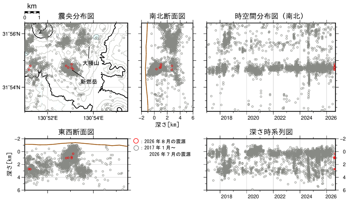
図 3 霧島山（新燃岳） 震源分布図（2017 年 1 月～2026 年 8 月）
