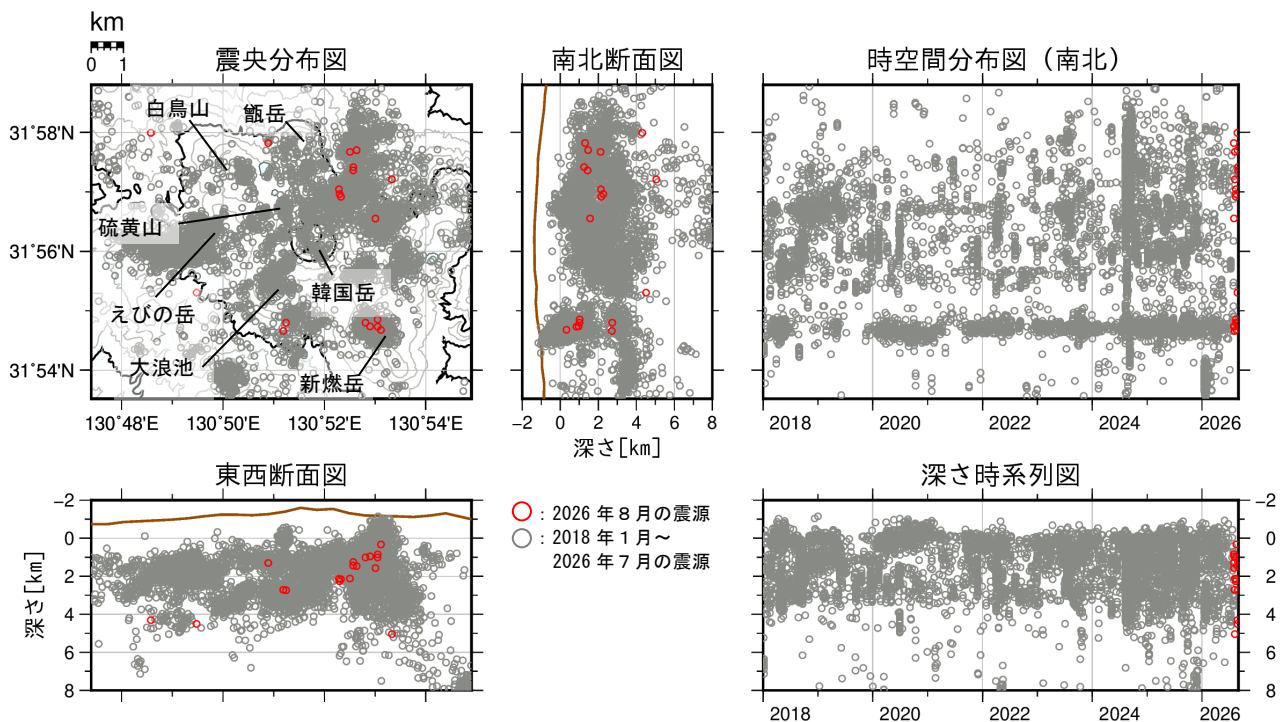
図3 霧島山（えびの高原（硫黄山）周辺） 震源分布図（2018年1月～2026年8月）
