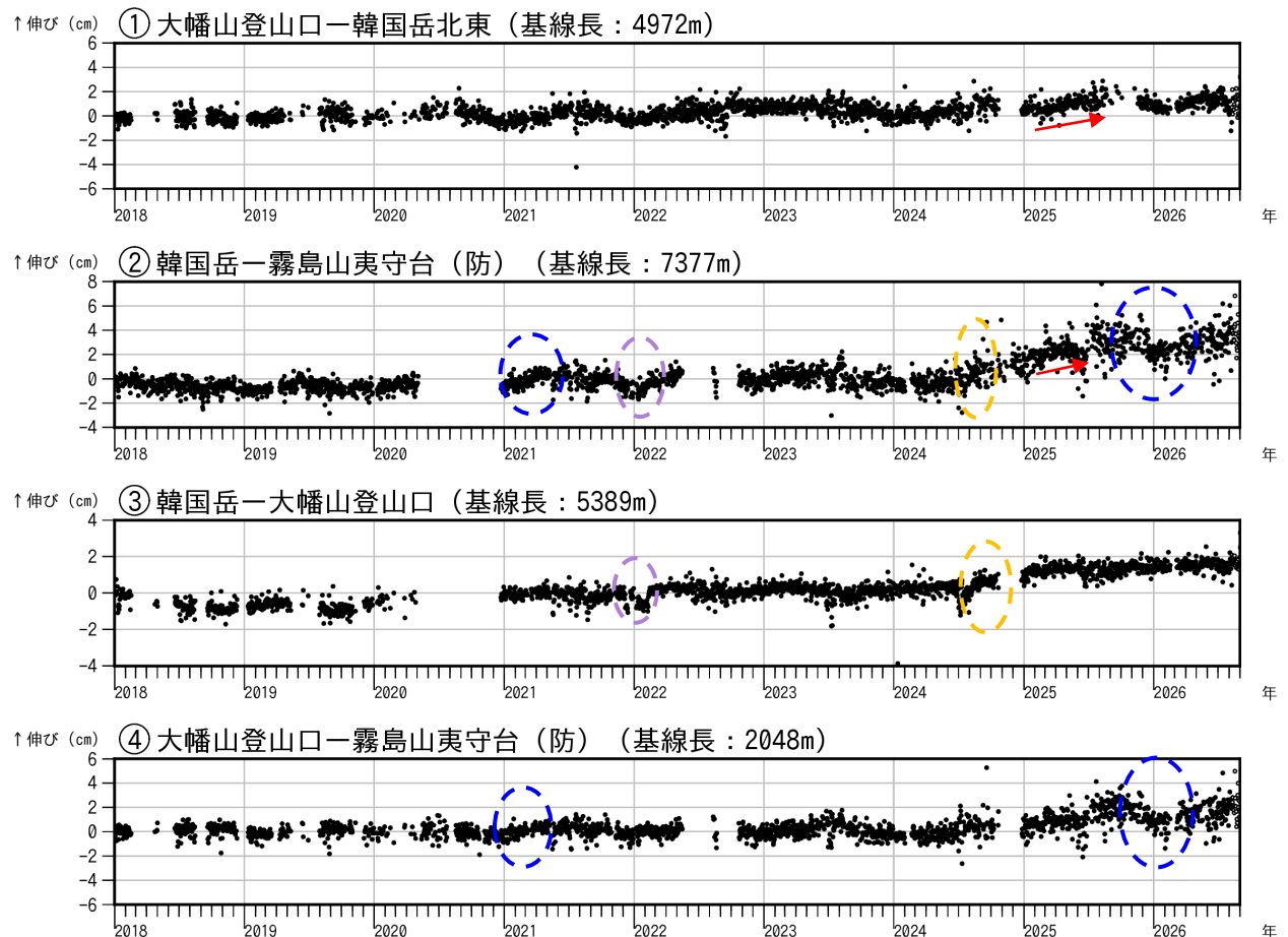
図4 霧島山（大幡池） GNSS 連続観測による基線長変化（2018年1月～2026年8月）
