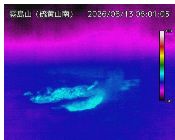
図1-2 霧島山（えびの高原（硫黄山）周辺） 硫黄山南側の状況 （8月13日、硫黄山南監視カメラ）
