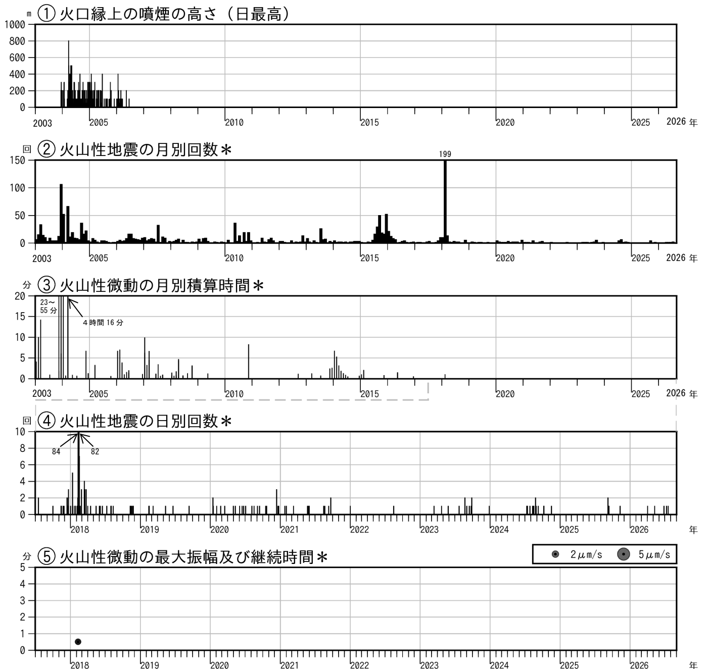
図3 霧島山（御鉢） 火山活動経過図（2003年1月～2026年8月）
