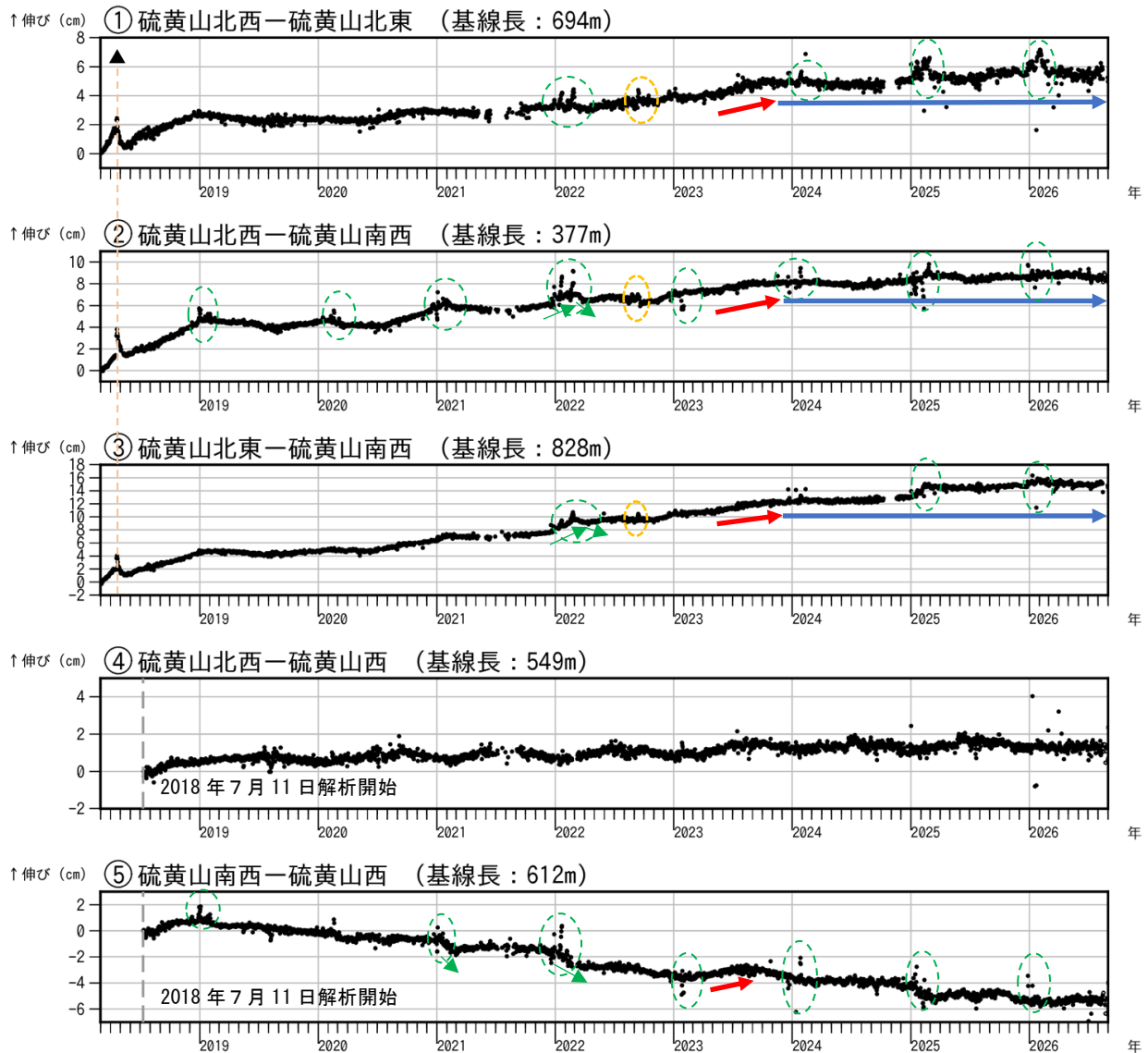
図4 霧島山（えびの高原（硫黄山）周辺） GNSS 連続観測による基線長変化（2018年3月～2026年8月）
