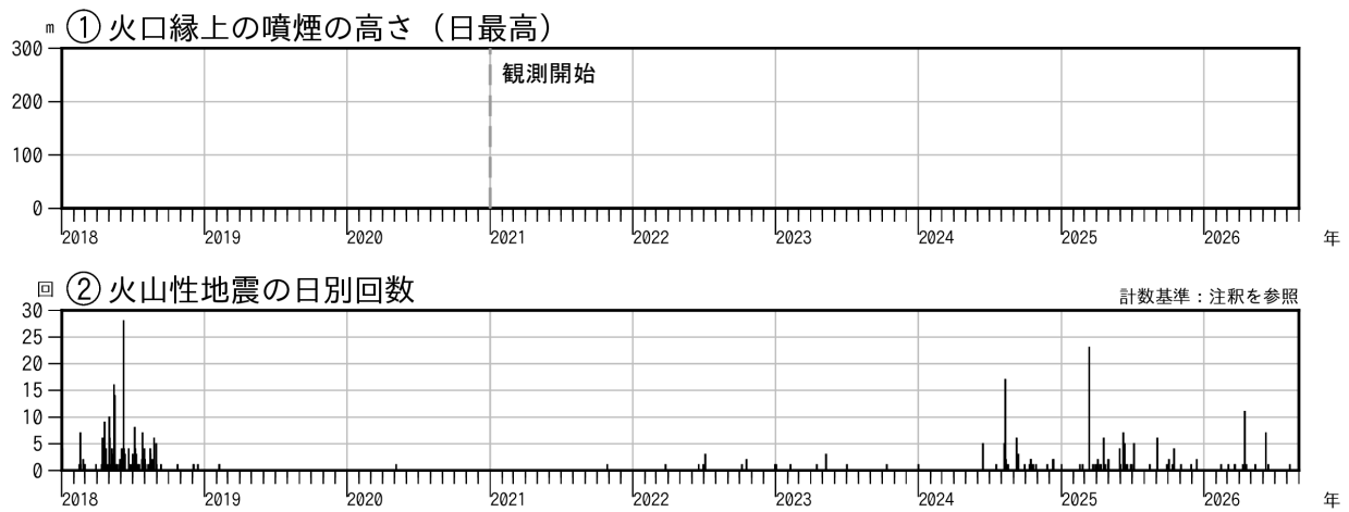
図2 霧島山（大幡池） 火山活動経過図（2018年1月～2026年8月）
