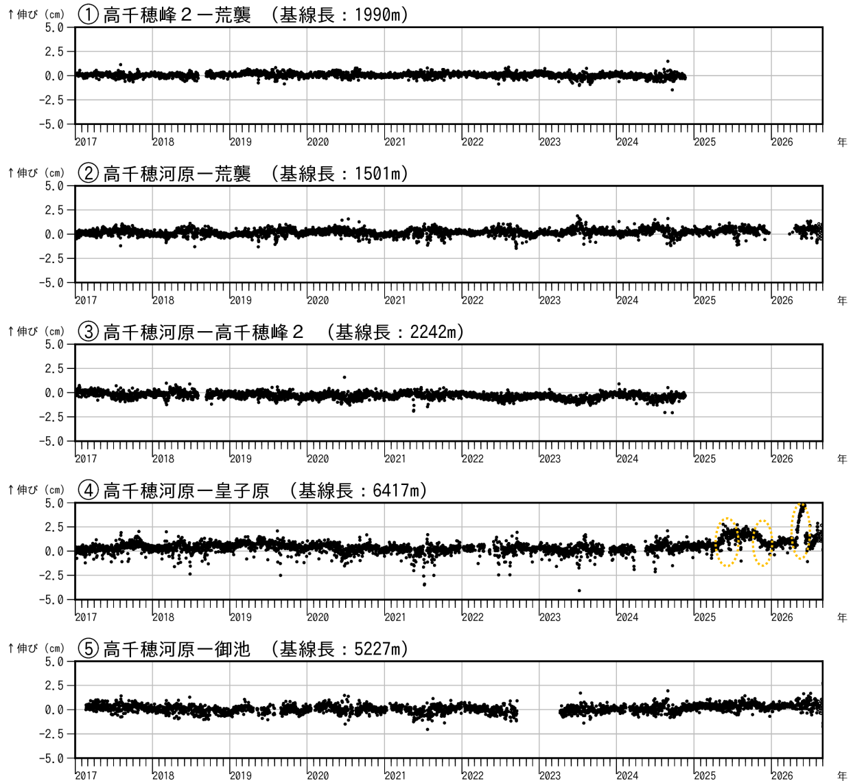
図4 霧島山（御鉢） GNSS 連続観測による基線長変化（2017年1月～2026年8月）
