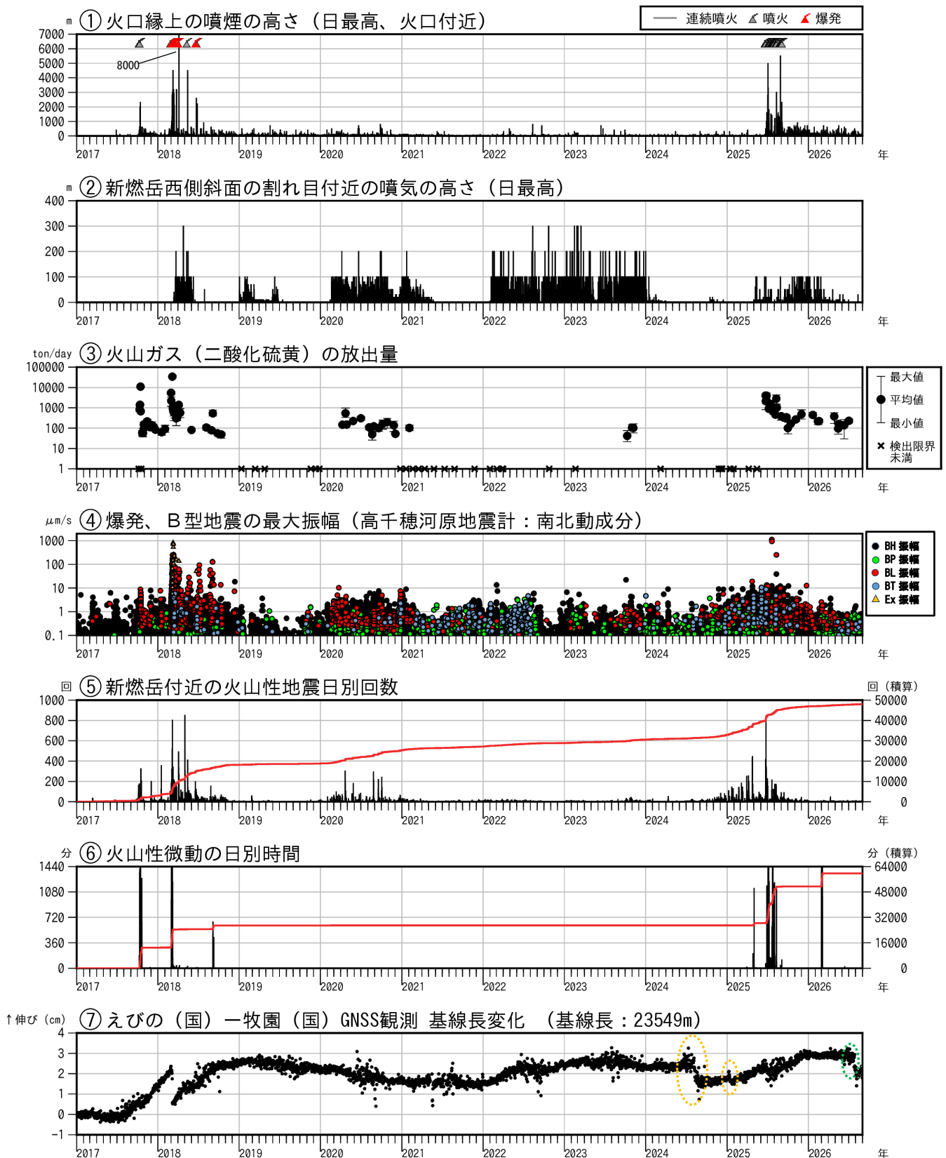
図 2-1 霧島山（新燃岳） 火山活動経過図（2017 年 1 月～2026 年 8 月）
