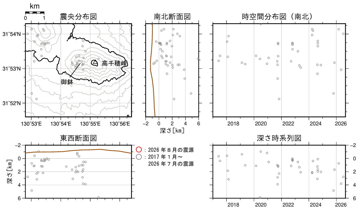
図2 霧島山（御鉢） 震源分布図（2017年1月～2026年8月）
