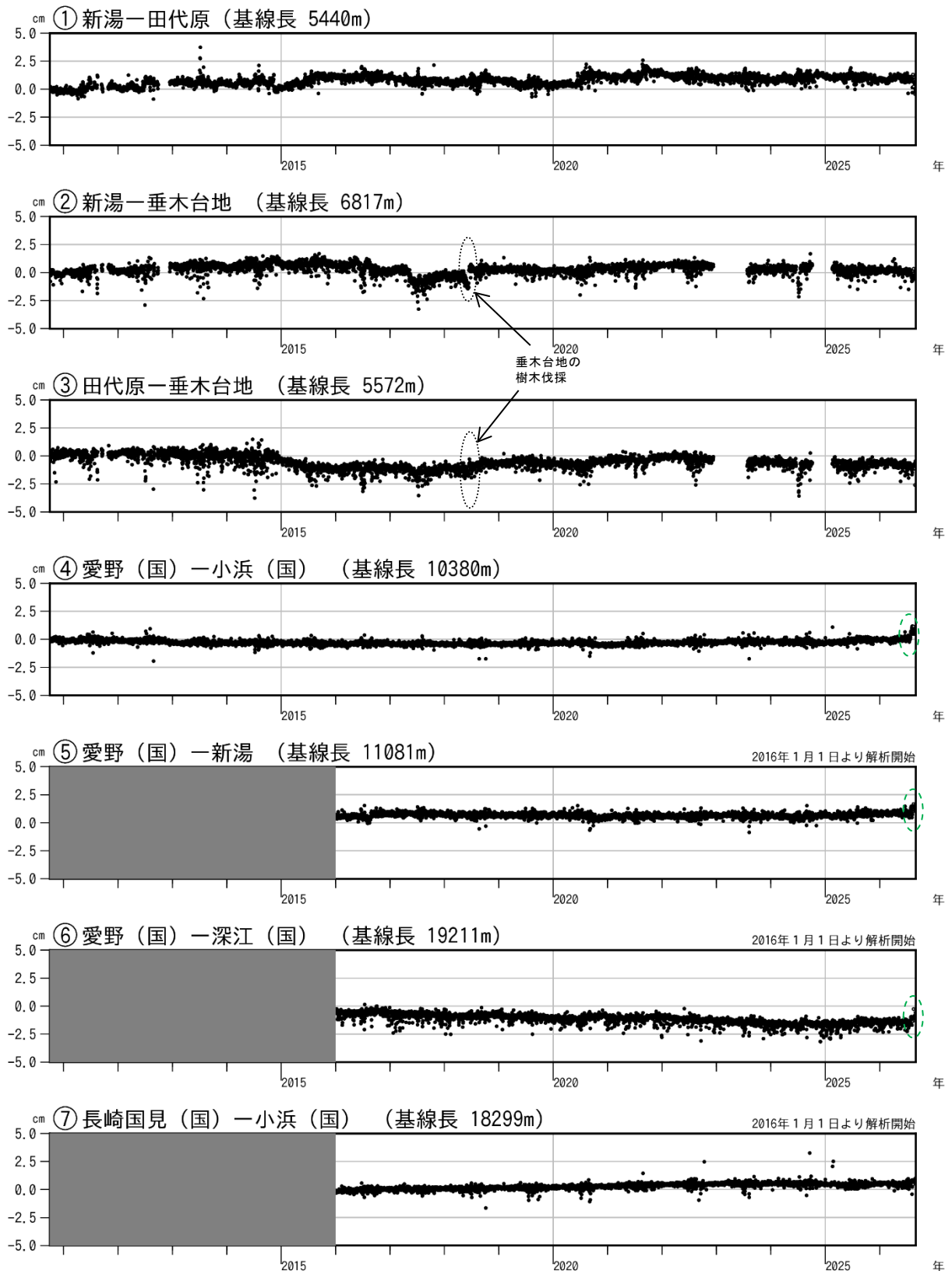
図 5 雲仙岳 GNSS連続観測による基線長変化（2010 年 10 月～2026 年 8 月）
