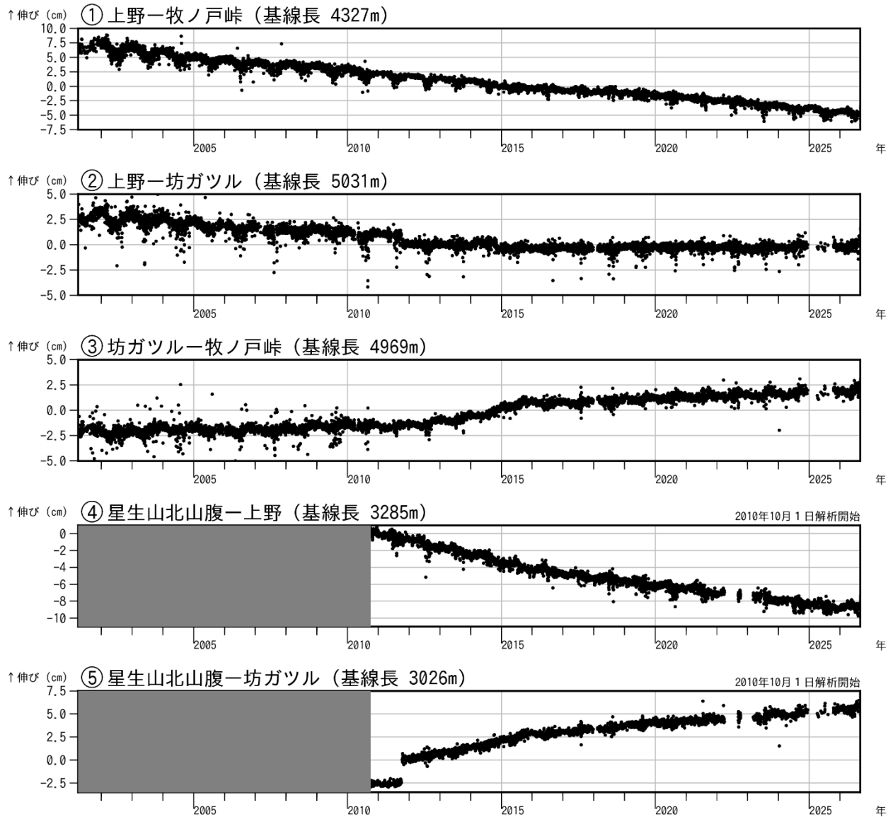
図 5-1 九重山 GNSS 連続観測による基線長変化（2001 年 4 月～2026 年 8 月）
