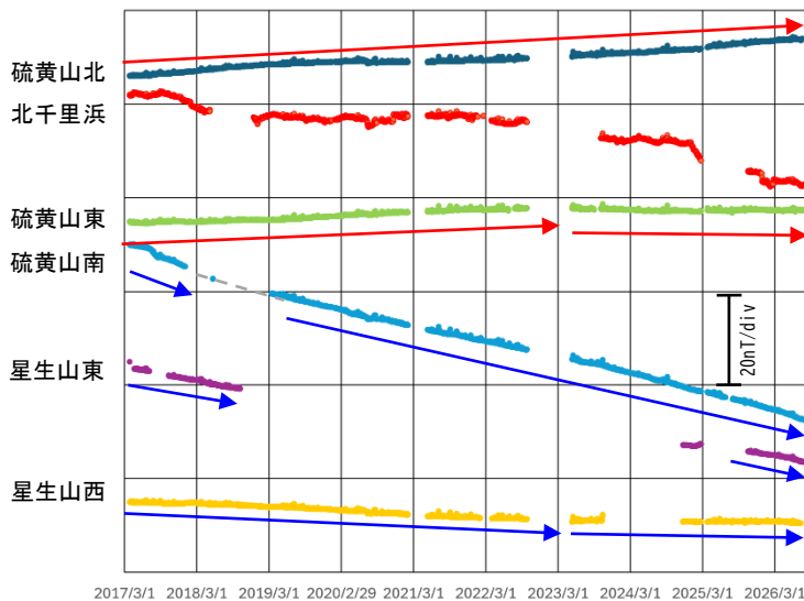
図 4-1 九重山 連続観測による全磁力の変化 (2017 年 3 月～2026 年 8 月)
