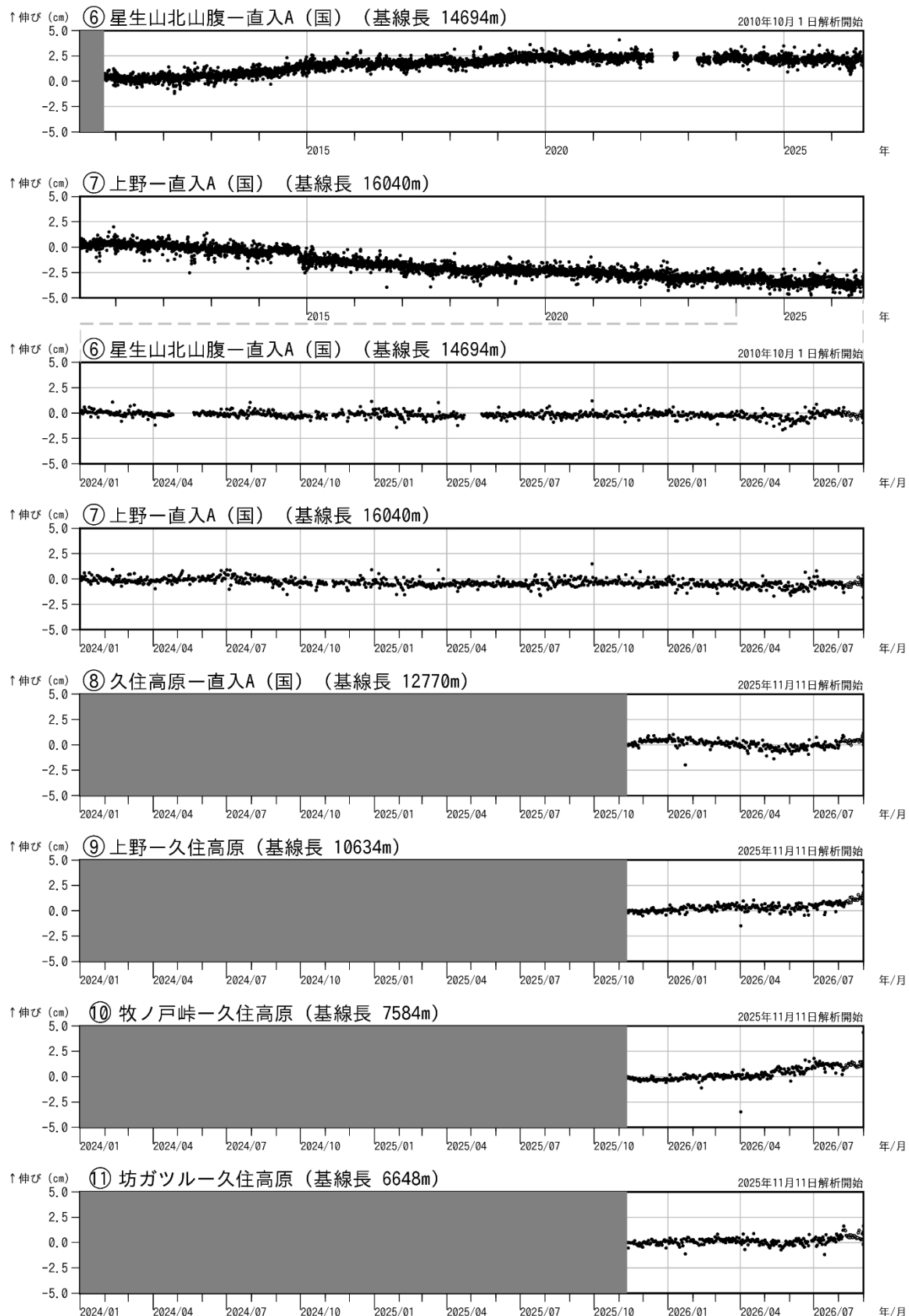
図 5-2 九重山 GNSS 連続観測による基線長変化 (2010 年 1 月～2026 年 8 月)
