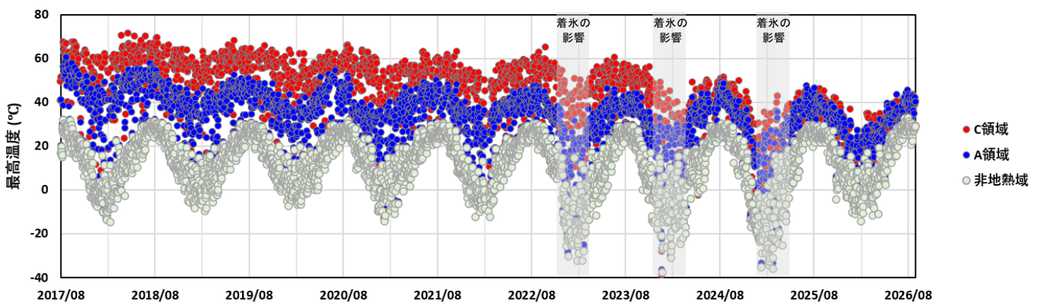
図 1-2 九重山 星生山北尾根の赤外熱映像装置による硫黄山の地熱域の日別最高温度（2017年8月～2026年8月）
