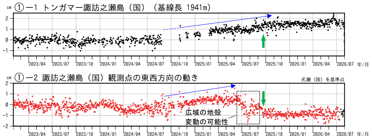
図6-1 諏訪之瀬島 GNSS連続観測（2023年2月～2026年7月）
