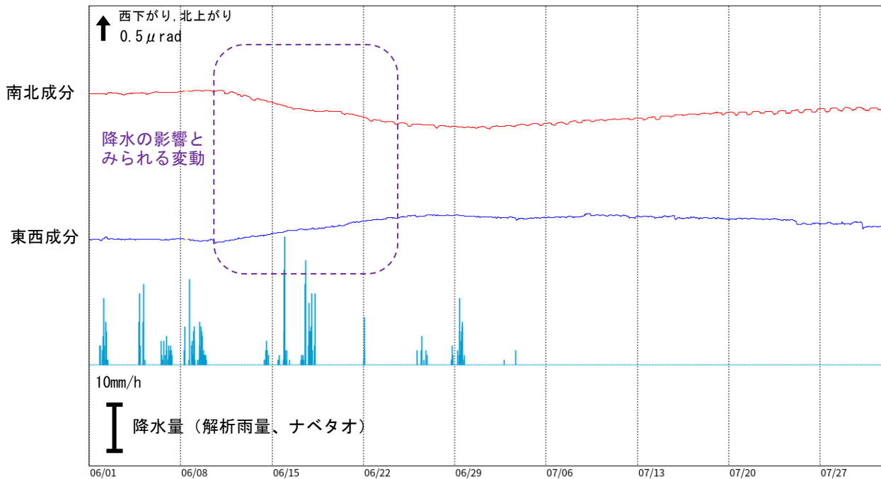
図5 諏訪之瀬島 ナベタオ観測点の傾斜変動（2026年6月～7月）
