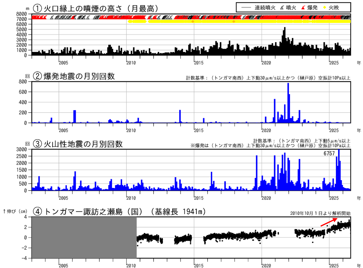
図2 諏訪之瀬島 長期の火山活動経過図（2003年1月～2026年7月）
