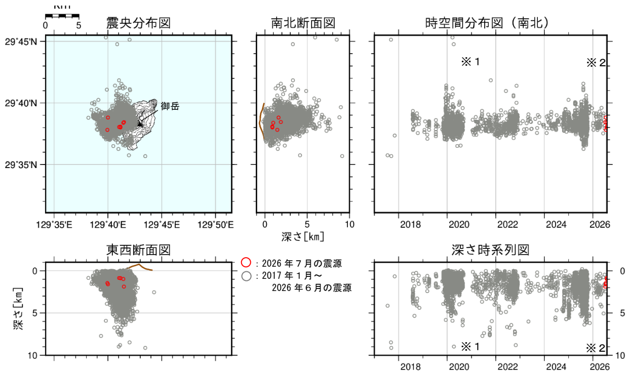
図4 諏訪之瀬島 震源分布図（2017年1月～2026年7月）
