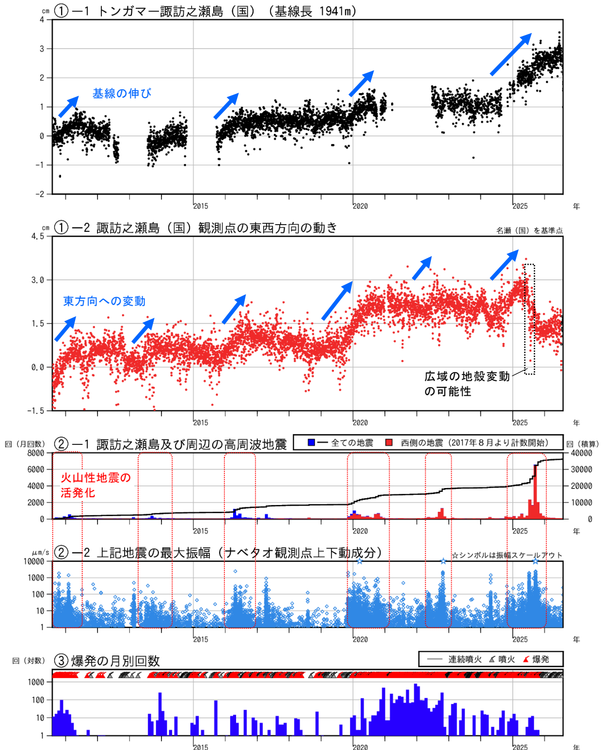
図 6-2 諏訪之瀬島 GNSS連続観測と周辺の火山性地震（2010 年 8 月～2026 年 7 月）
