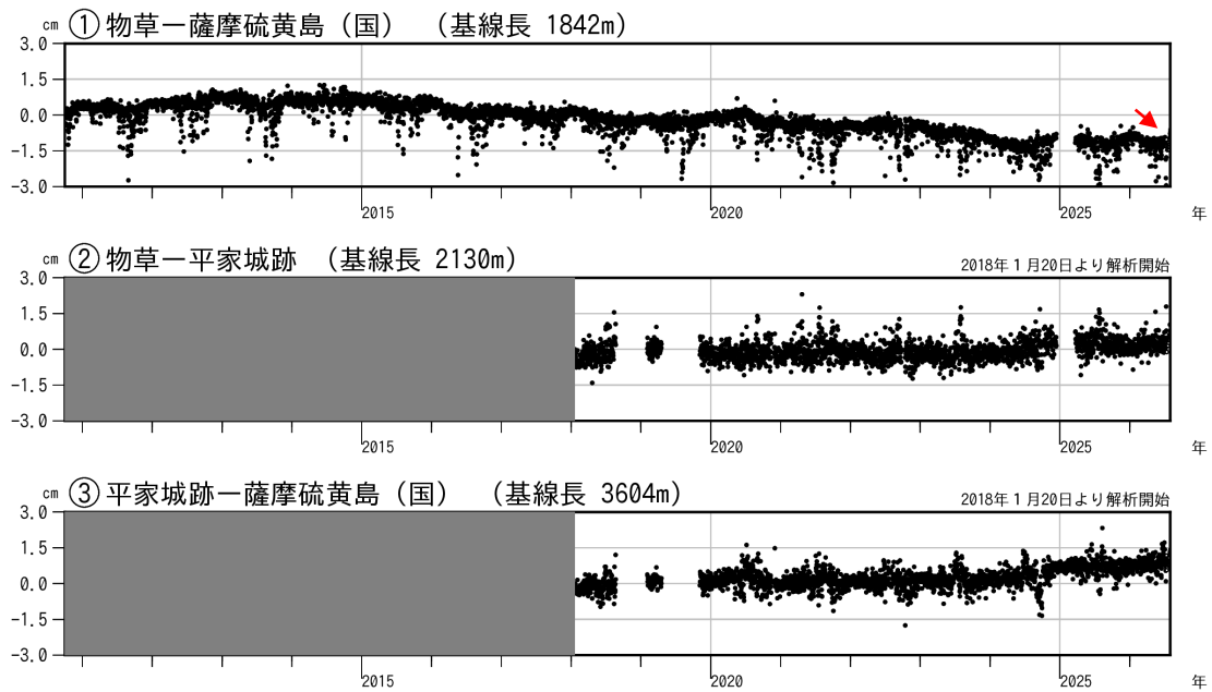
図5 薩摩硫黄島 GNSS連続観測による基線長変化（2010年10月～2026年7月）
