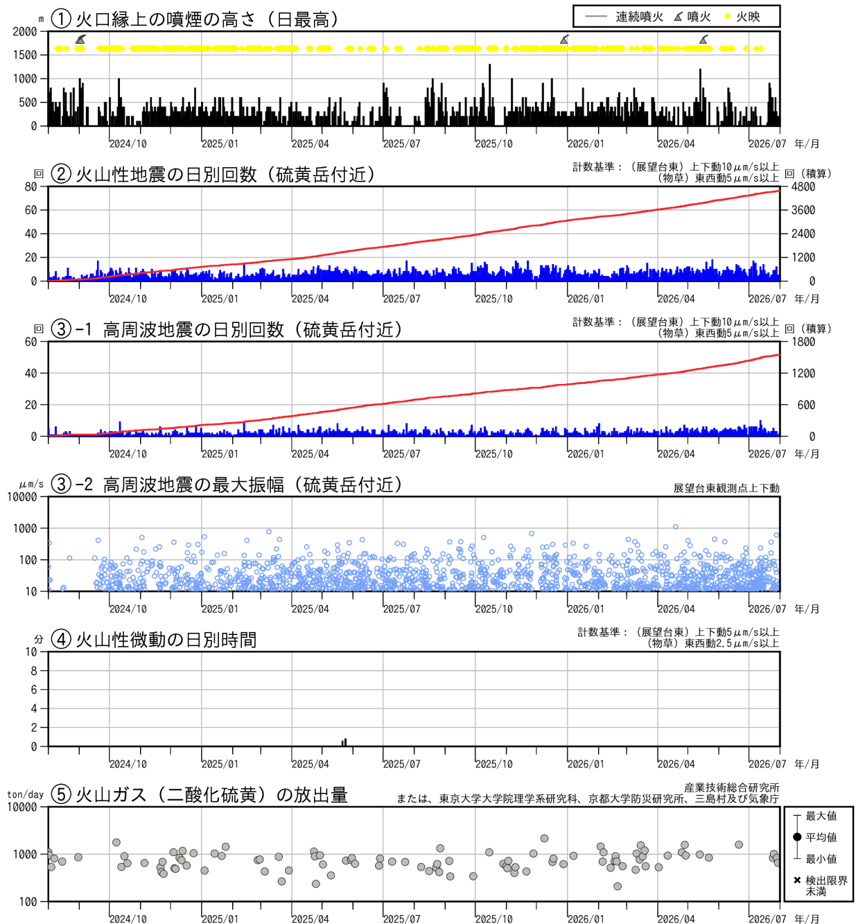
図3 薩摩硫黄島 火山活動経過図（2024年8月～2026年7月）
