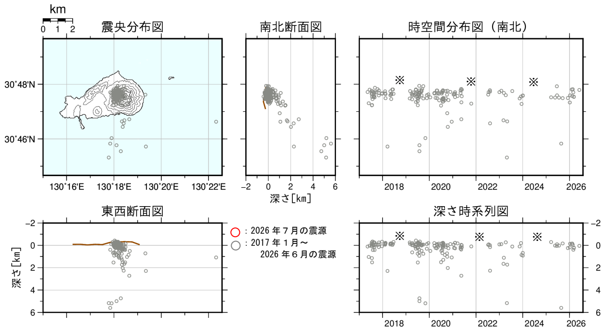
図4 薩摩硫黄島 火山性地震の震源分布図（2017年1月～2026年7月）
