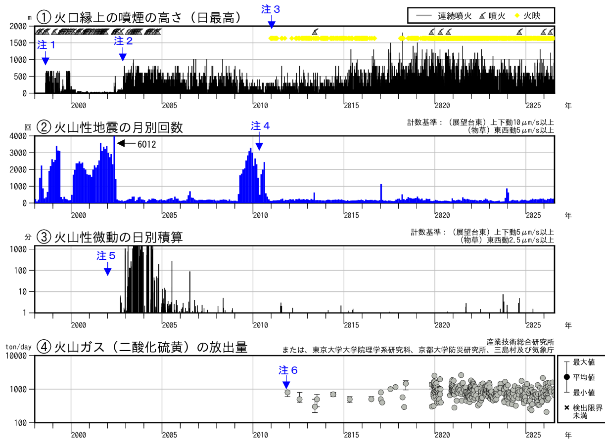
図2 薩摩硫黄島 火山活動経過図（1998年1月～2026年7月）
