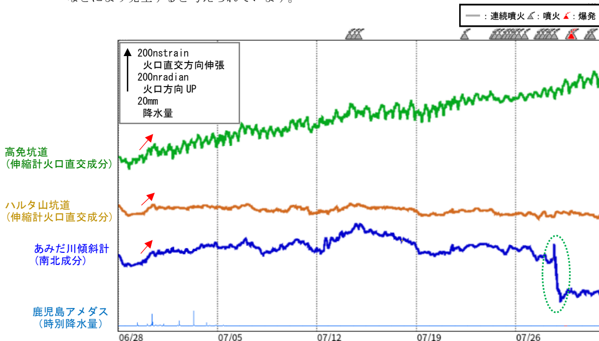
図 6 桜島 傾斜計及び伸縮計による地殻変動の状況（2026年6月28日～7月31日）
