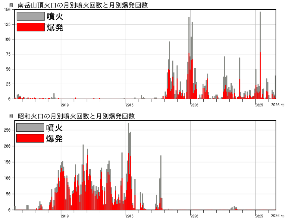
図3 桜島 南岳山頂火口（上図）と昭和火口（下図）の月別噴火回数と月別爆発回数 （2006年6月～2026年7月）
