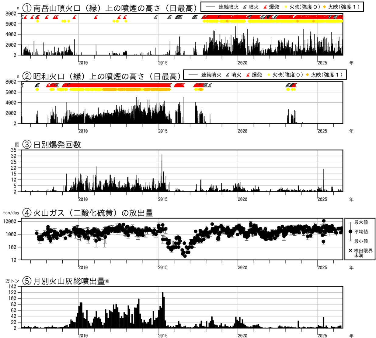
図 5-1 桜島 昭和火口噴火活動再開（2006 年 6 月）以降の活動経過図（2006 年 6 月～2026 年 7 月）
