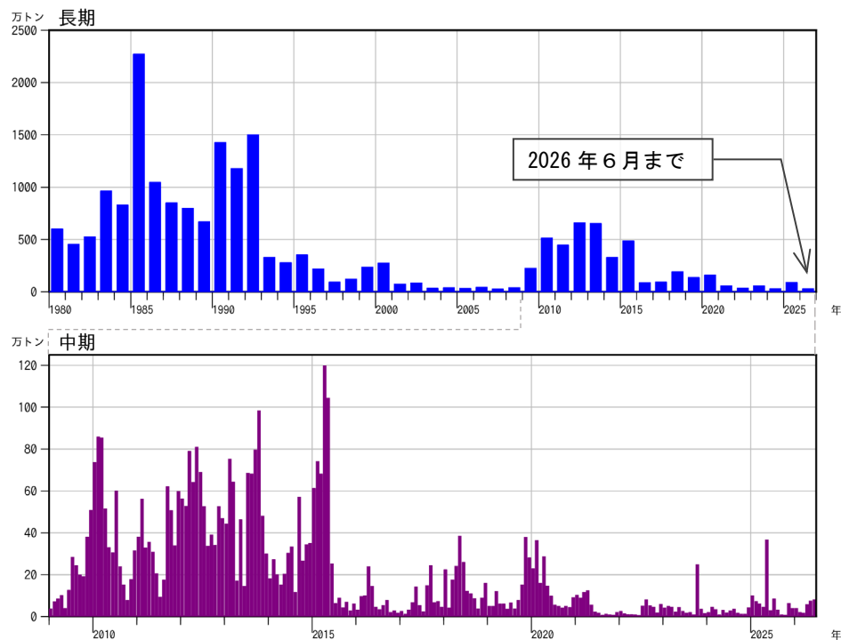
図4 桜島 鹿児島県が実施している降灰の観測データから推定した火山灰の総噴出量 （上段：1980年1月～2026年6月までの年別値、下段：2009年1月～2026年6月の月別値）
