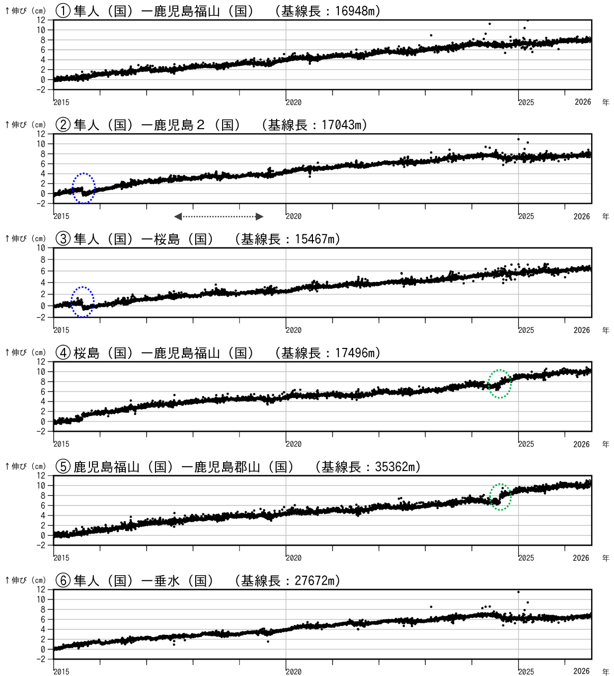
図 7-1 桜島 GNSS 連続観測による基線長変化 (2015 年 1 月～2026 年 7 月)
