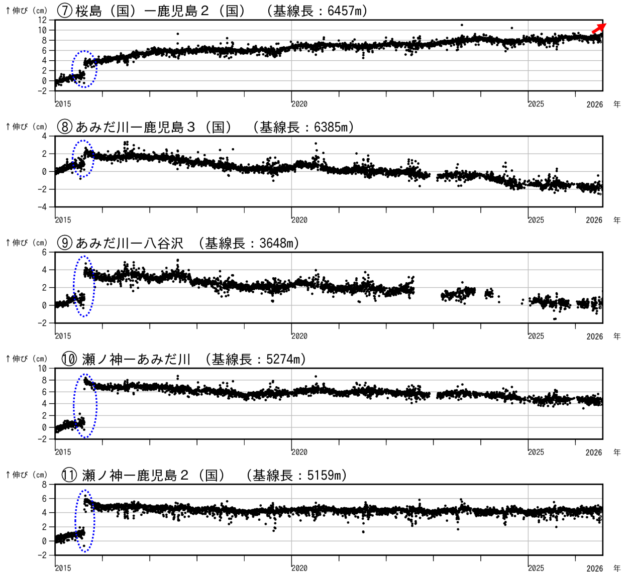
図 7-2 桜島 GNSS 連続観測による基線長変化（2015 年 1 月～2026 年 7 月）
