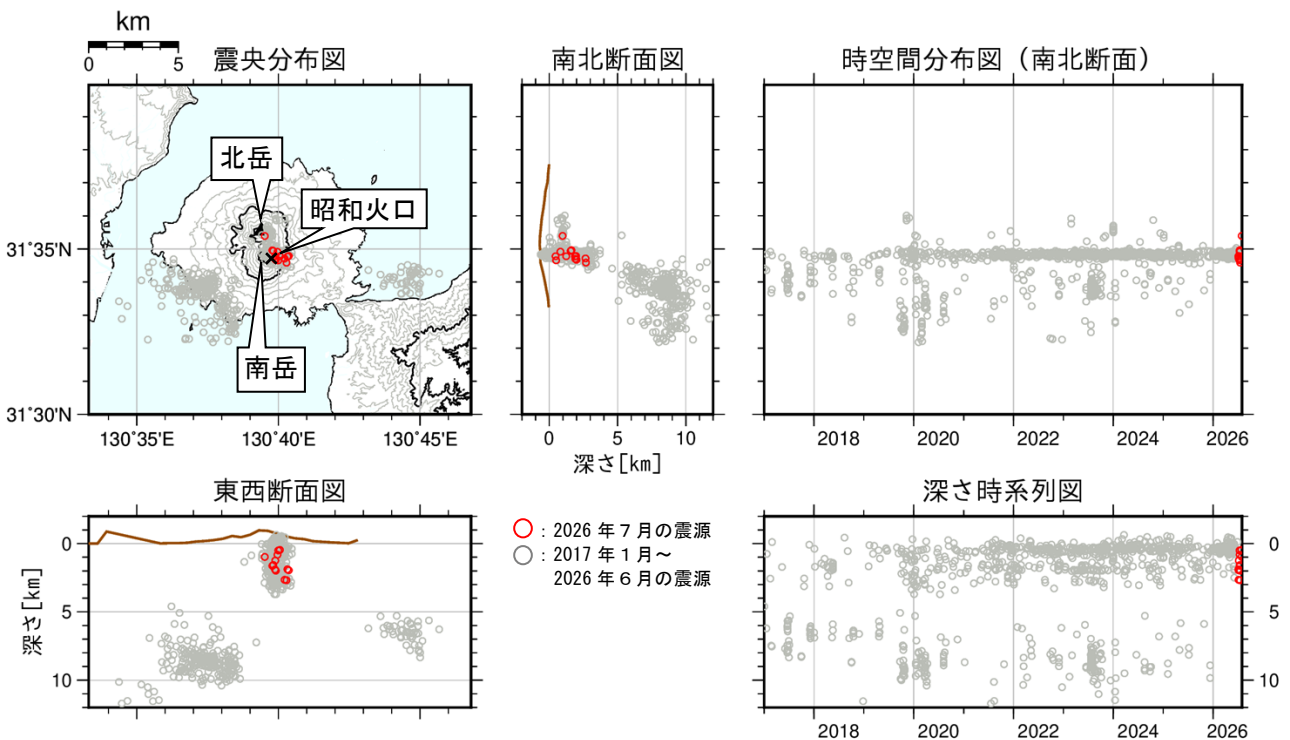
図 2-2 桜島 桜島付近の震源分布図（2017 年 1 月～2026 年 7 月）
