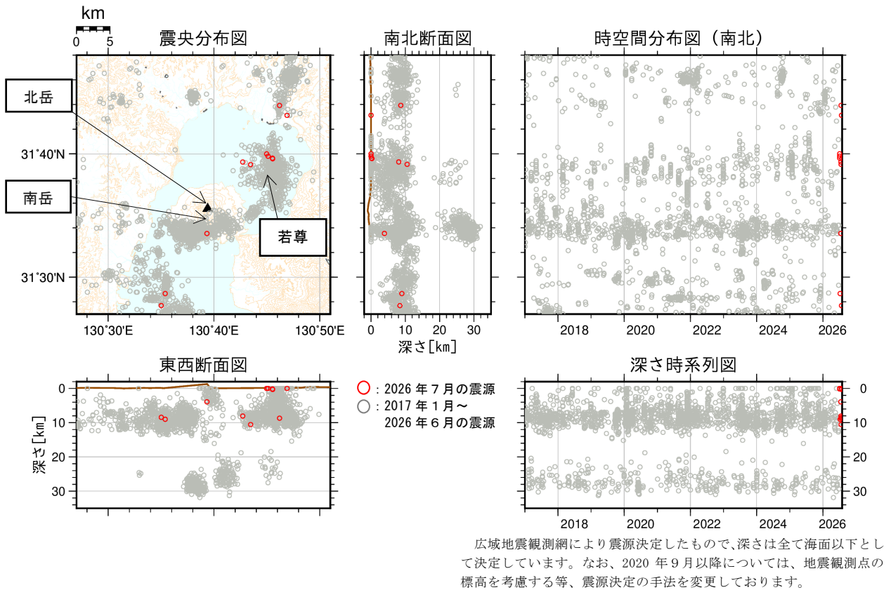
図 2-1 桜島 始良カルデラ周辺の震源分布図（2017 年 1 月～2026 年 7 月）
