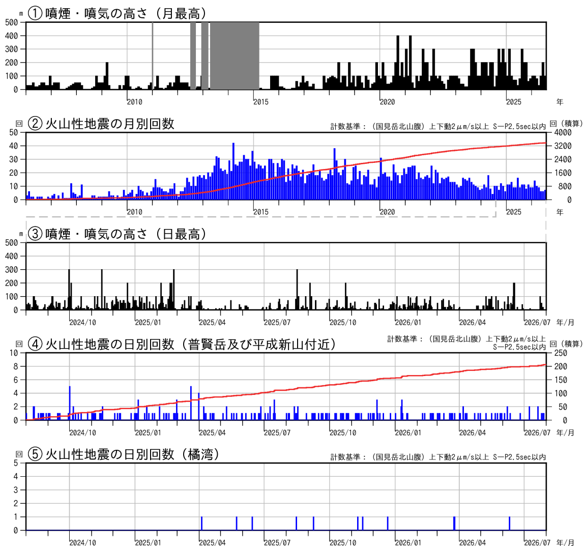
図3 雲仙岳 火山活動経過図（2006年1月～2026年7月）
