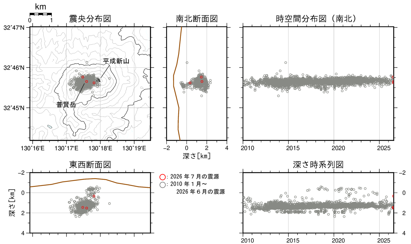
図4 雲仙岳 震源分布図 ①広域図 ②狭域図（2010年1月～2026年7月）
