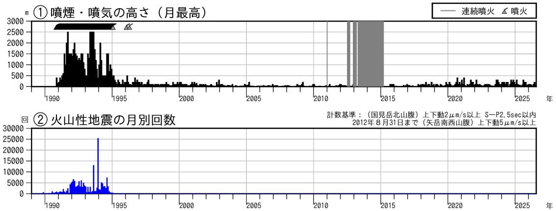
図2 雲仙岳 長期の火山活動経過図（1989年1月～2026年7月）
