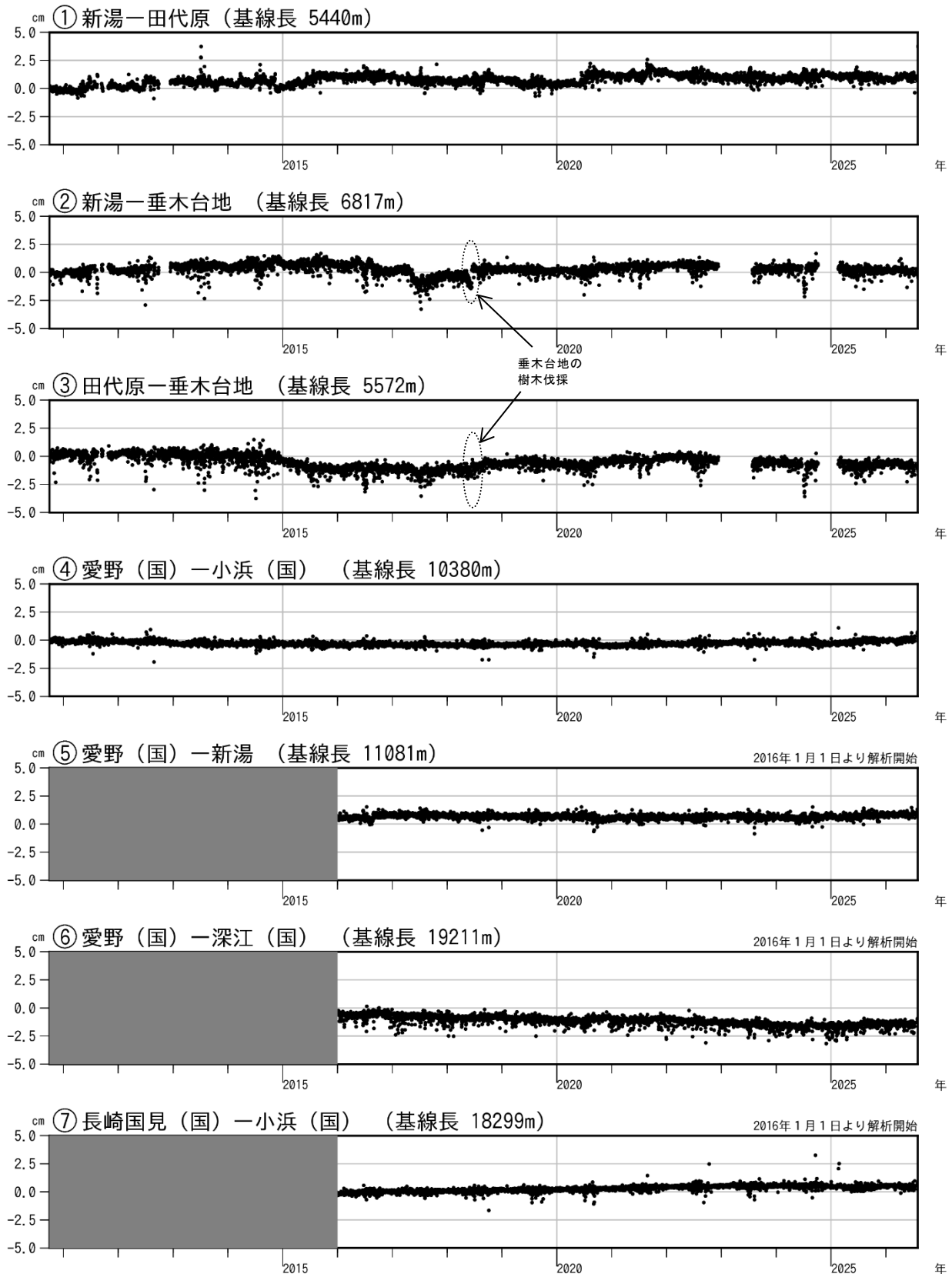
図5 雲仙岳 GNSS連続観測による基線長変化（2010年10月～2026年7月）
