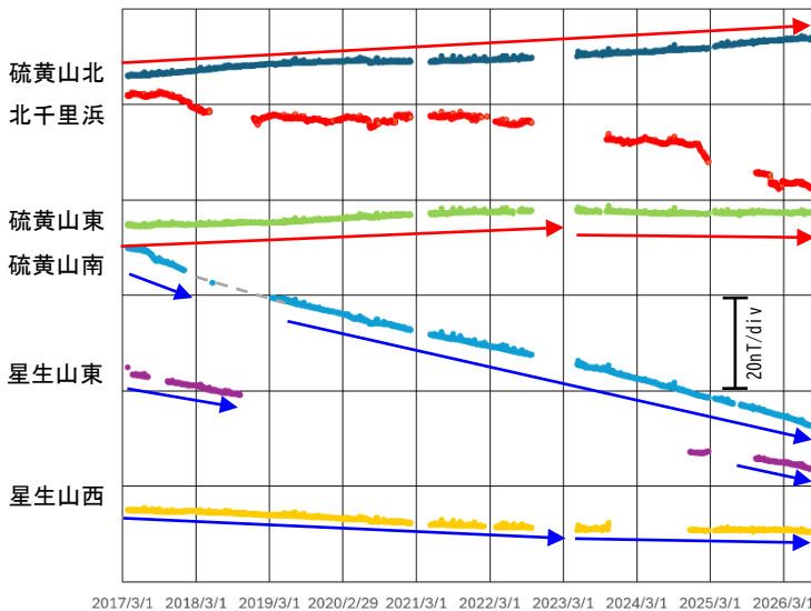
図 4-1 九重山 連続観測による全磁力の変化 (2017 年 3 月～2026 年 7 月)
