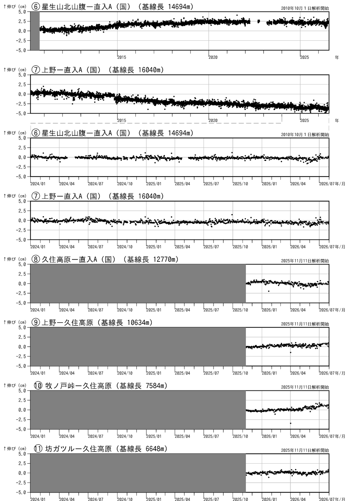
図 5-2 九重山 GNSS 連続観測による基線長変化（2010 年 1 月～2026 年 7 月）
