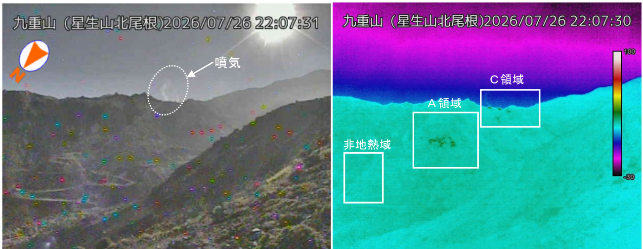
図 1-1 九重山 硫黄山の噴気及び地熱域の状況（7月26日 星生山北尾根監視カメラ）
