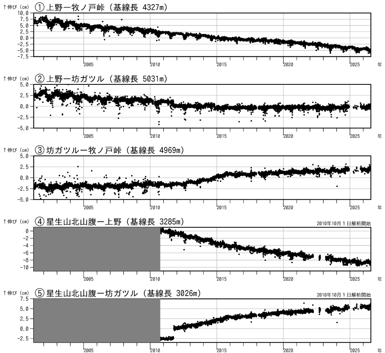
図 5-1 九重山 GNSS 連続観測による基線長変化（2001 年 4 月～2026 年 7 月）
