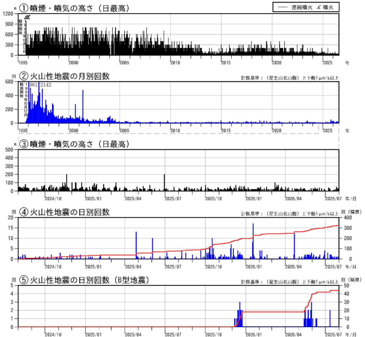
図2 九重山 火山活動経過図（1995年1月～2026年7月）
