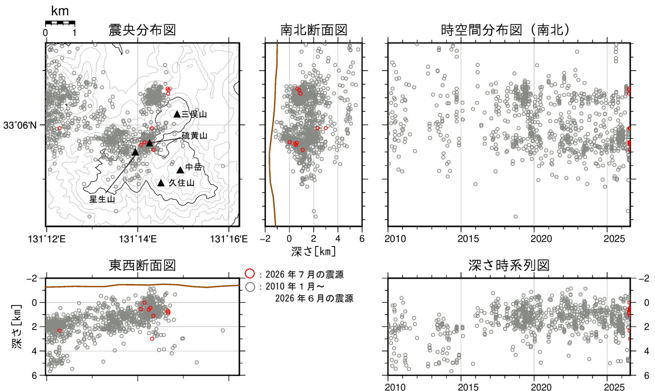
図3 九重山 震源分布図 ①広域図 ②狭域図（2010年1月～2026年7月）
