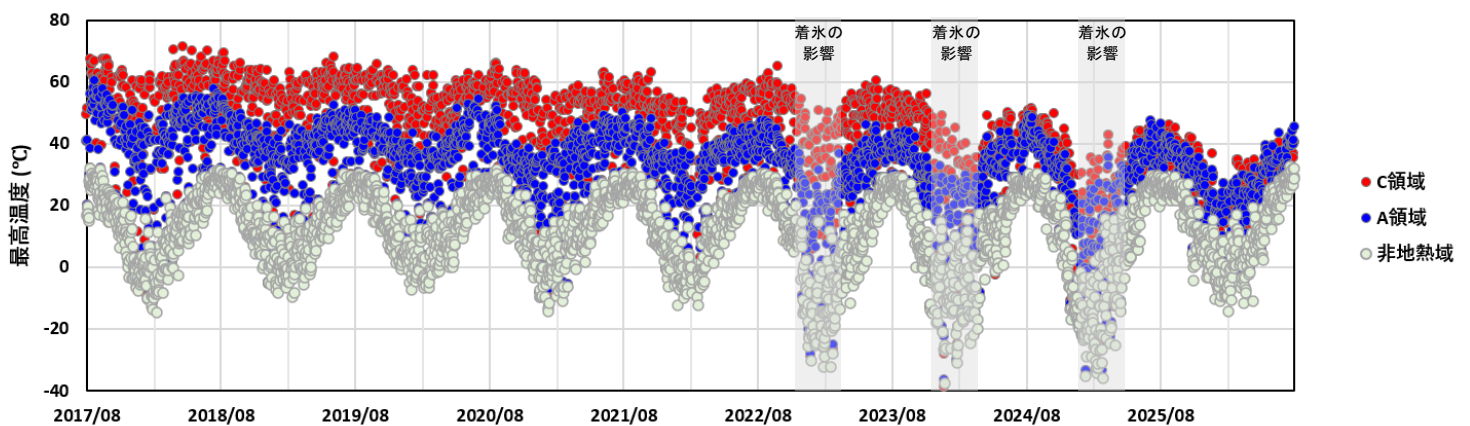
図 1-2 九重山 星生山北尾根の赤外熱映像装置による硫黄山の地熱域の日別最高温度（2017年8月～2026年7月）
