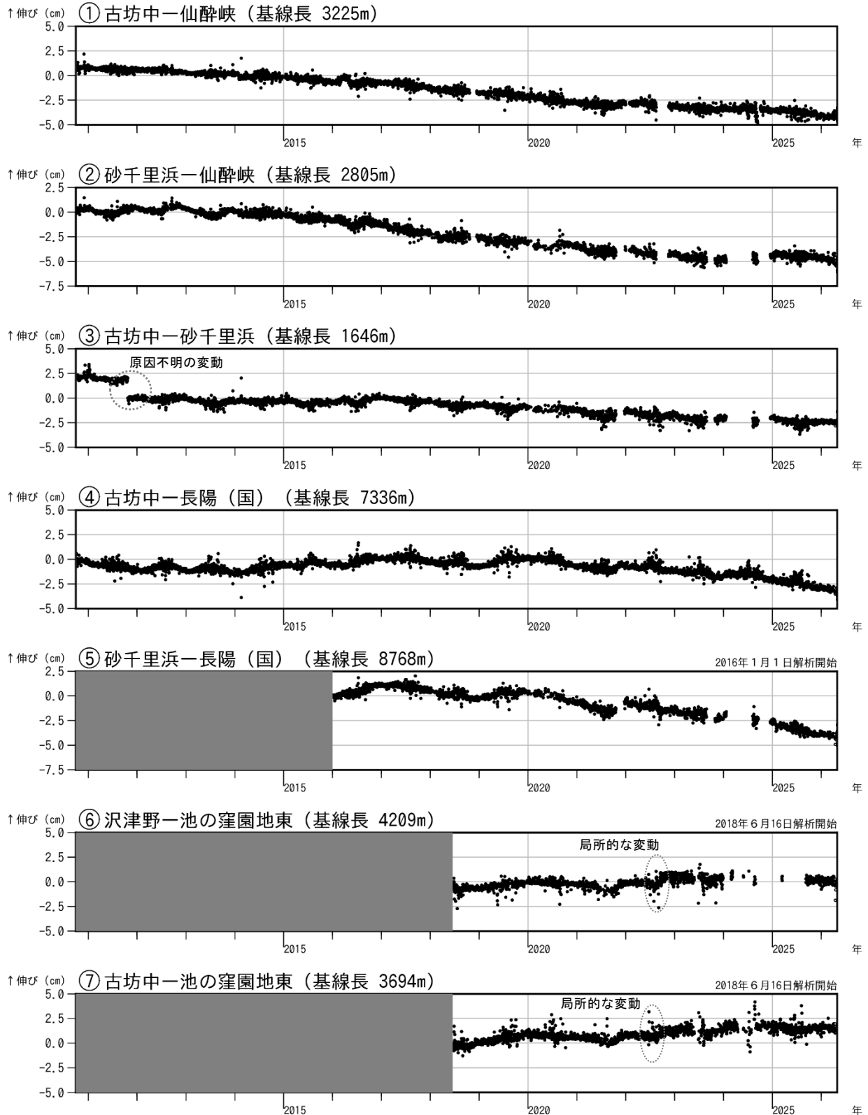
図5 阿蘇山 GNSS 連続観測による基線長変化（2010年10月～2026年4月）
