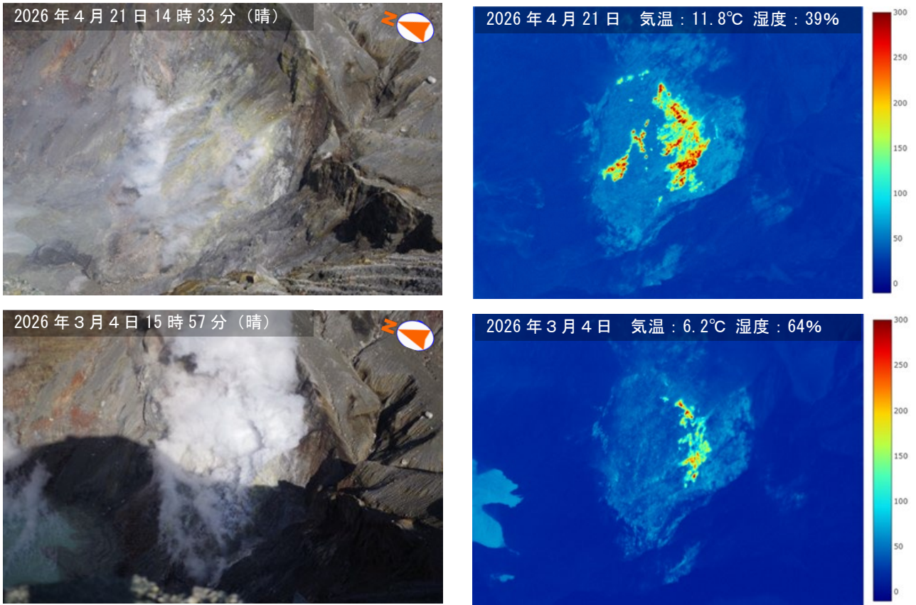
図 2-2 阿蘇山 中岳第一火口 南側火口壁の状況 （火口南西側観測定点から撮影 上図：4月21日、下図：3月4日）
