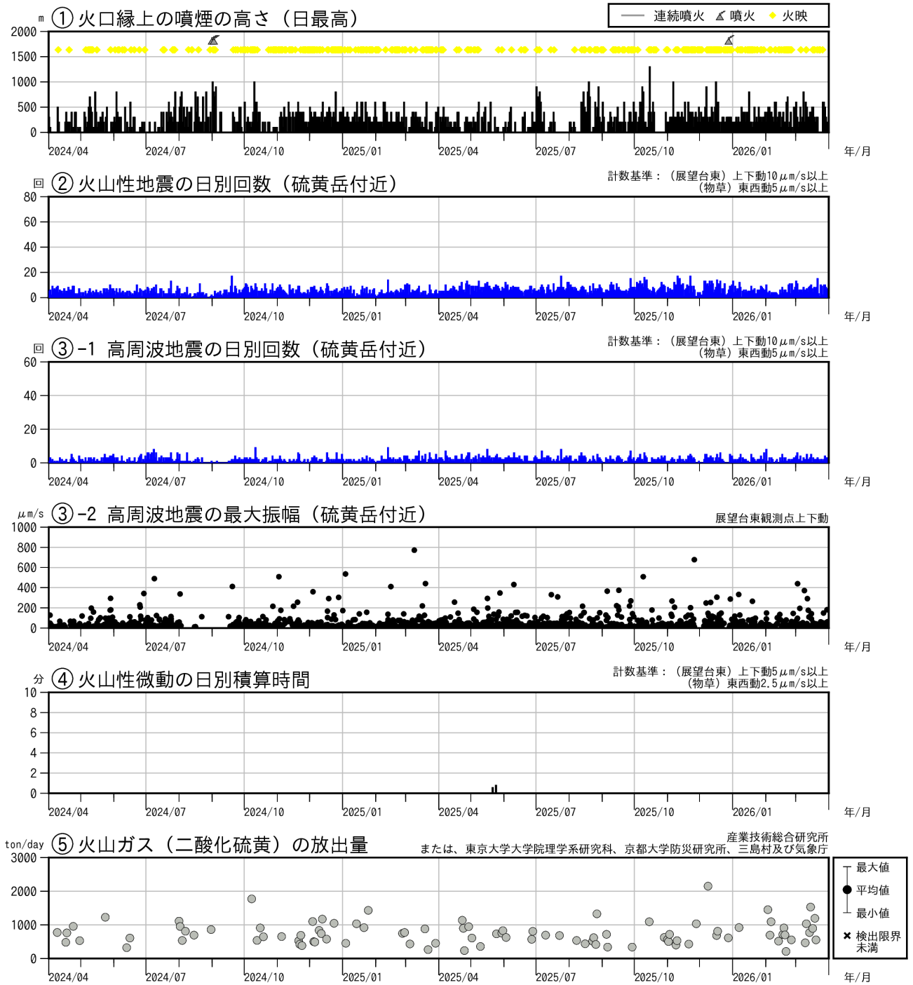
図3 薩摩硫黄島 火山活動経過図（2024年4月～2026年3月）
