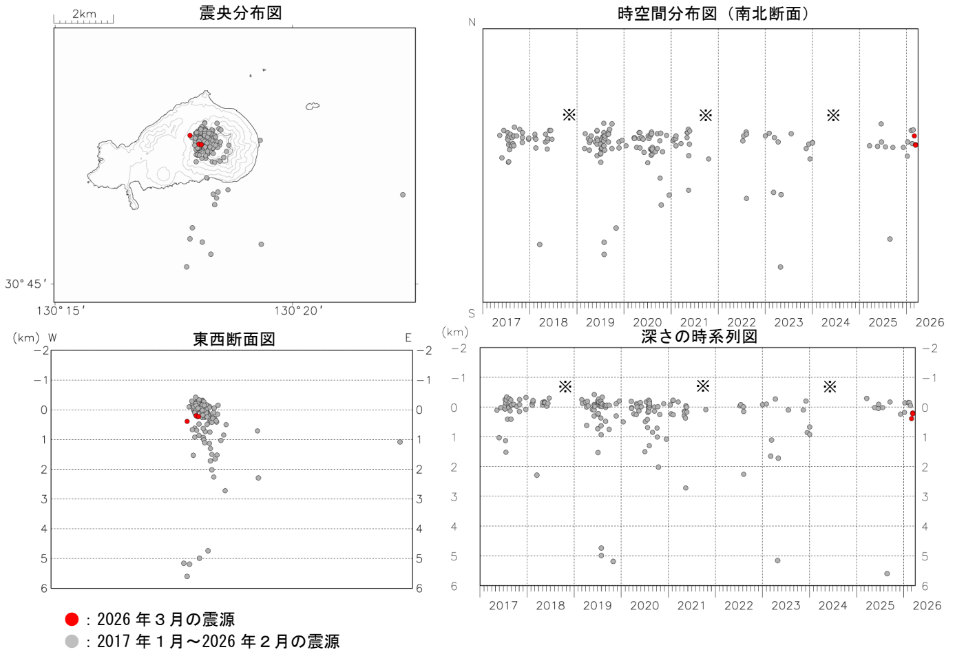
図4 薩摩硫黄島 火山性地震の震源分布図（2017年1月～2026年3月）
