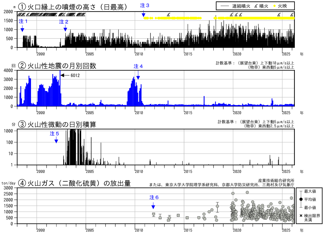
図2 薩摩硫黄島 火山活動経過図（1998年1月～2026年3月）
