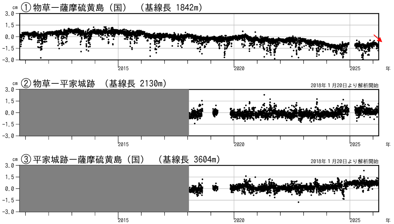
図5 薩摩硫黄島 GNSS連続観測による基線長変化（2010年10月～2026年3月）
