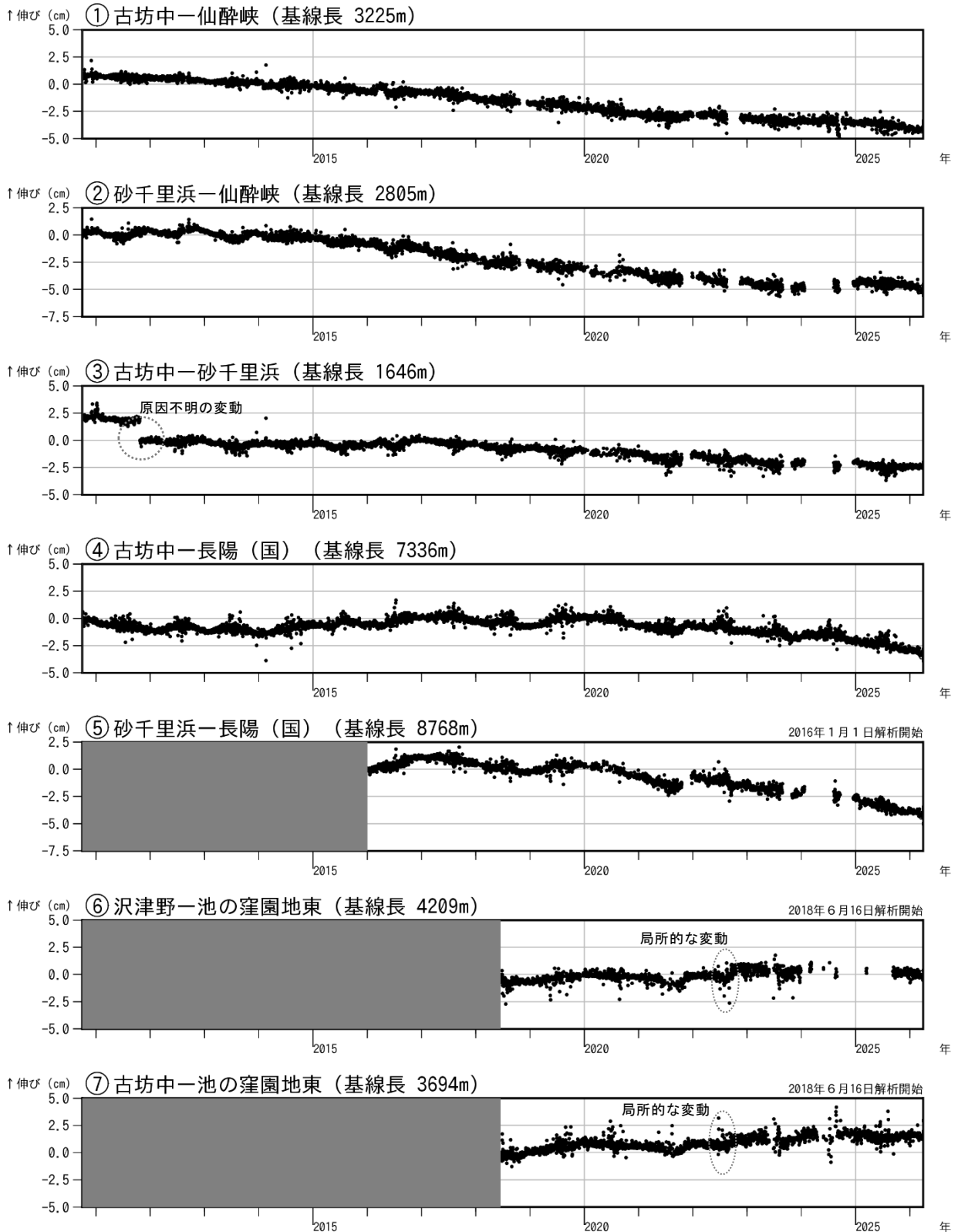
図5 阿蘇山 GNSS 連続観測による基線長変化（2010年10月～2026年3月）
