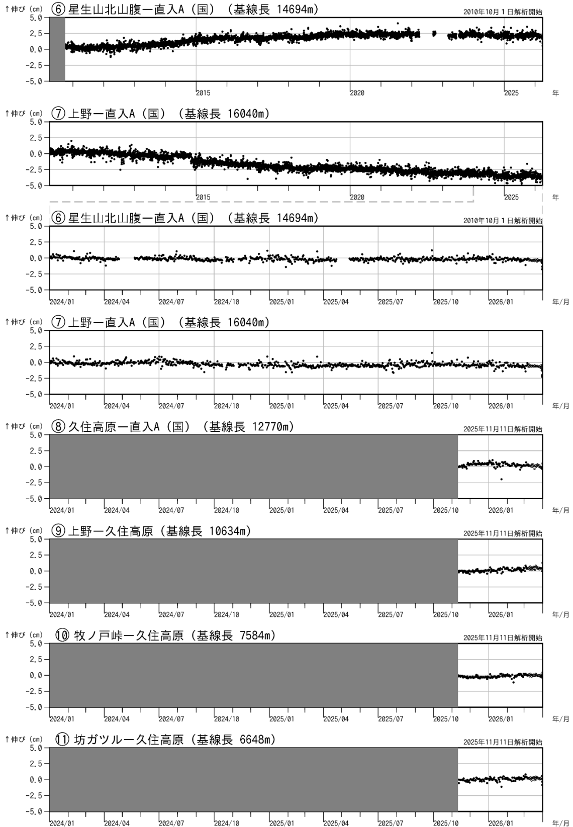
図 5-2 九重山 GNSS 連続観測による基線長変化（2010 年 1 月～2026 年 3 月）
