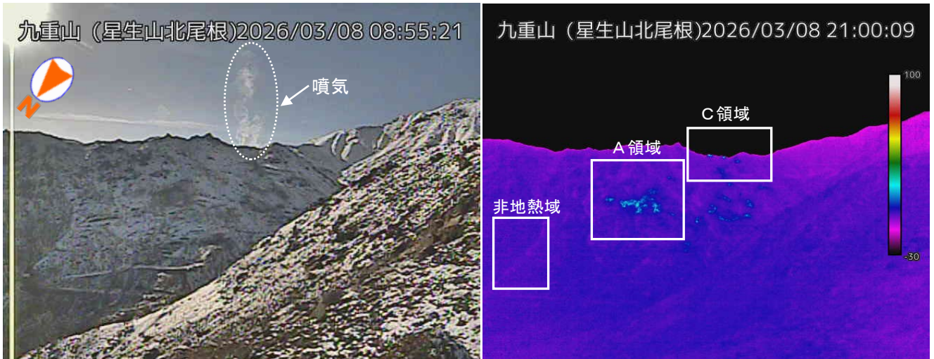
図 1-1 九重山 硫黄山の噴気及び地熱域の状況（3月8日 星生山北尾根監視カメラ）
