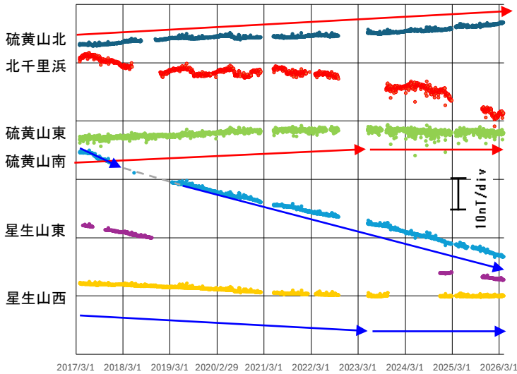
図 4-1 九重山 連続観測による全磁力の変化 (2017年3月～2026年3月)
