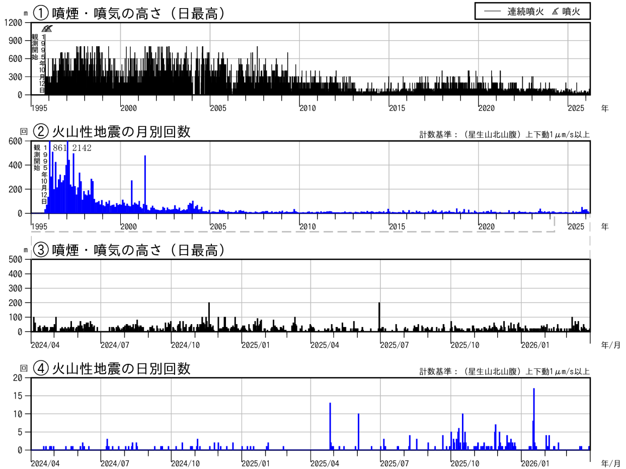
図2 九重山 火山活動経過図（1995年1月～2026年3月）
