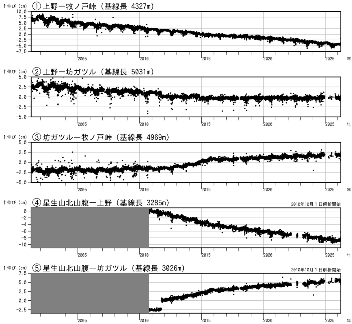
図 5-1 九重山 GNSS 連続観測による基線長変化（2001 年 4 月～2026 年 3 月）
