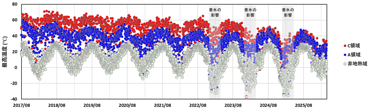
図 1-2 九重山 星生山北尾根の赤外熱映像装置による日別最高温度（2017年8月～2026年3月）
