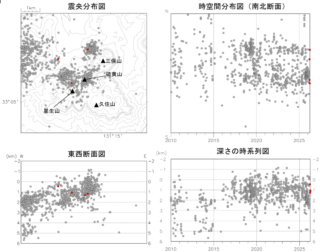
図3 九重山 震源分布図 ①広域図 ②狭域図 (2010年1月～2026年3月)
