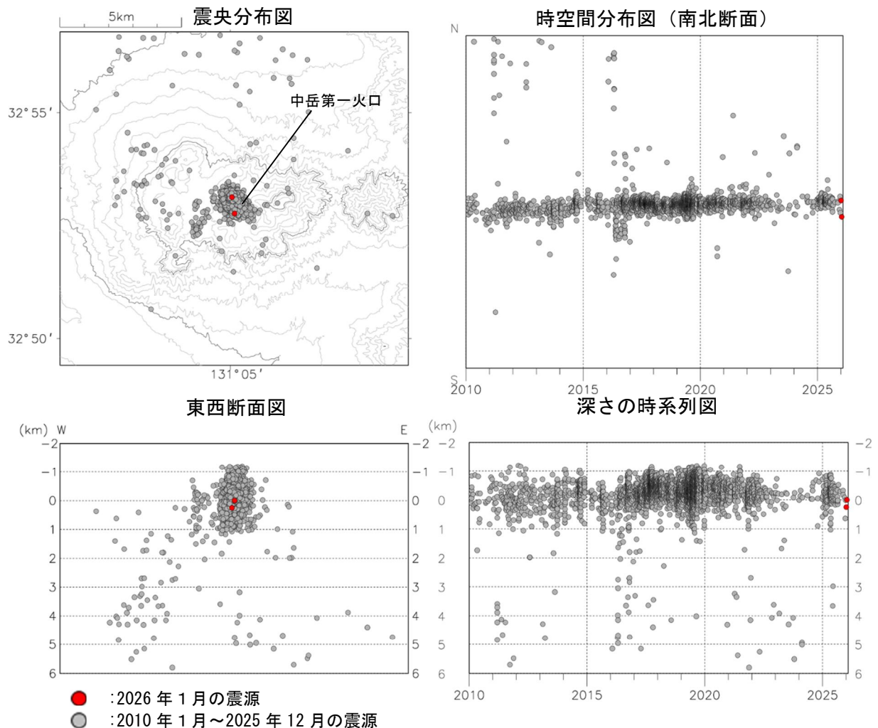
図4 阿蘇山 火山性地震の震源分布
