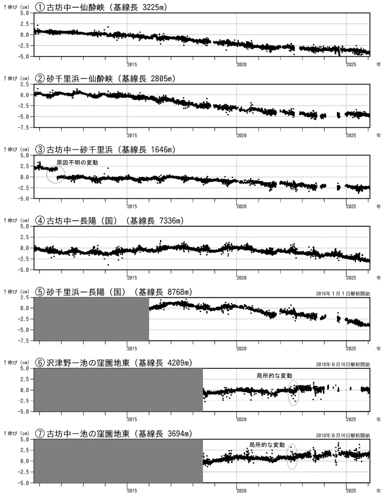
図5 阿蘇山 GNSS 連続観測による基線長変化（2010年10月～2026年1月）
