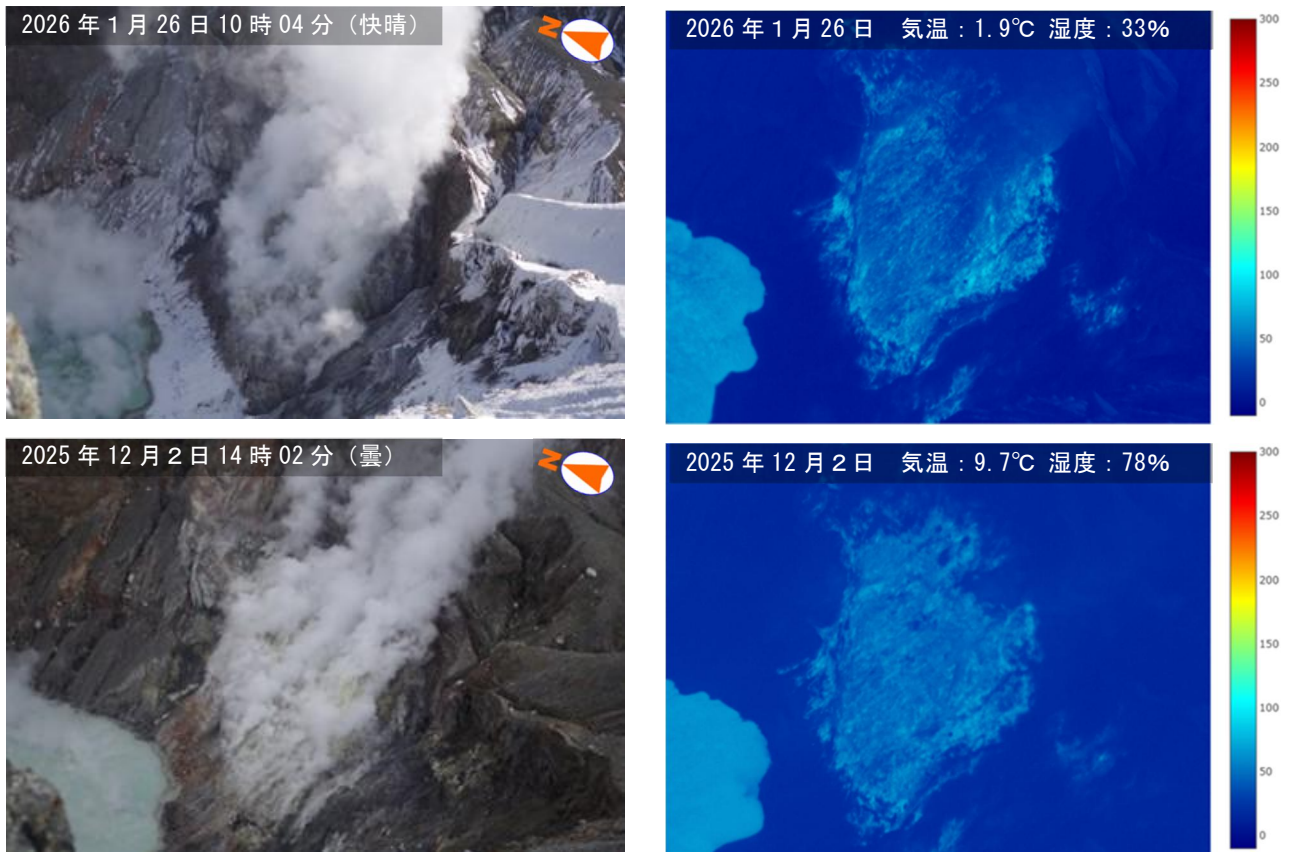
図 2-2 阿蘇山 中岳第一火口 南側火口壁の状況 （火口南西側観測定点から撮影 上図：2026 年 1 月 26 日、下図：2025 年 12 月 2 日）
