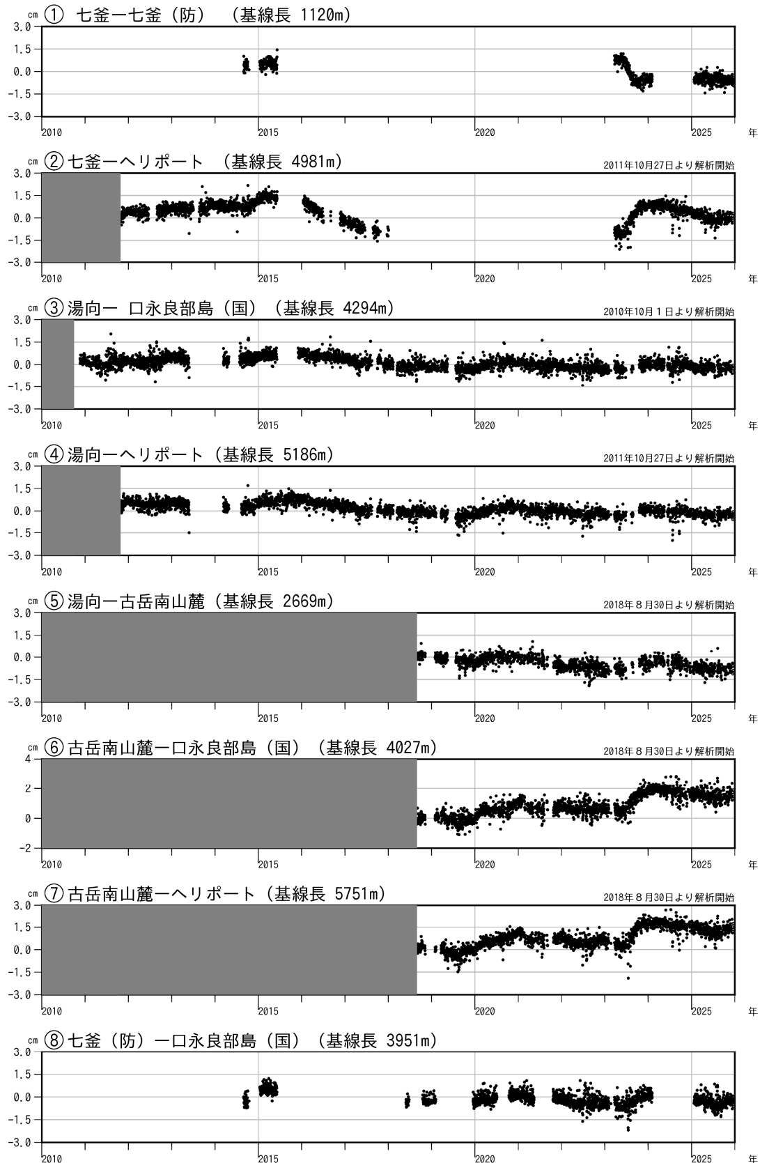
図 6 口永良部島 GNSS 連続観測による基線長変化（2010 年 1 月～2025 年 12 月）
