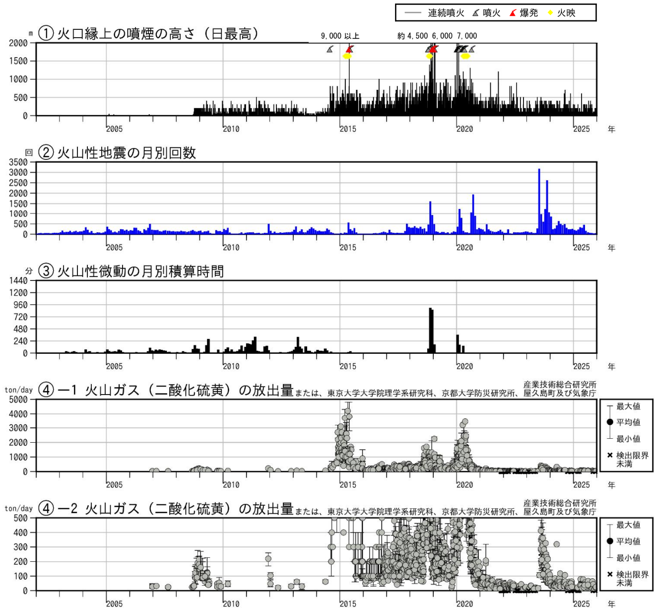
図 3 口永良部島 火山活動経過図（2002 年 1 月～2025 年 12 月）
