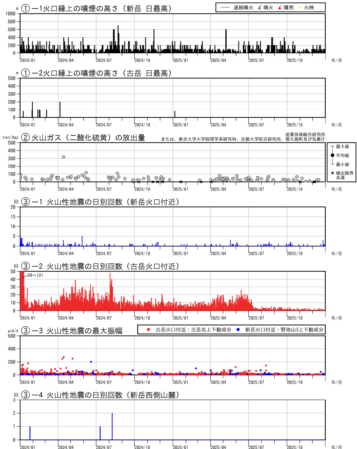
図4 口永良部島 最近の火山活動経過図（2024年1月～2025年12月）
