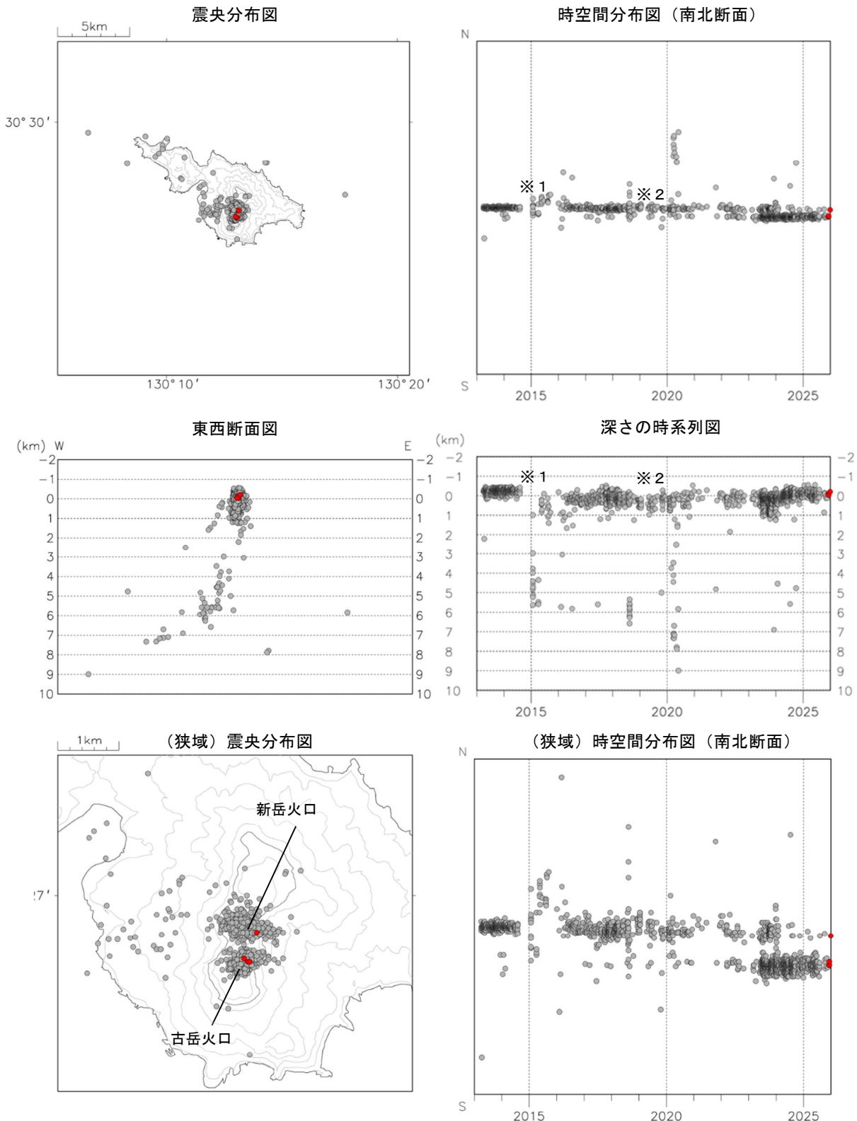
図5 口永良部島 震源分布図（2013年1月～2025年12月）
