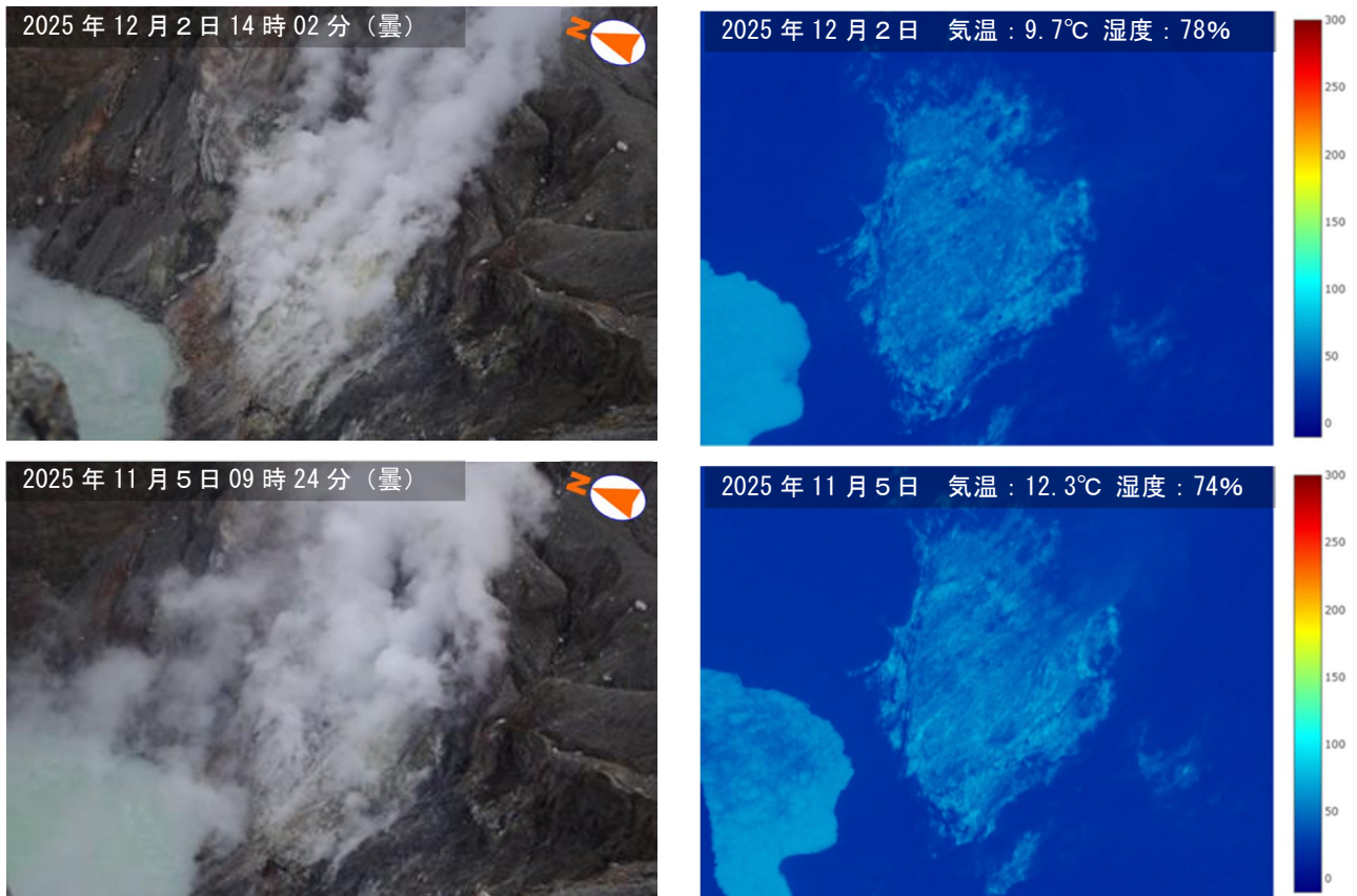
図 2-2 阿蘇山 中岳第一火口 南側火口壁の状況 （火口南西側観測定点から撮影 上図：12月2日、下図：11月5日）
