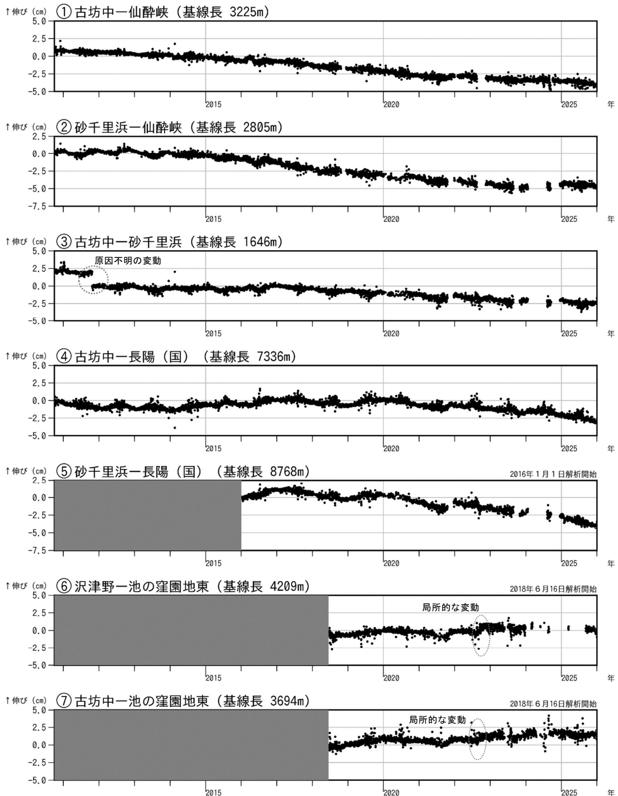
図5 阿蘇山 GNSS 連続観測による基線長変化（2010 年 10 月～2025 年 12 月）
