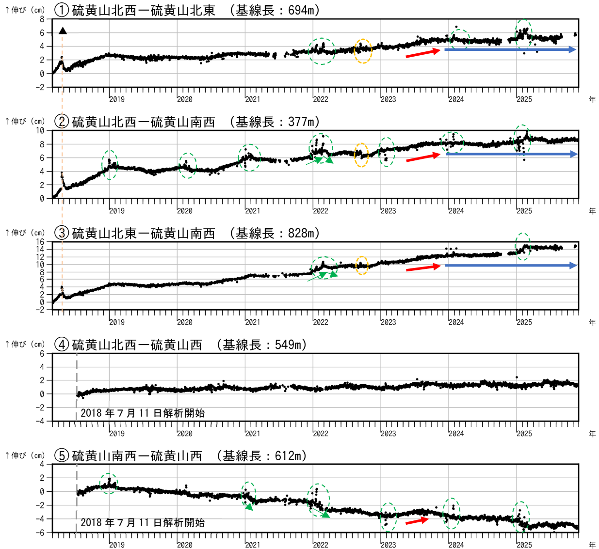
図6 霧島山（えびの高原（硫黄山）周辺） GNSS 連続観測による基線長変化（2018年3月～2025年11月）
