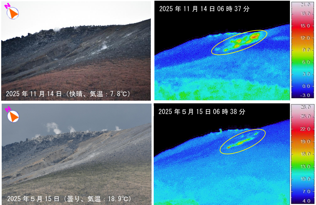
図 2-2 霧島山（新燃岳） 新燃岳西側斜面の割れ目付近の状況（新湯温泉付近からの観測）
