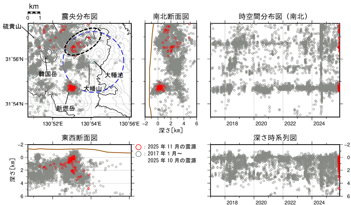
図3 霧島山（大幡池） 震源分布図（2017年1月～2025年11月）
