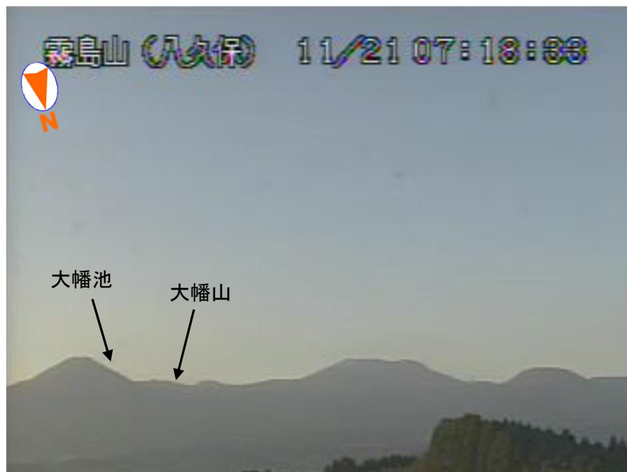
図1 霧島山（大幡池） 大幡池及び大幡山の状況（11月21日、八久保監視カメラ）
