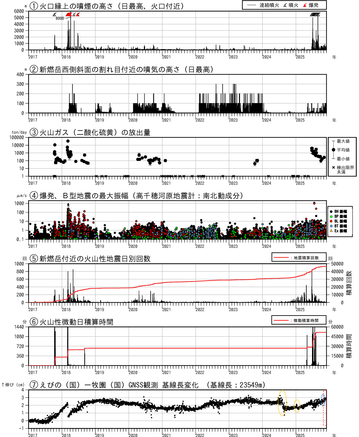
図 3-1 霧島山（新燃岳） 火山活動経過図（2017 年 1 月～2025 年 11 月）
