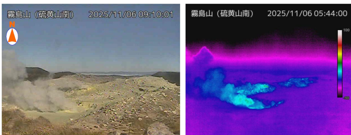
図 1-2 霧島山（えびの高原（硫黄山）周辺） 硫黄山南側の状況 （11 月 6 日、硫黄山南監視カメラ）
