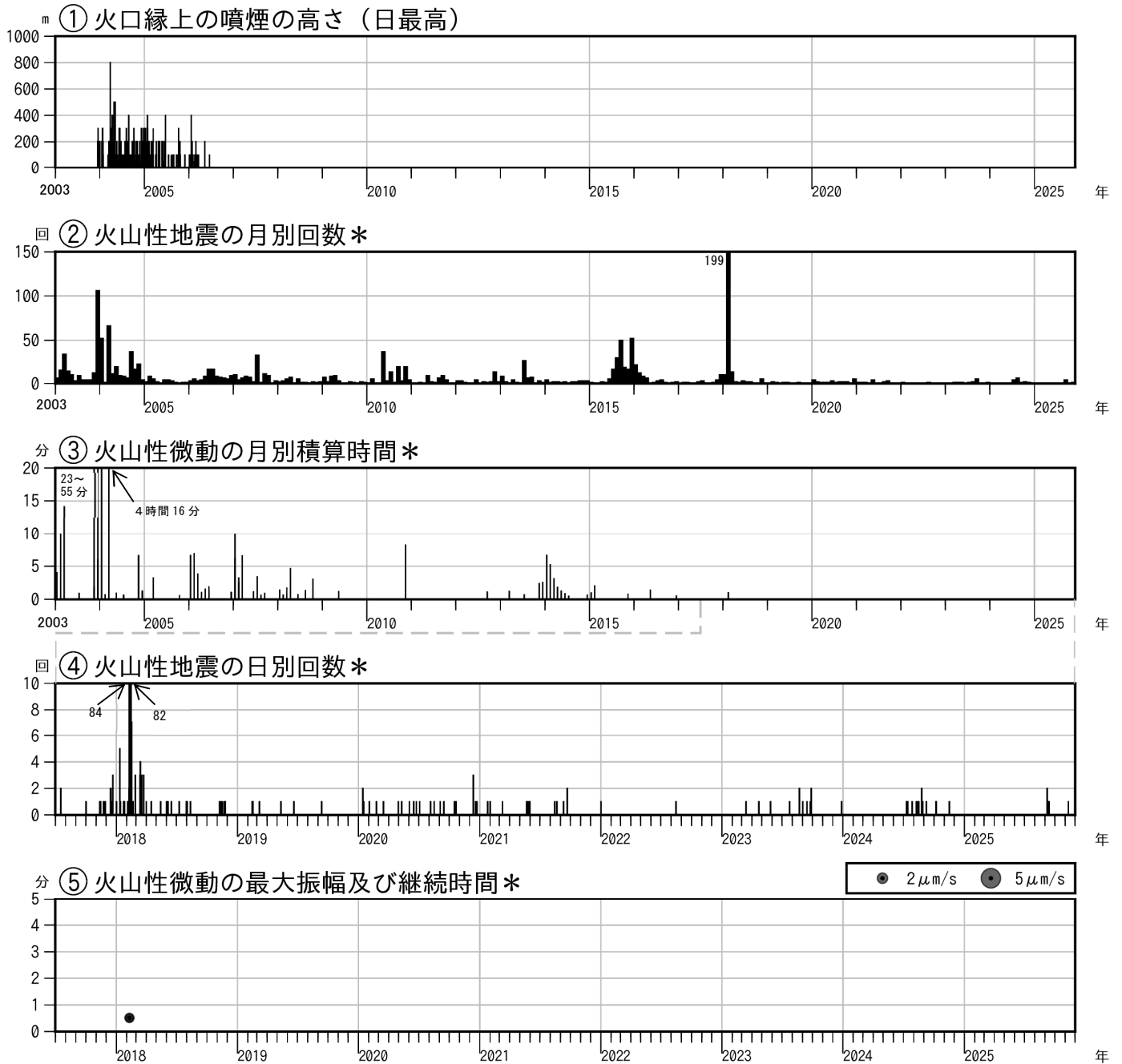
図3 霧島山（御鉢） 火山活動経過図（2003年1月～2025年11月）
