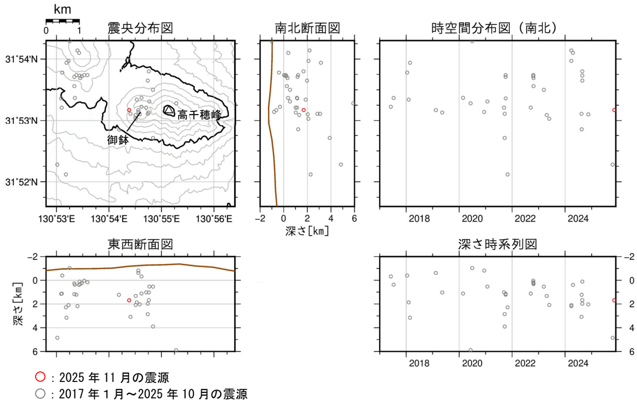
図2 霧島山（御鉢） 震源分布図（2017 年 1 月～2025 年 11 月）
