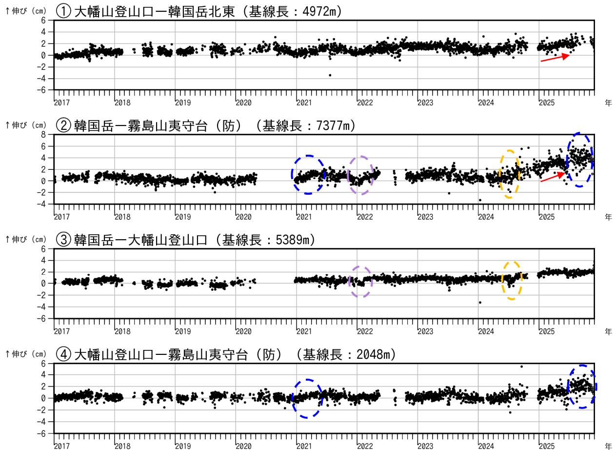
図4 霧島山（大幡池） GNSS 連続観測による基線長変化（2017年1月～2025年11月）
