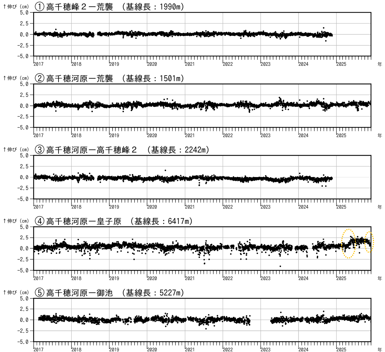
図4 霧島山（御鉢） GNSS 連続観測による基線長変化（2017年1月～2025年11月）
