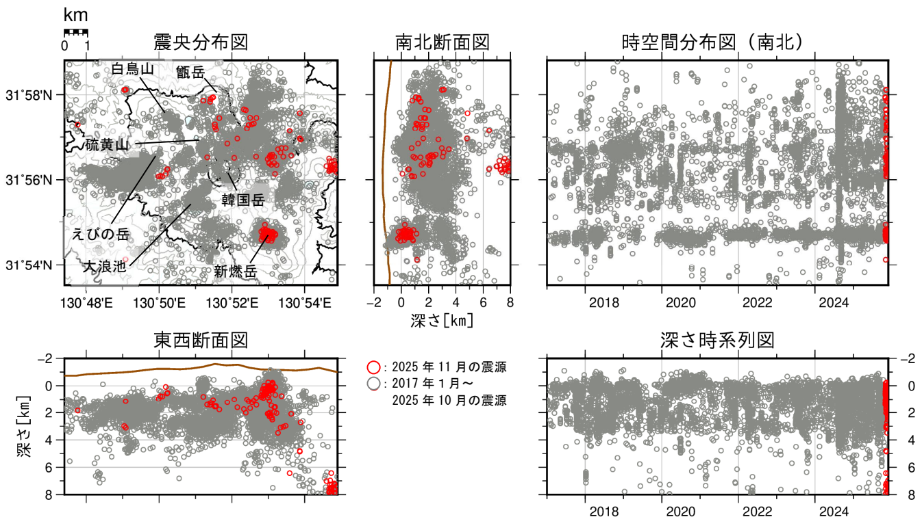
図5 霧島山（えびの高原（硫黄山）周辺）震源分布図（2017年1月～2025年11月）
