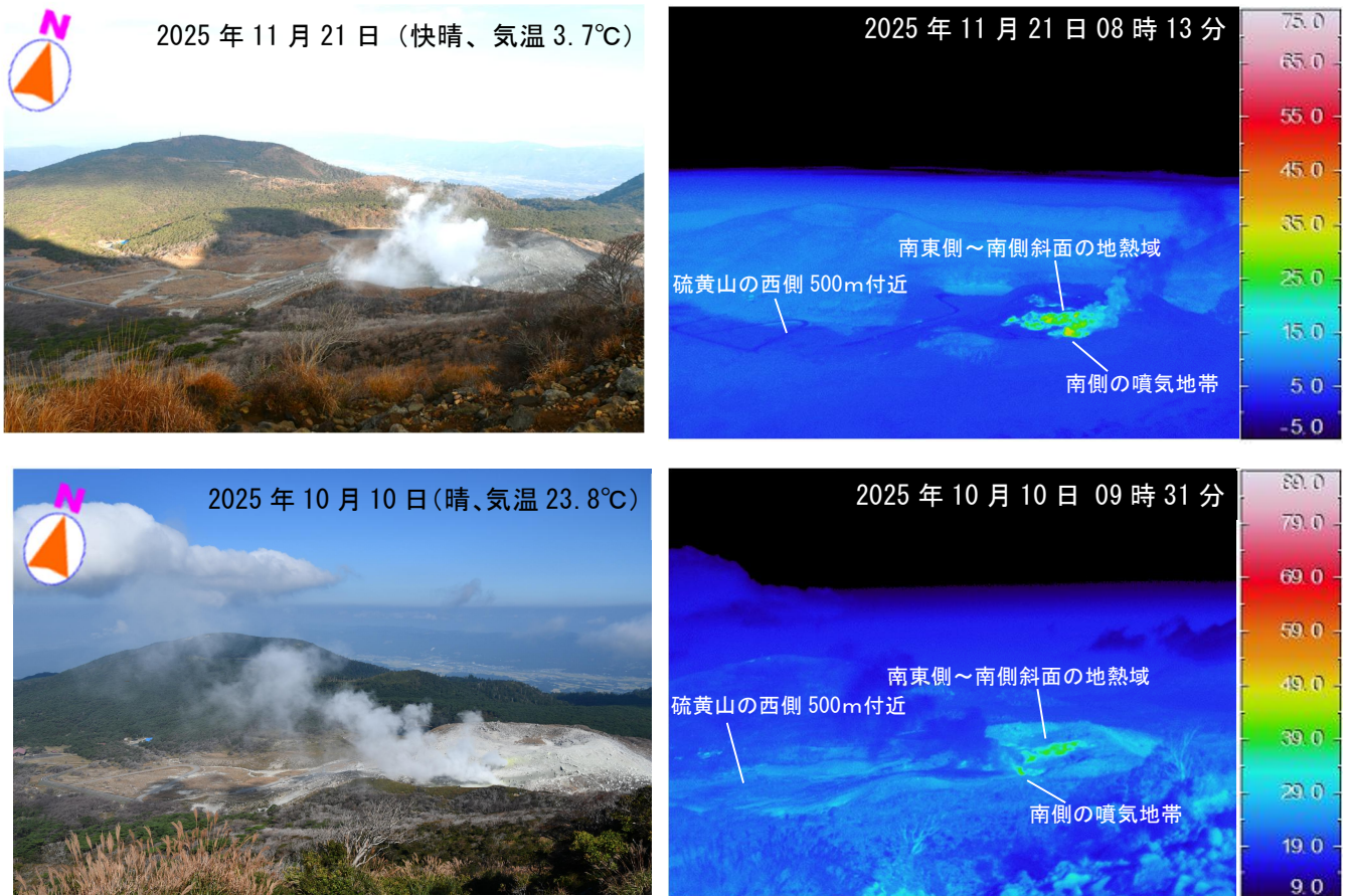
図2 霧島山（えびの高原（硫黄山）周辺） 硫黄山の火口及びその周辺の状況
