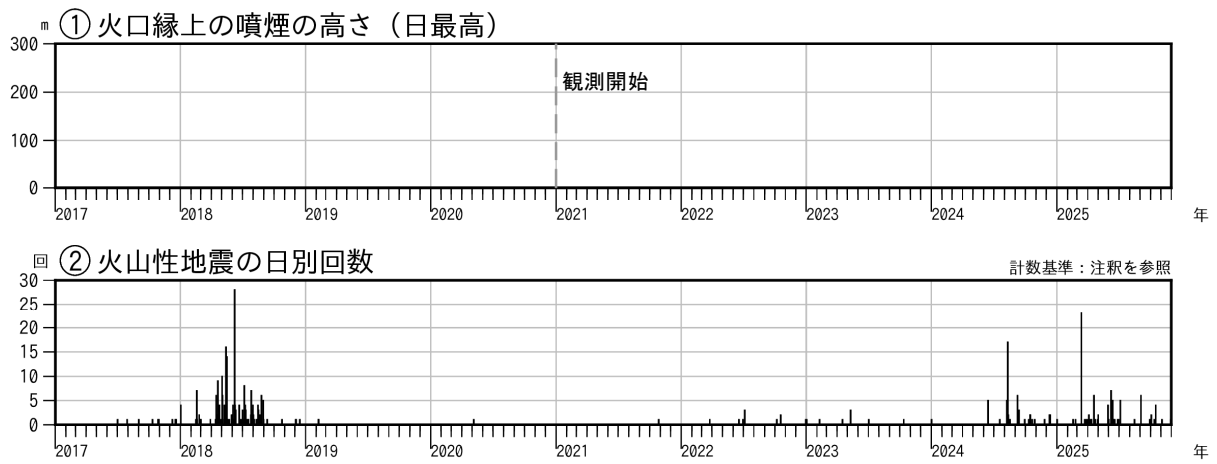
図2 霧島山（大幡池） 火山活動経過図（2017年1月～2025年11月）
