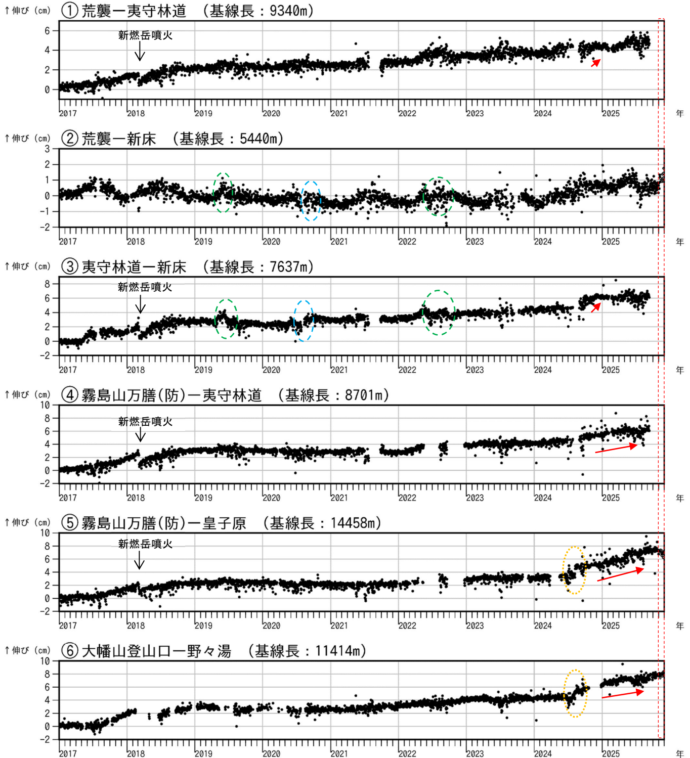
図5 霧島山（新燃岳） GNSS 連続観測による基線長変化（2017年1月～2025年11月）
