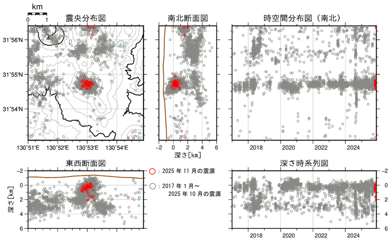
図 4 霧島山（新燃岳） 震源分布図（2017 年 1 月～2025 年 11 月）
