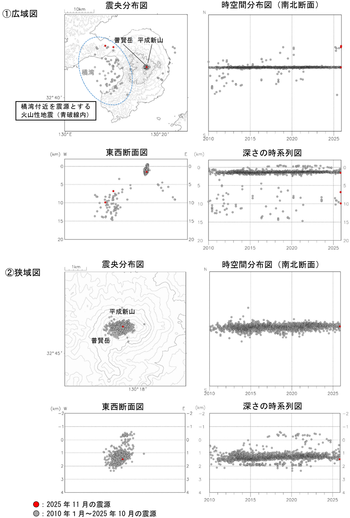
図5 雲仙岳 震源分布図 ①広域図 ②狭域図（2010年1月～2025年11月）
