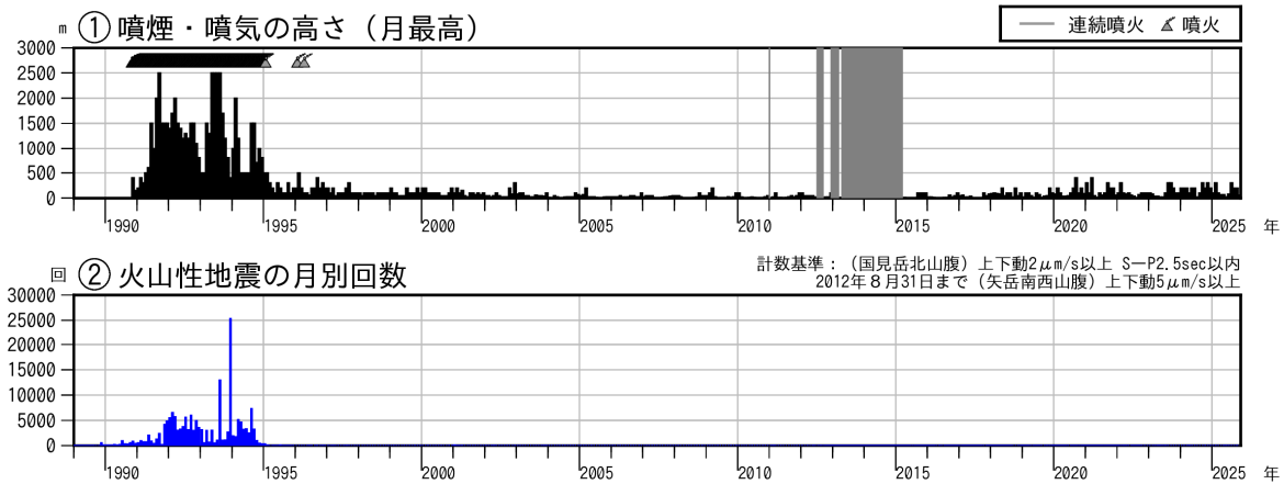
図3 雲仙岳 長期の火山活動経過図（1989年1月～2025年11月）
