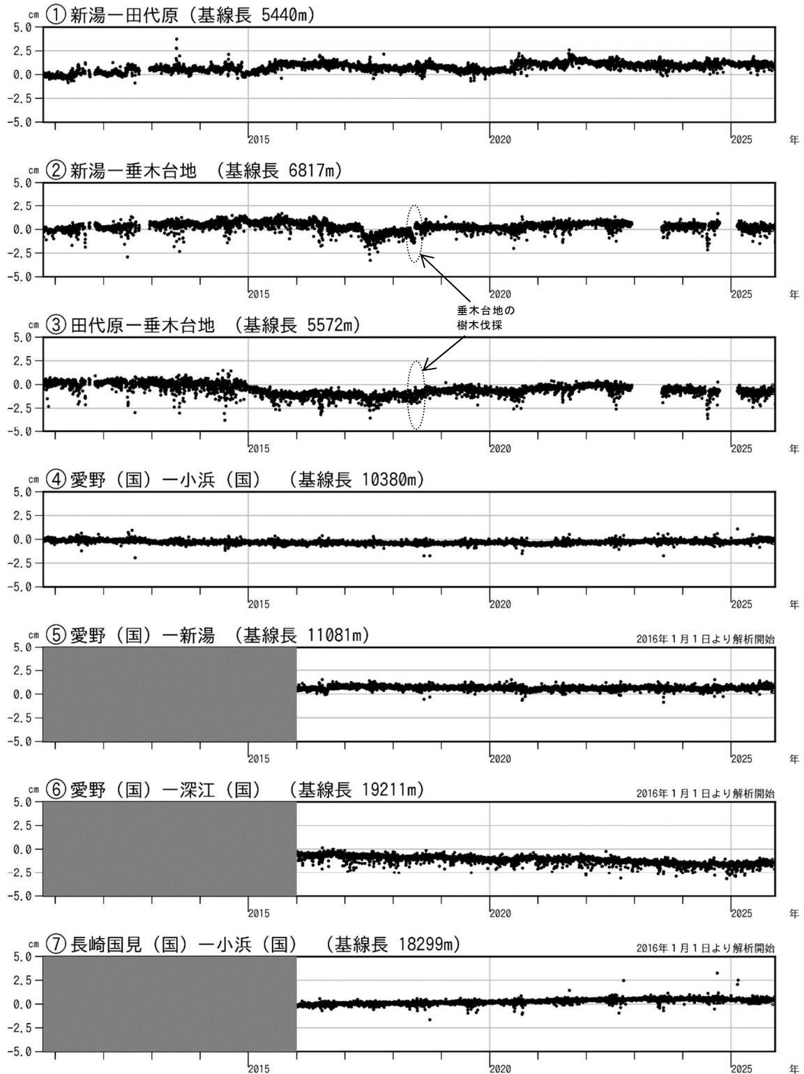
図6 雲仙岳 GNSS連続観測による基線長変化（2010年10月～2025年11月）
