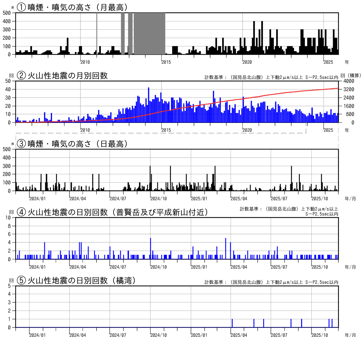
図4 雲仙岳 火山活動経過図（2006年1月～2025年11月）
