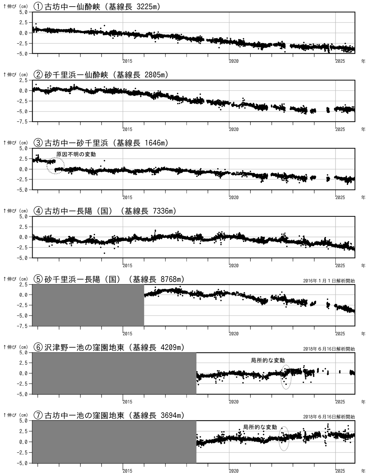
図5 阿蘇山 GNSS 連続観測による基線長変化 (2010年10月～2025年11月)
