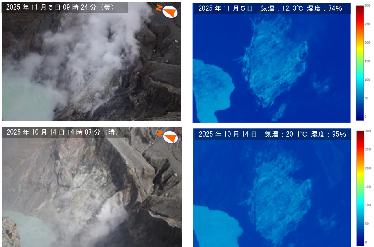
図 2-2 阿蘇山 中岳第一火口 南側火口壁の状況 （火口南西側観測定点から撮影 上図：11月5日、下図：10月14日）
