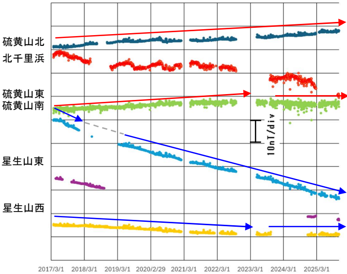
図 4-1 九重山 連続観測による全磁力の変化 (2017 年 3 月～2025 年 11 月)
