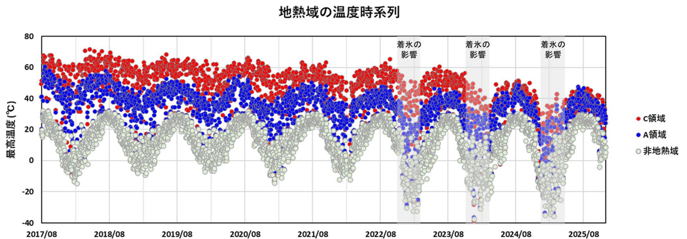
図 1-2 九重山 星生山北尾根の赤外熱映像装置による日別最高温度（2017 年 8 月～2025 年 11 月）
