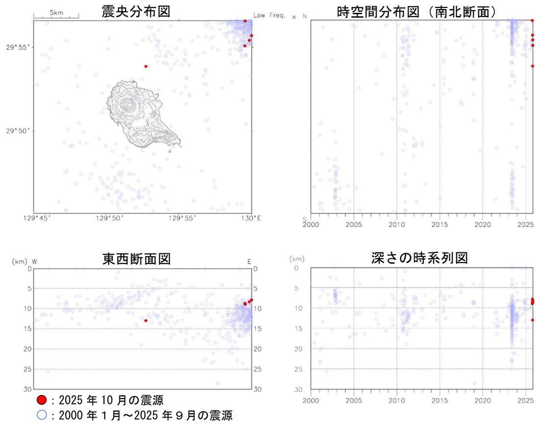
図3 中之島 中之島周辺の震源分布図（2000 年 1 月～2025 年 10 月）
