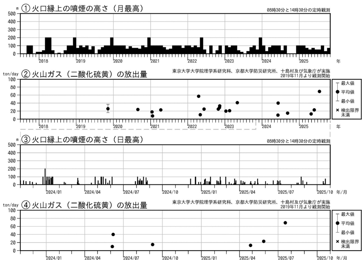
図2 中之島 火山活動経過図（2017年7月～2025年10月）
