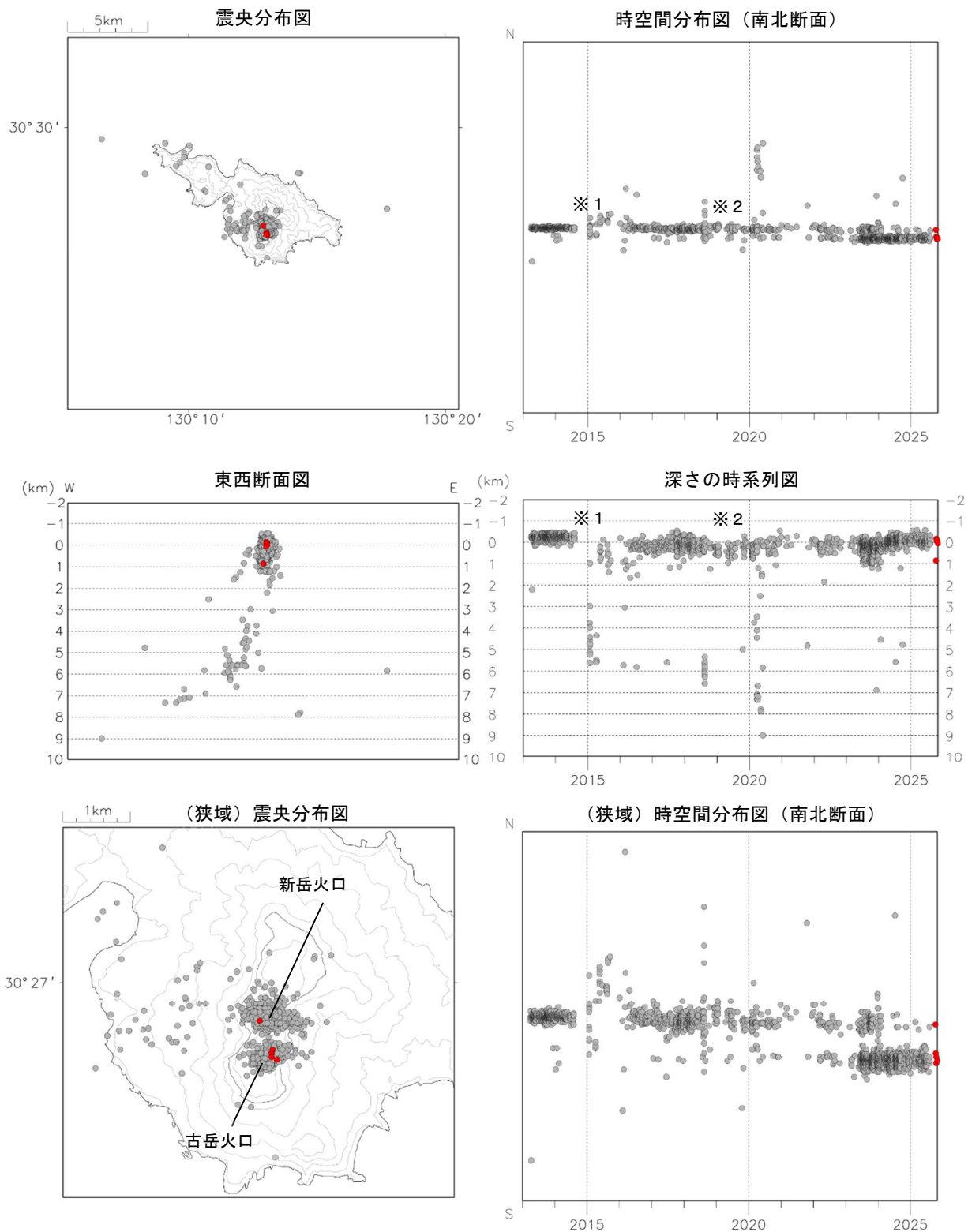
図5 口永良部島 震源分布図（2013年1月～2025年10月）
