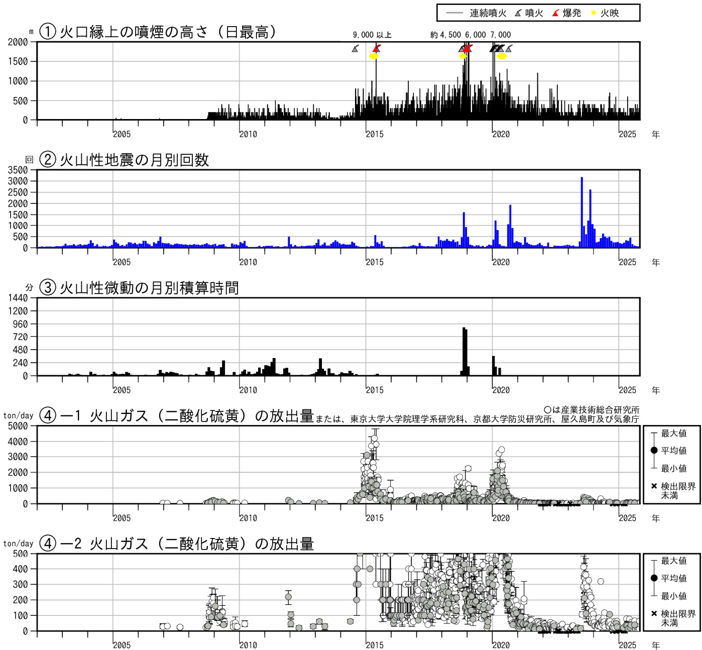
図3 口永良部島 火山活動経過図（2002年1月～2025年10月）
