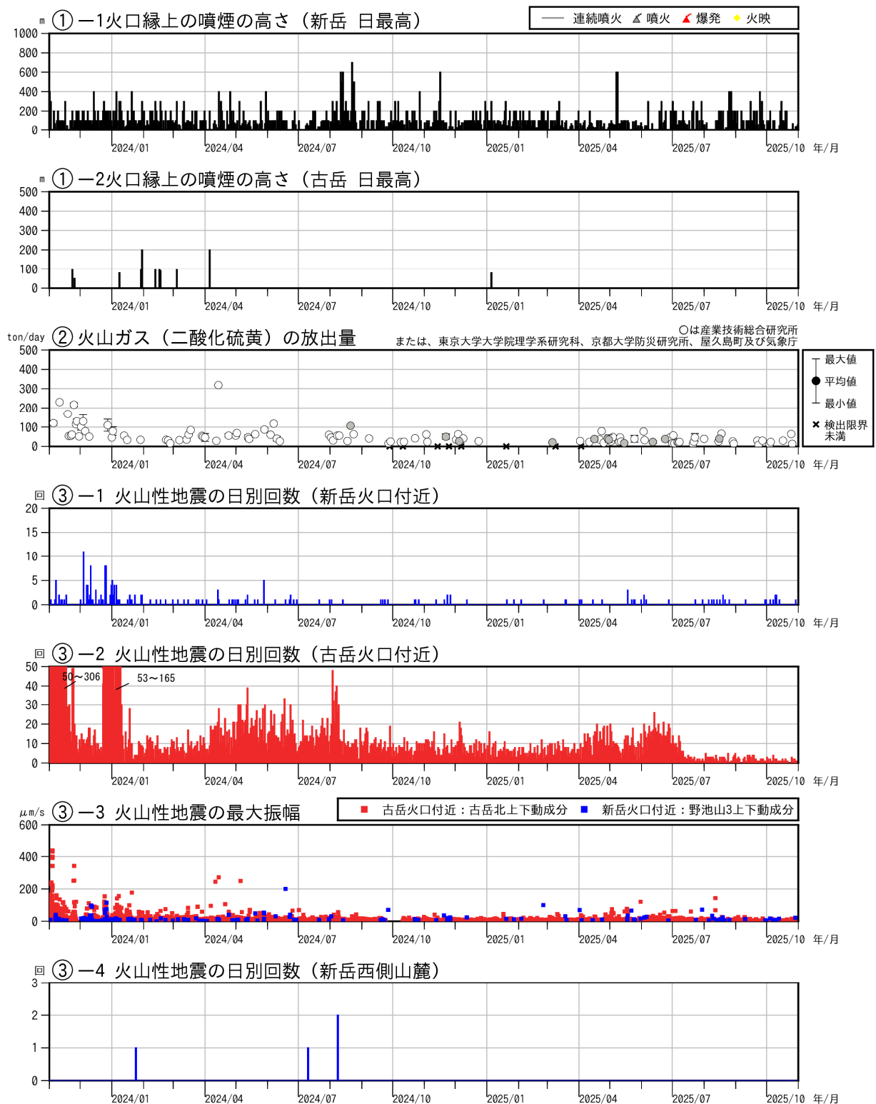
図4 口永良部島 最近の火山活動経過図（2023年11月～2025年10月）
