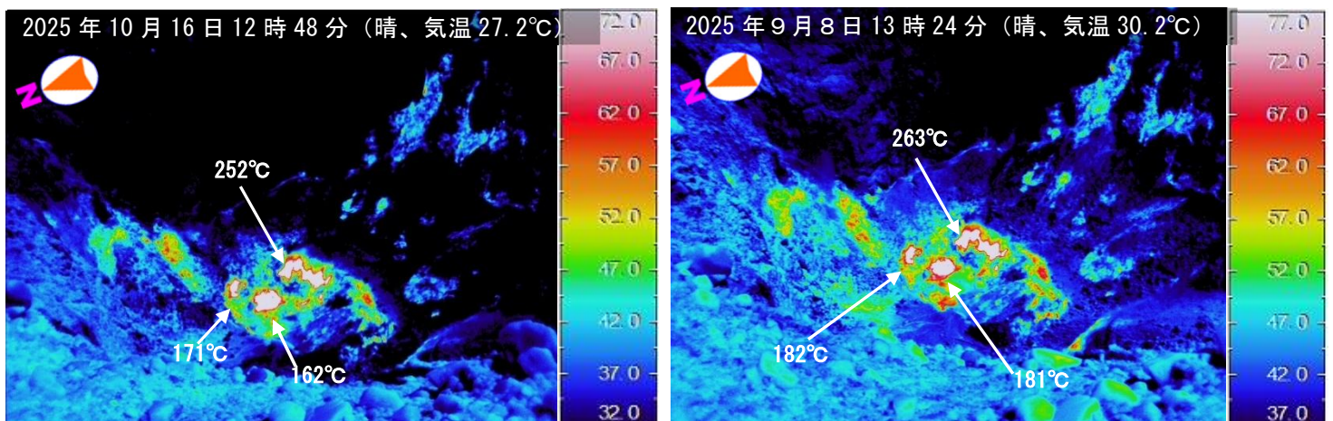
図 2-3 口永良部島 新岳火口内の状況（新岳火口縁北西側から撮影）
