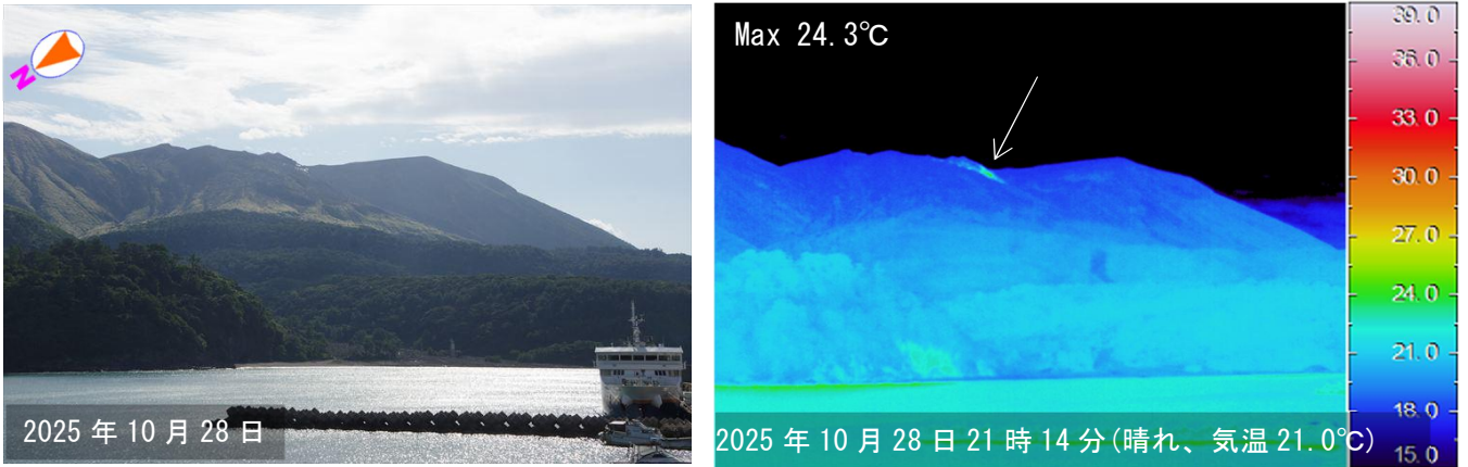
図 2-2 口永良部島 新岳火口及び新岳火口西側割れ目付近の状況（本村から観測）
