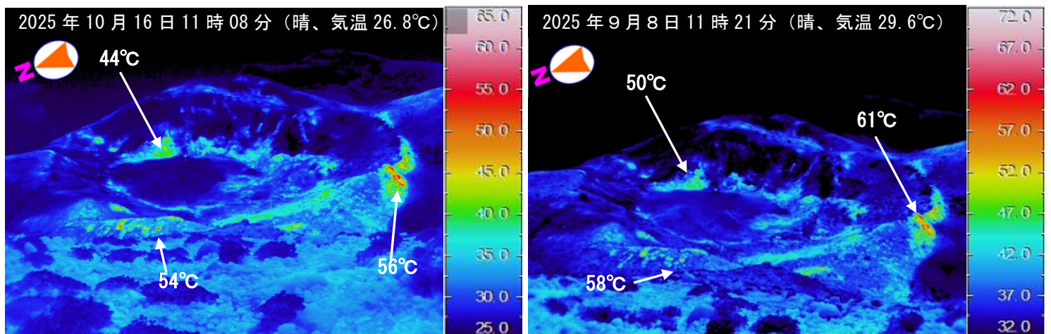
図 2-5 口永良部島 古岳火口内の状況（古岳山頂から撮影）
