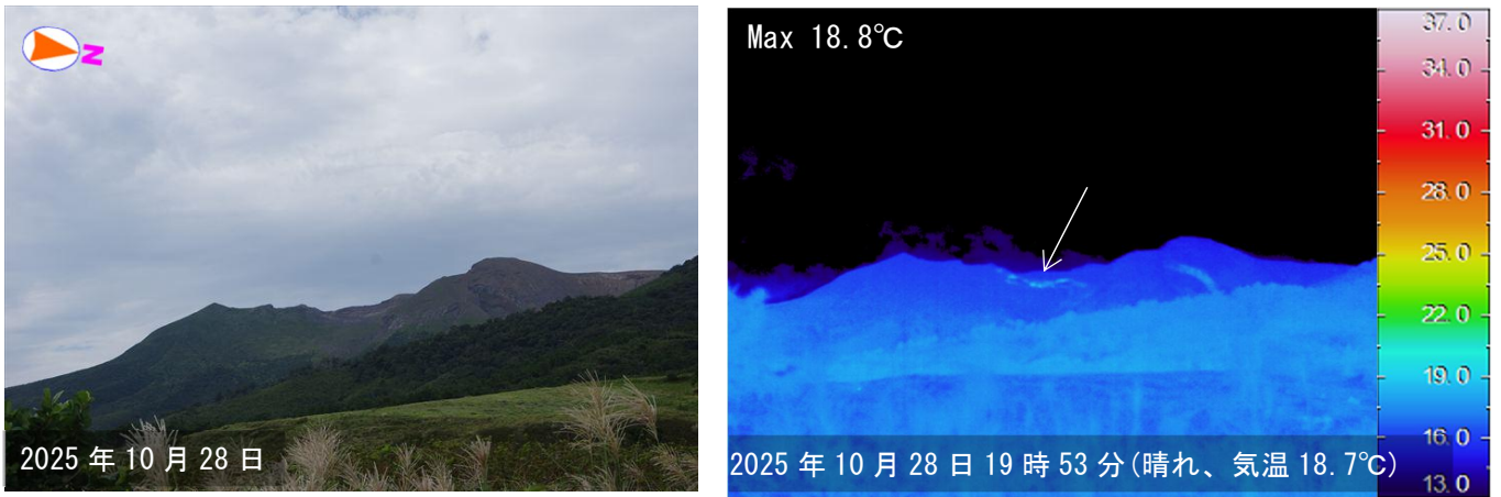
図 2-4 口永良部島 古岳周辺の地熱域の状況（湯向から観測）
