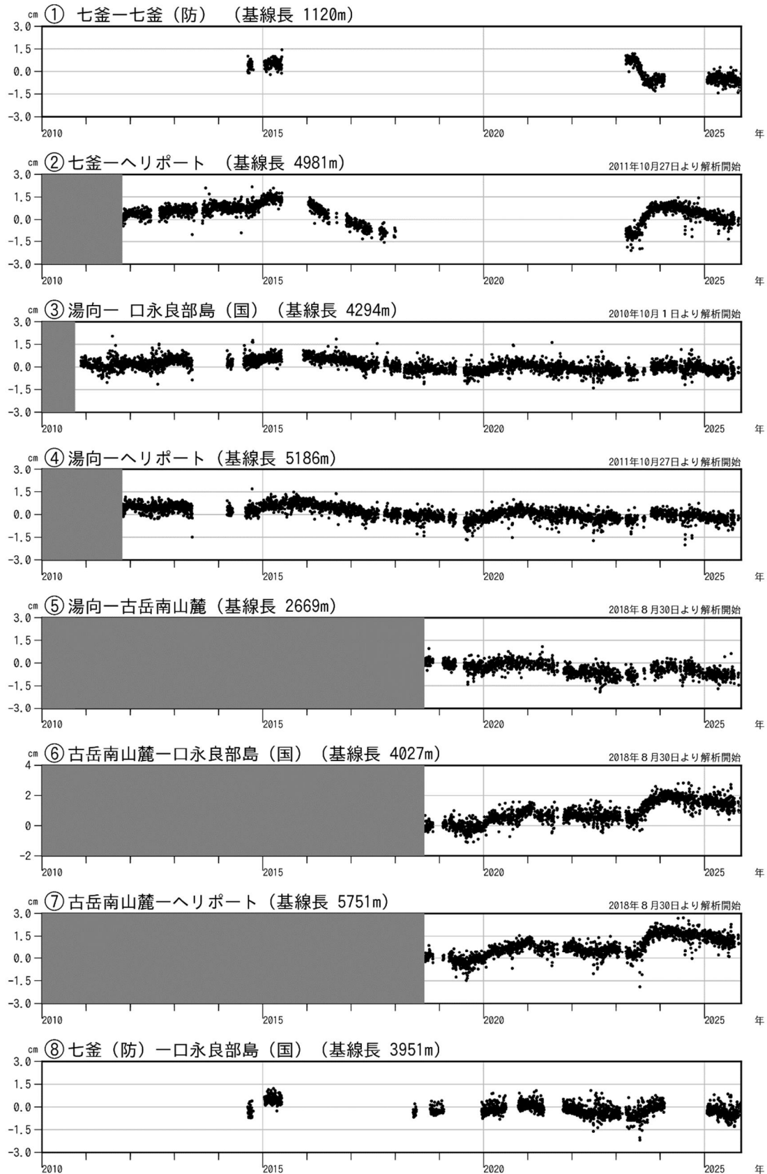
図6 口永良部島 GNSS 連続観測による基線長変化（2010年1月～2025年10月）
