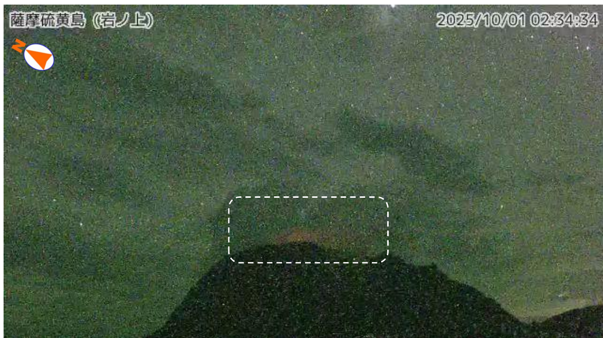
図 1-2 薩摩硫黄島 火映の状況（10 月 1 日、岩ノ上監視カメラ）
