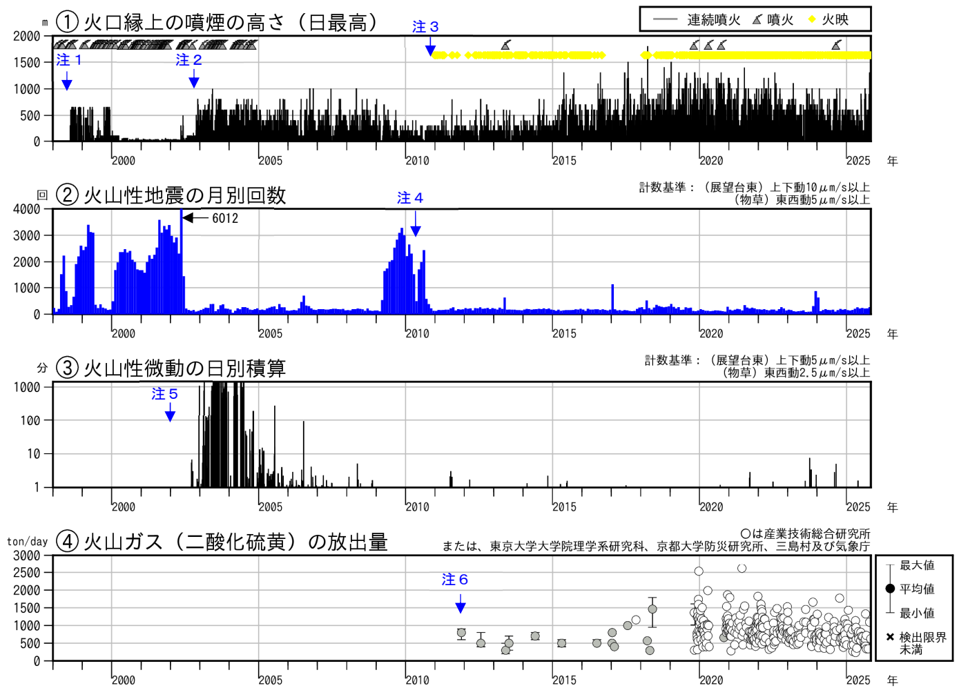
図2 薩摩硫黄島 火山活動経過図（1998年1月～2025年10月）
