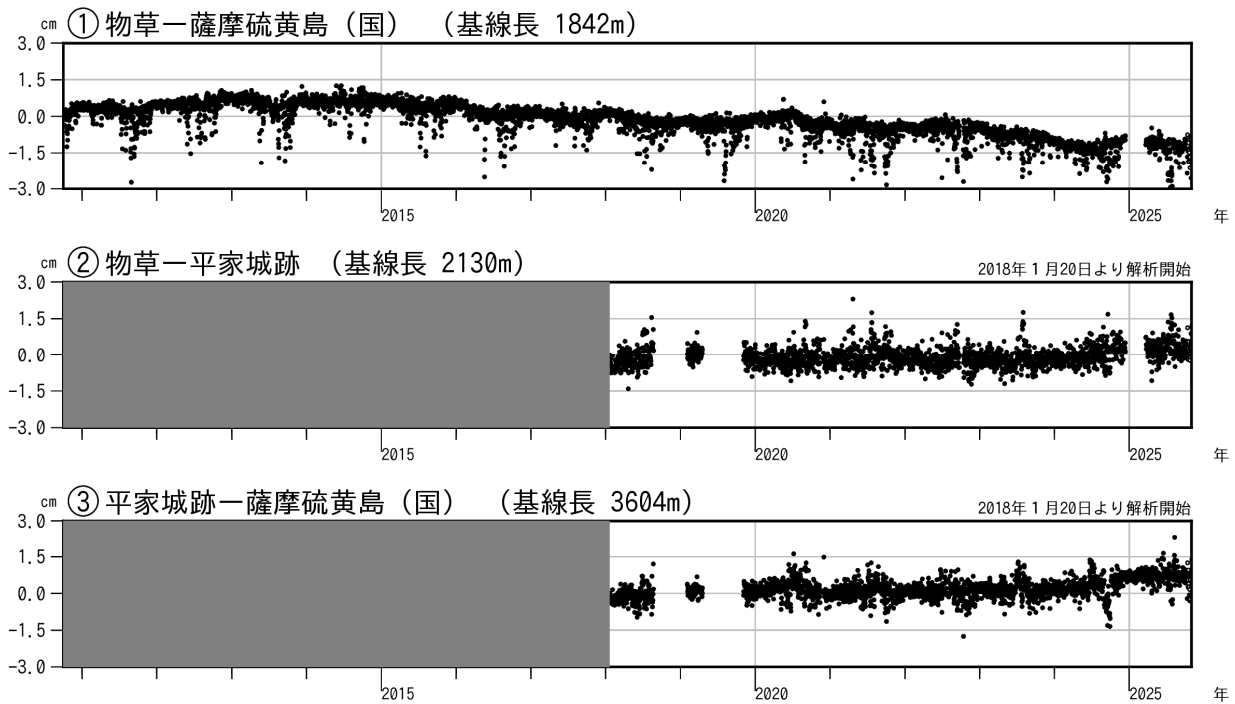
図5 薩摩硫黄島 GNSS連続観測による基線長変化 (2010年10月~2025年10月)
