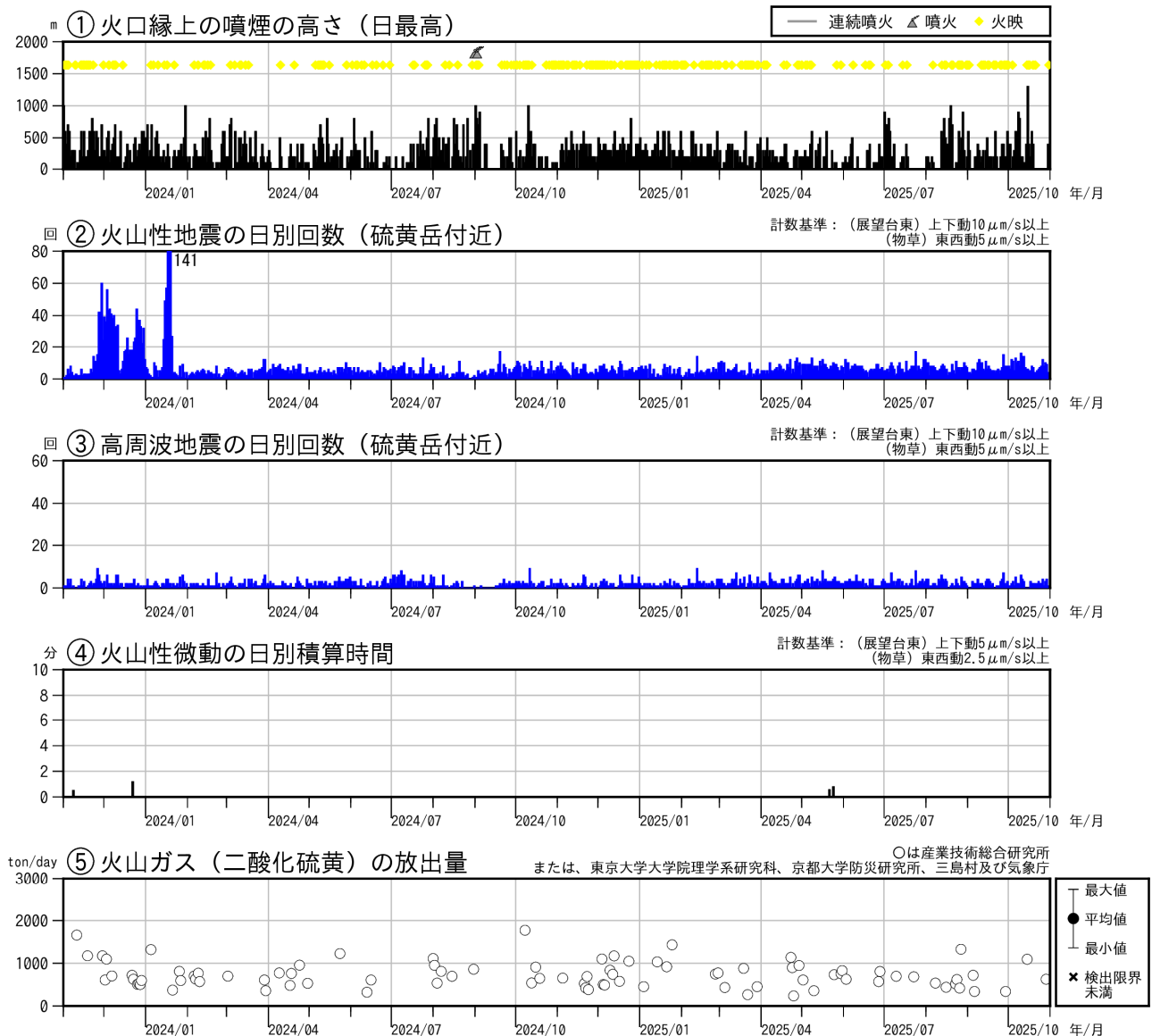
図3 薩摩硫黄島 火山活動経過図（2023年11月～2025年10月）
