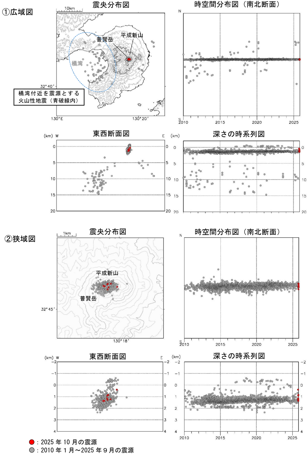
図4 雲仙岳 震源分布図 ①広域図 ②狭域図（2010年1月～2025年10月）
