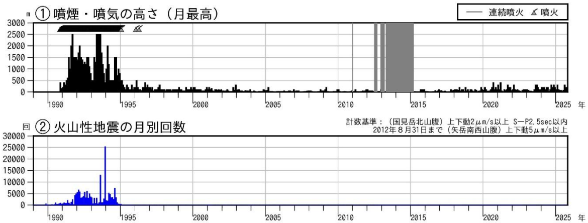
図2 雲仙岳 長期の火山活動経過図（1989年1月～2025年10月）
