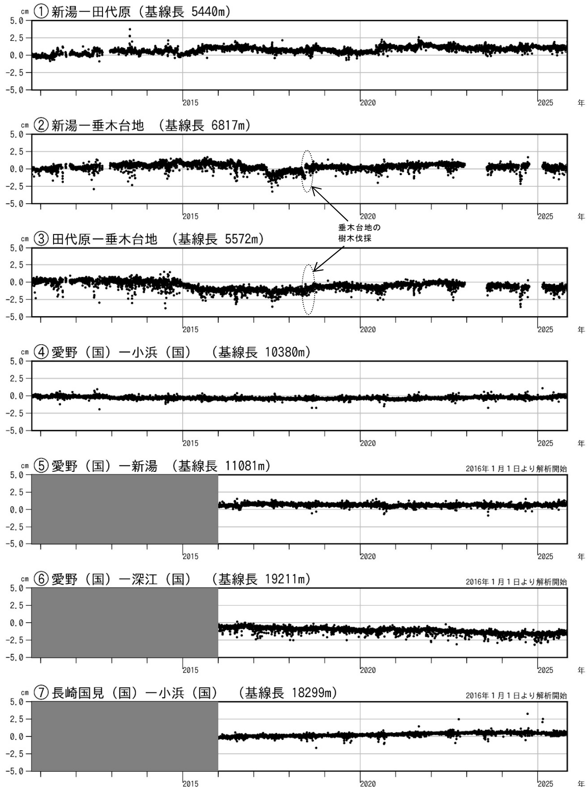
図5 雲仙岳 GNSS連続観測による基線長変化（2010年10月～2025年10月）
