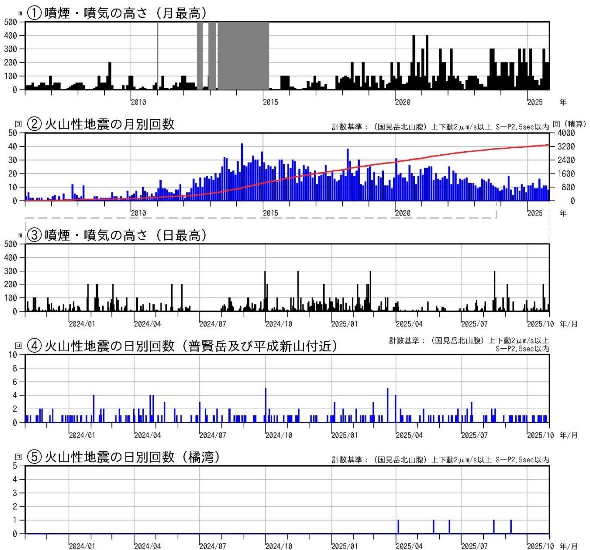
図3 雲仙岳 火山活動経過図（2006年1月～2025年10月）
