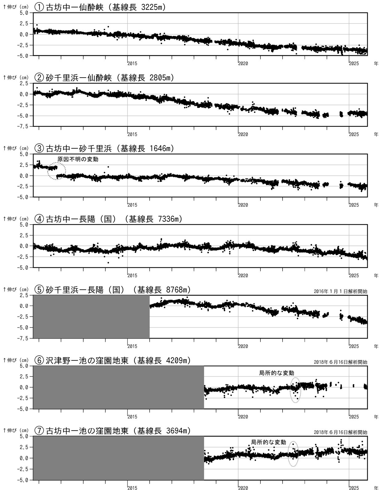
図5 阿蘇山 GNSS 連続観測による基線長変化（2010年10月～2025年10月）
