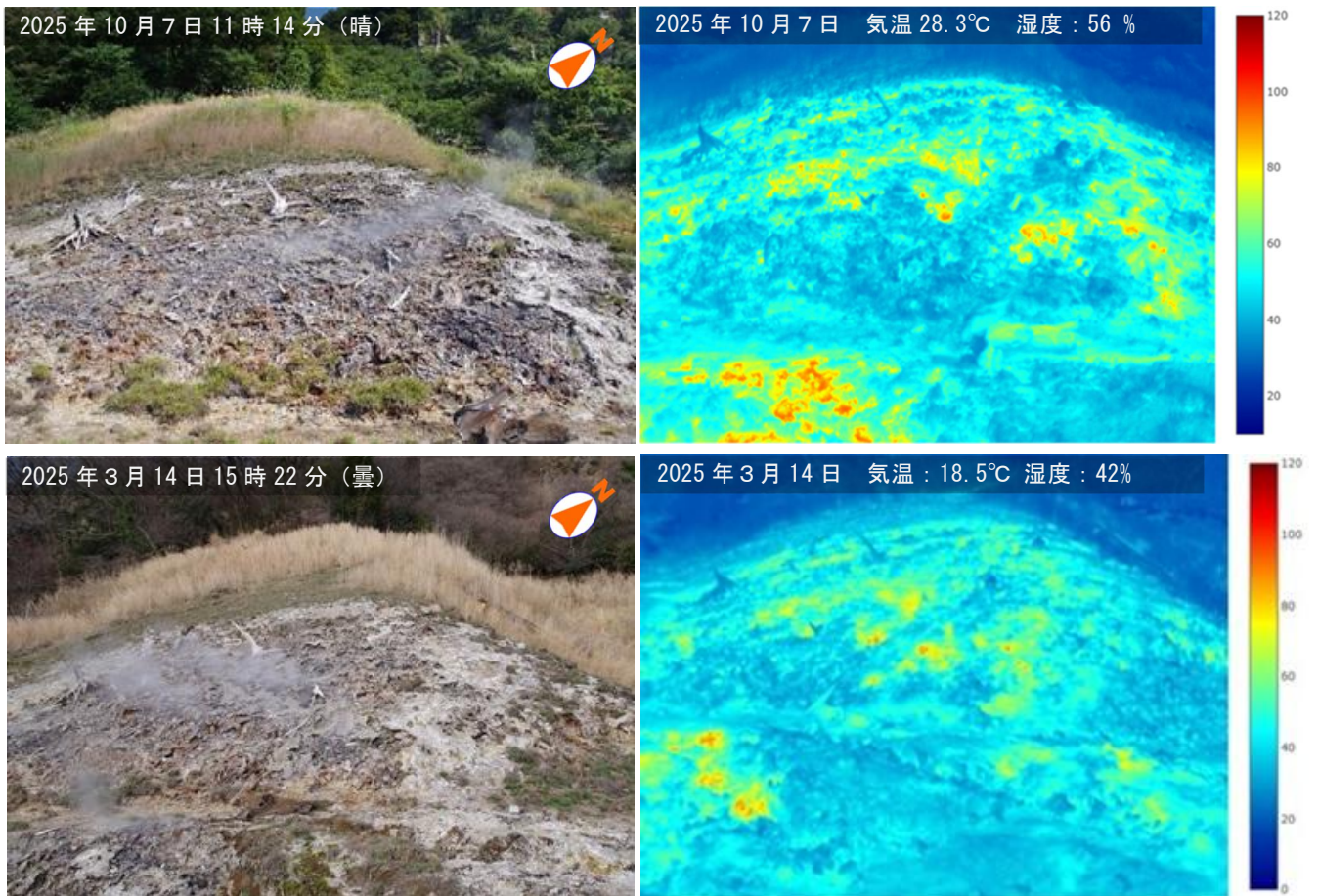
図 7-1 阿蘇山 南阿蘇村吉岡噴気地帯の状況（噴気地帯を南東側から撮影）
