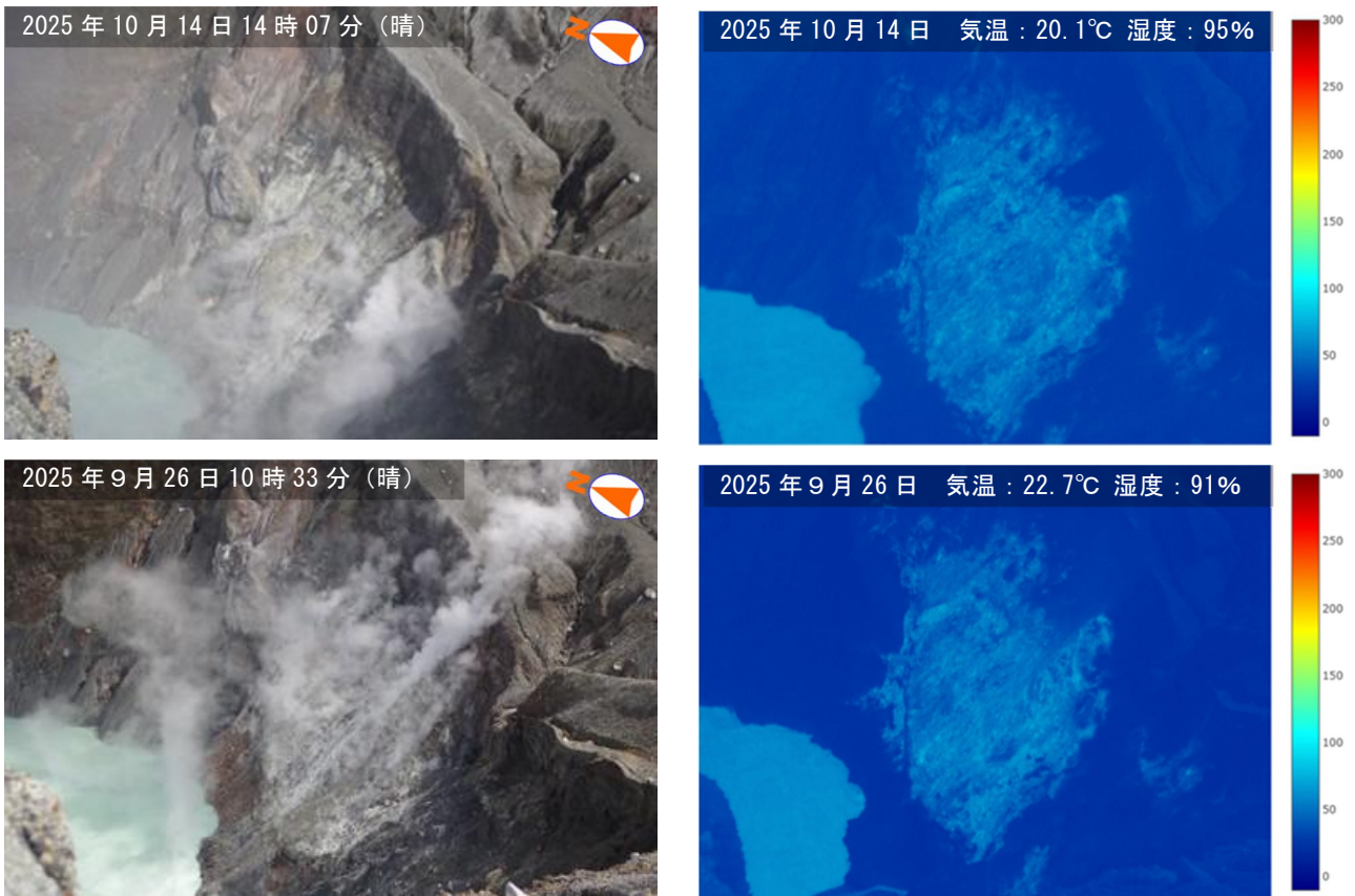
図 2-2 阿蘇山 中岳第一火口 南側火口壁の状況 (火口南西側観測定点から撮影 上図：10月14日、下図：9月26日)
