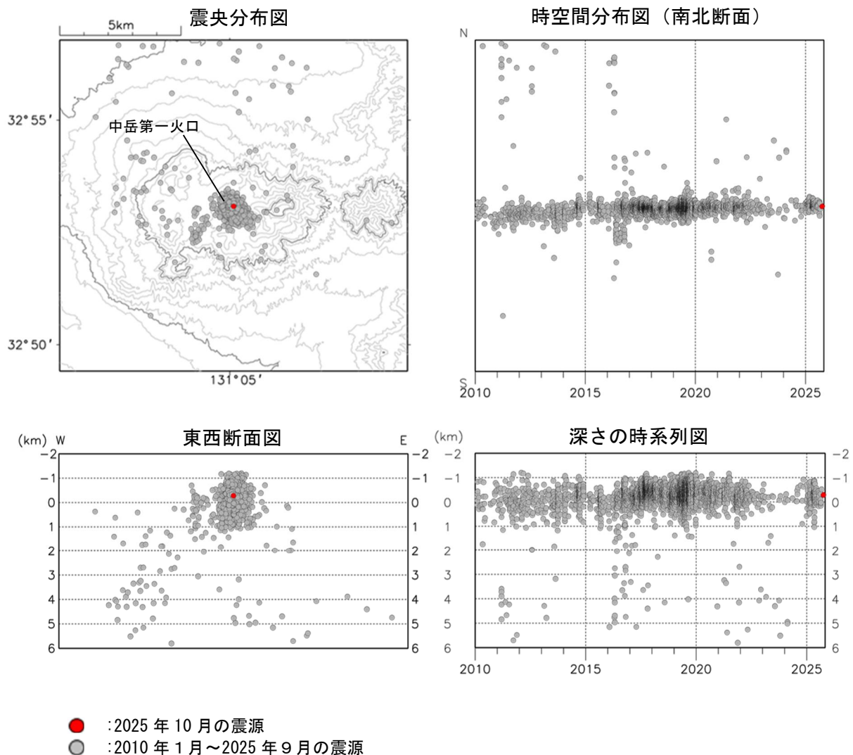
図4 阿蘇山 火山性地震の震源分布
