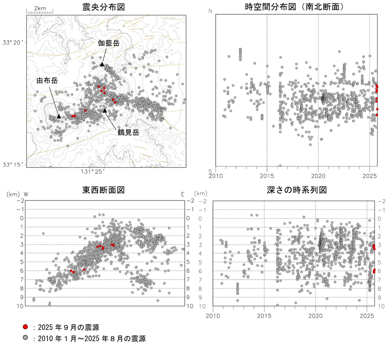
図 3 鶴見岳・伽藍岳 震源分布図（2010 年 1 月～2025 年 9 月）
