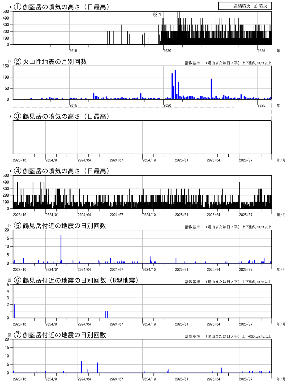
図2 鶴見岳・伽藍岳 火山活動経過図（2012年1月～2025年9月）
