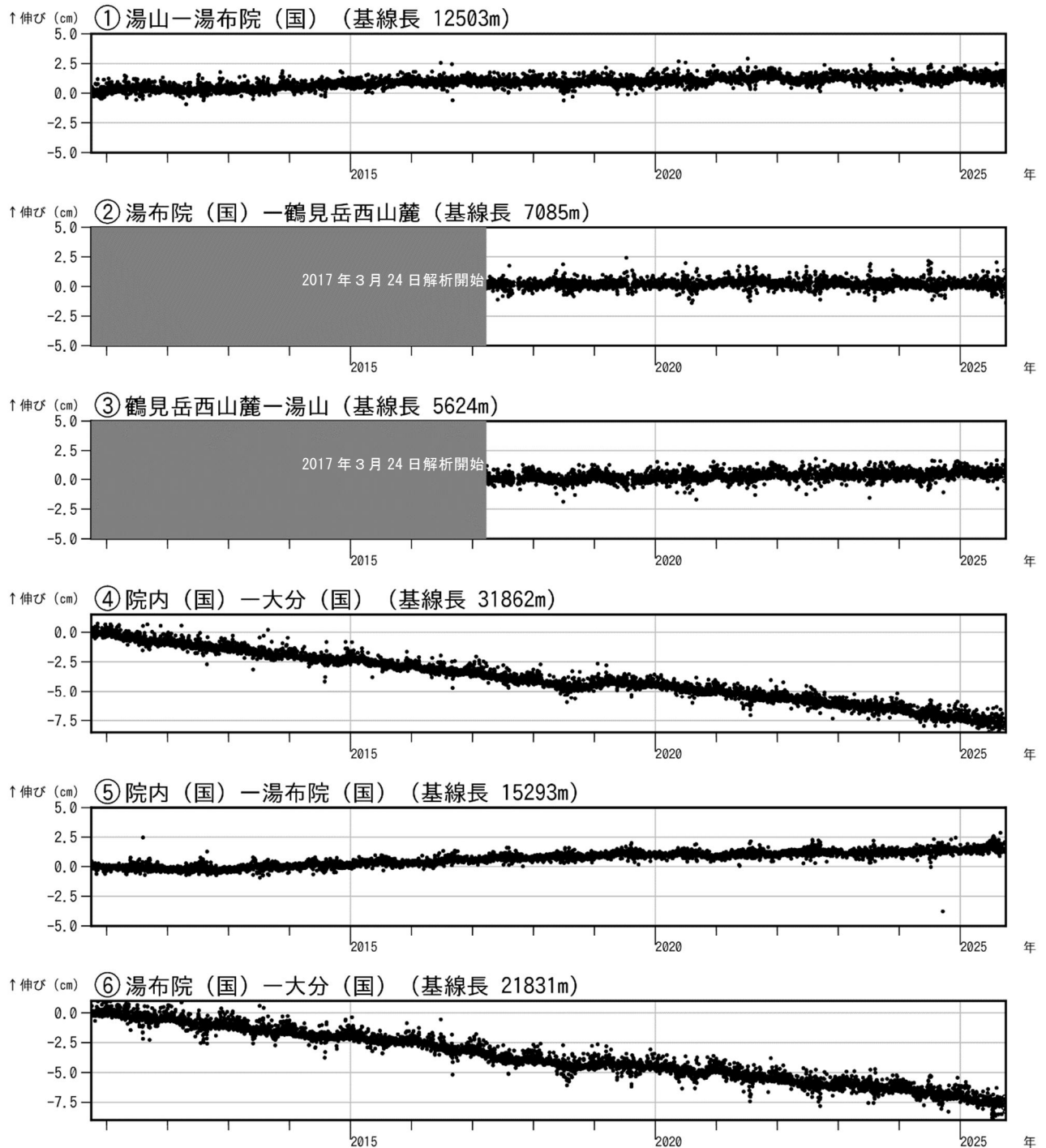
図4 鶴見岳・伽藍岳 GNSS連続観測による基線長変化（2010年10月～2025年9月）
