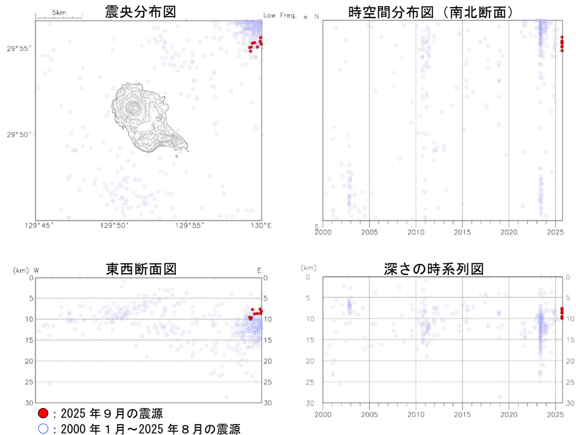
図3 中之島 中之島周辺の震源分布図（2000 年 1 月～2025 年 9 月）
