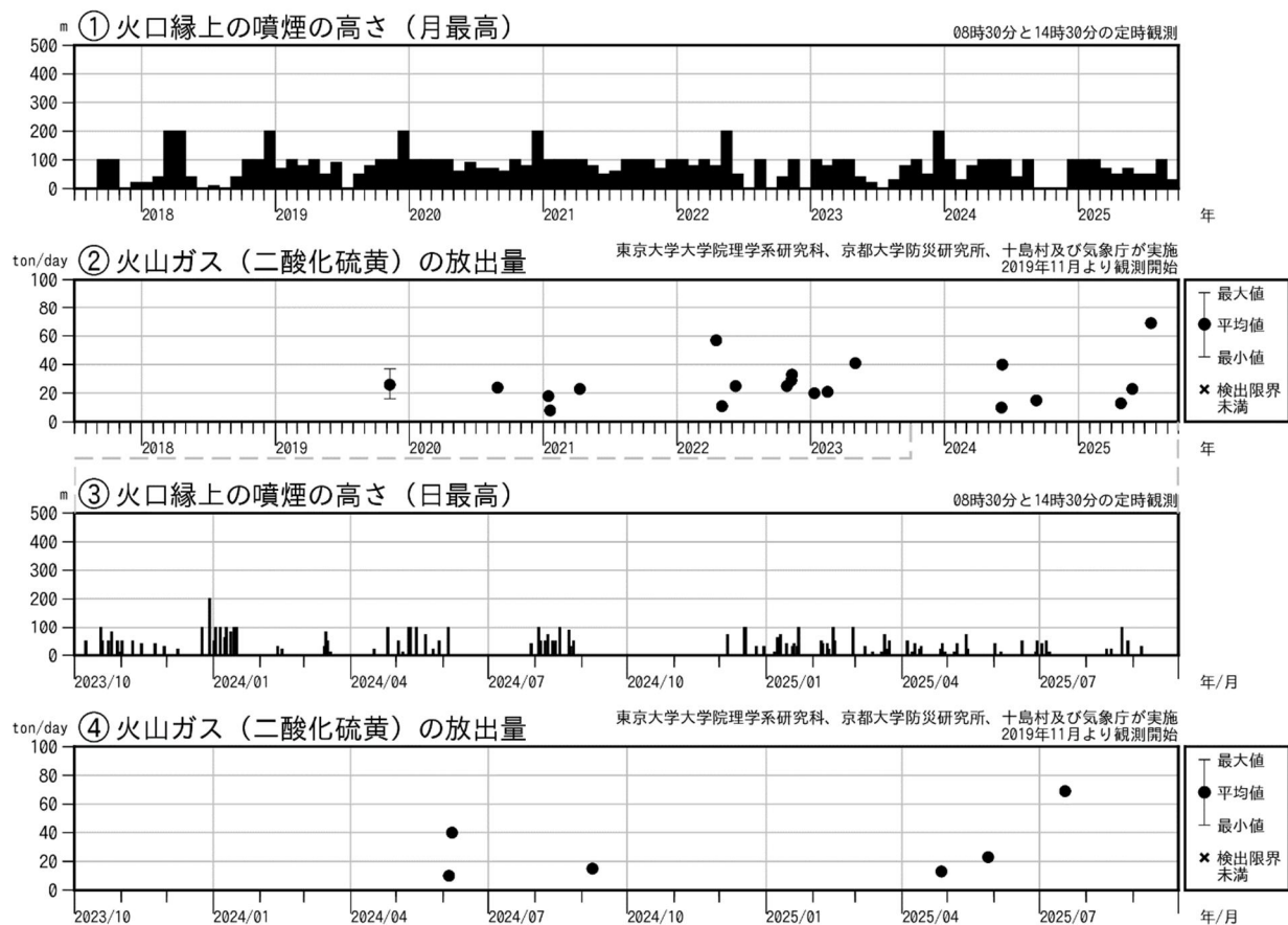
図 2 中之島 火山活動経過図（2017 年 7 月～2025 年 9 月）
