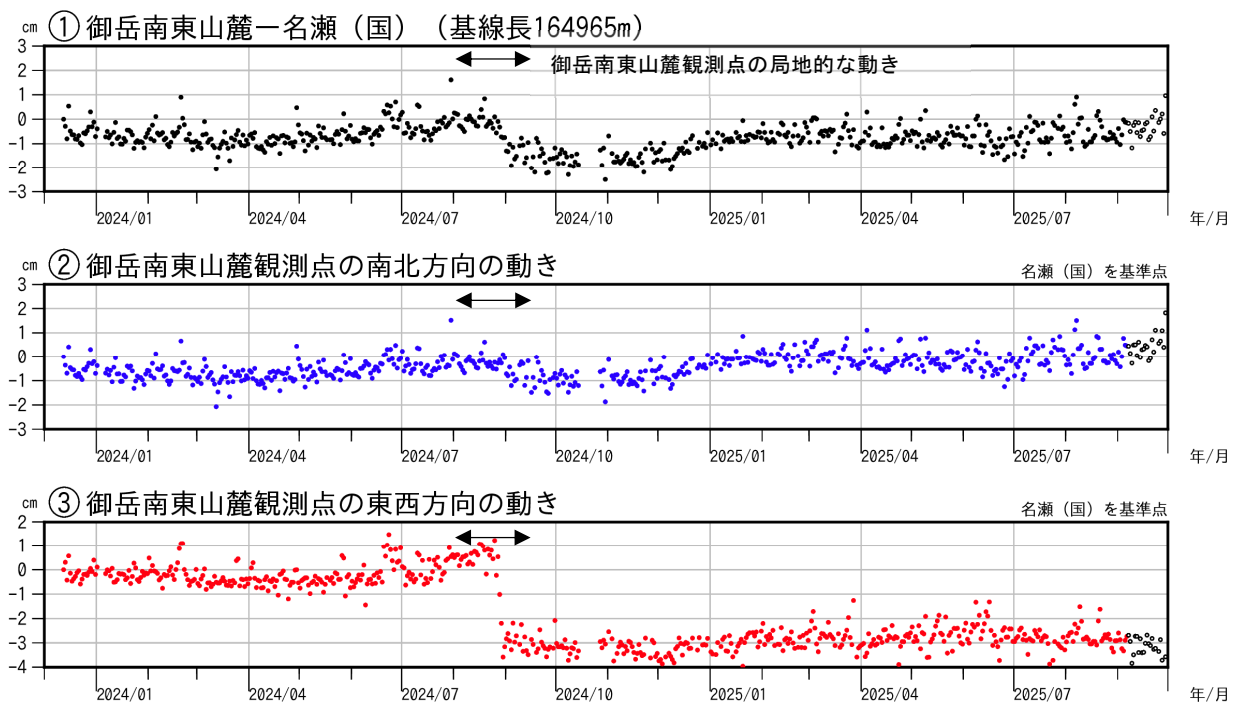
図4 中之島 GNSS連続観測（2023 年 12 月～2025 年 9 月）
