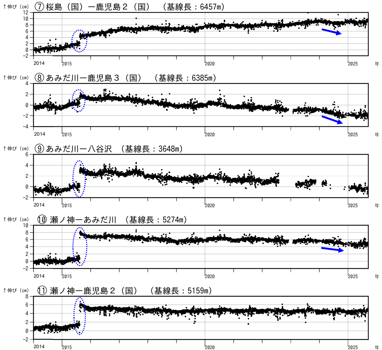
図 7-2 桜島 GNSS 連続観測による基線長変化（2014 年 1 月～2025 年 9 月）
