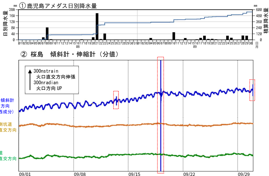
図6 桜島 傾斜計及び伸縮計による地殻変動の状況（2025年9月1日～9月30日）
