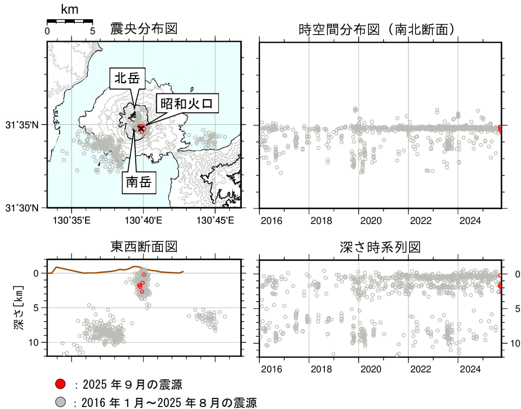
図 2-2 桜島 桜島付近の震源分布図（2016 年 1 月～2025 年 9 月）
