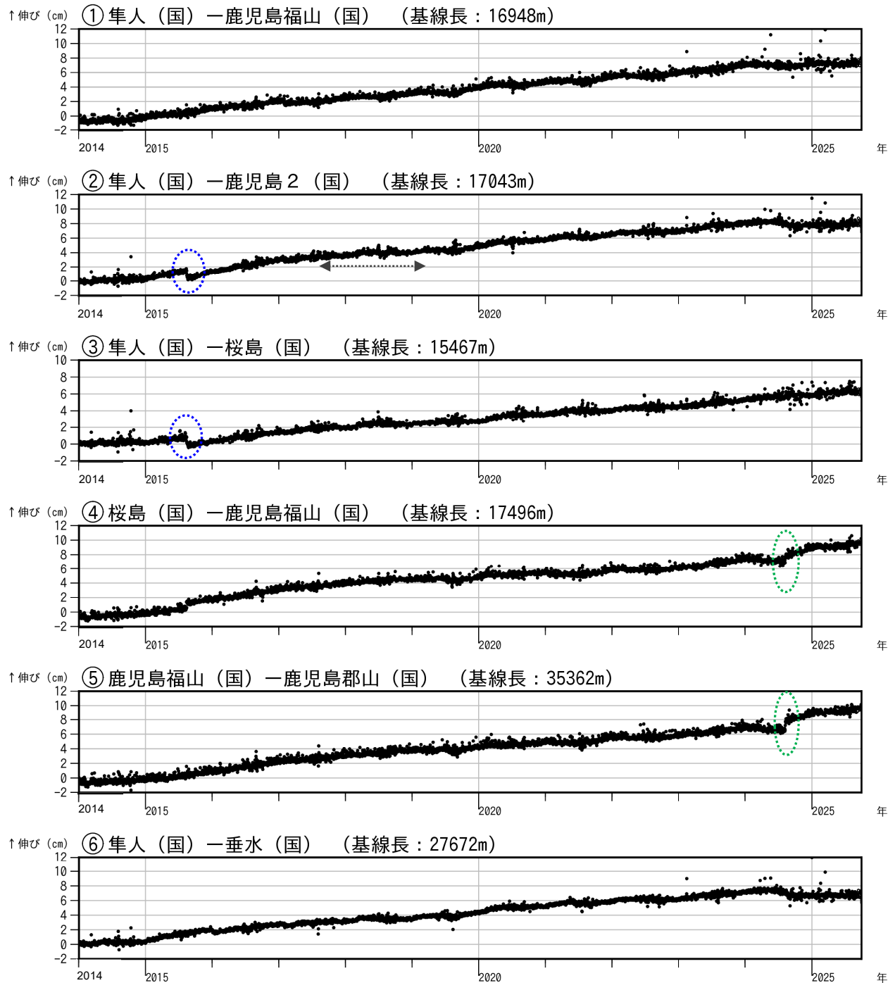
図 7-1 桜島 GNSS 連続観測による基線長変化 (2014 年 1 月～2025 年 9 月)
