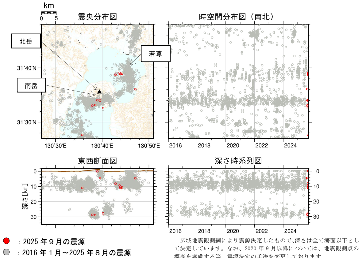
図 2-1 桜島 始良カルデラ周辺の震源分布図（2016 年 1 月～2025 年 9 月）
