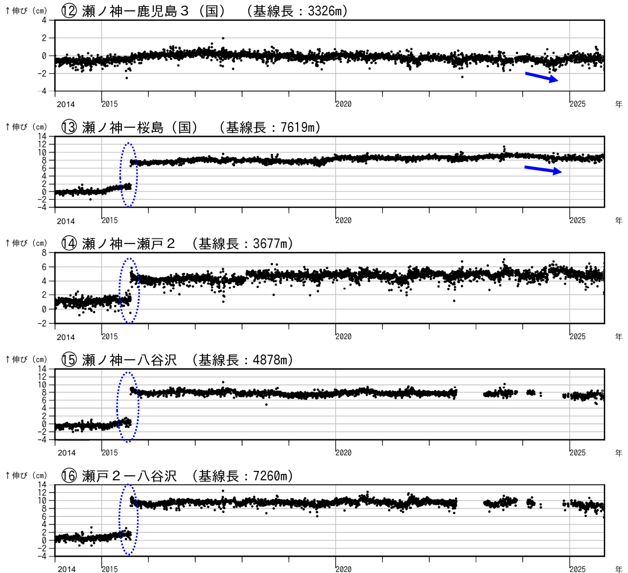
図 7-3 桜島 GNSS 連続観測による基線長変化（2014 年 1 月～2025 年 9 月）
