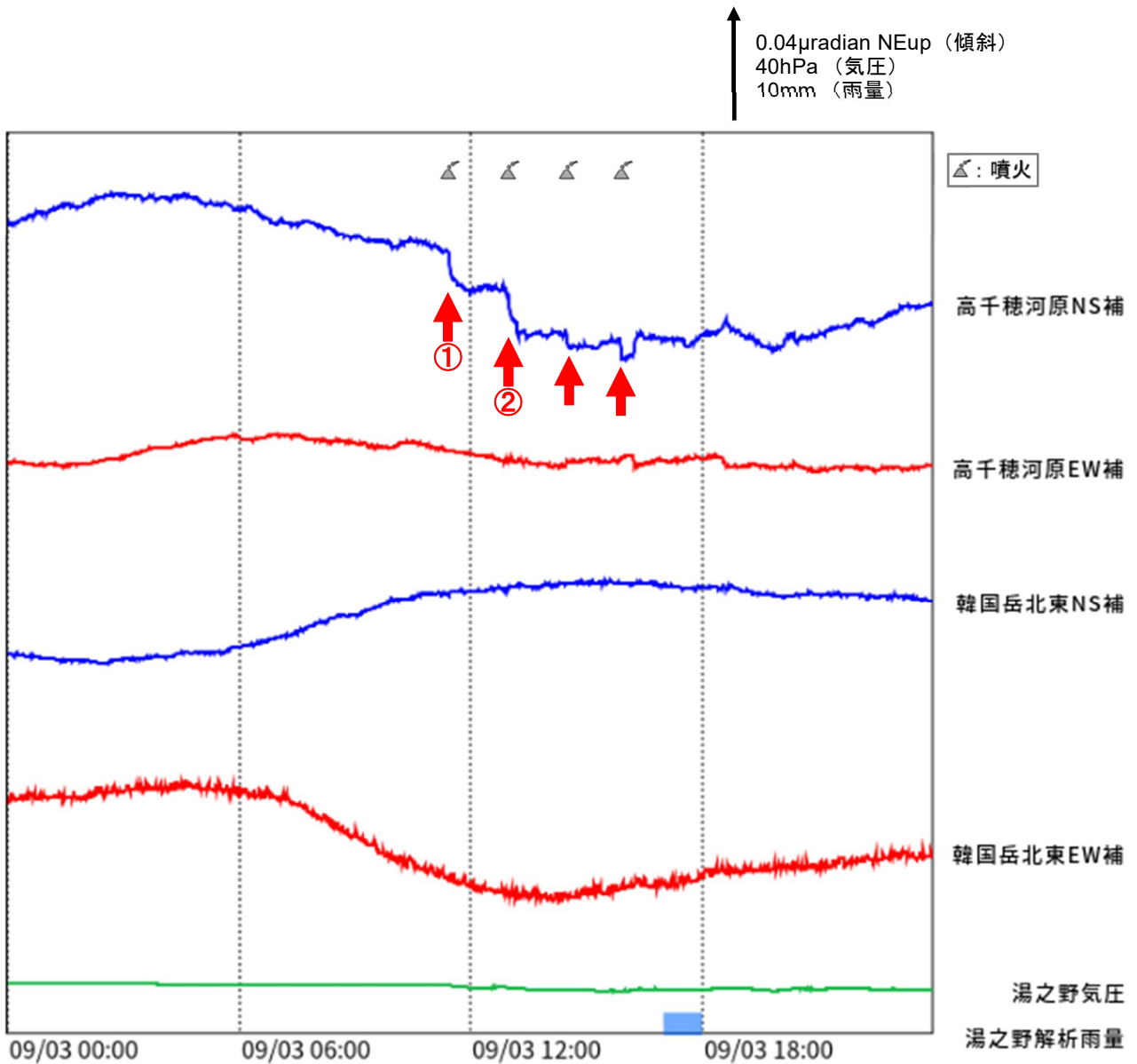
図6 霧島山（新燃岳） 傾斜計による地殻変動の状況（分値）（9月3日00時～4日00時）
