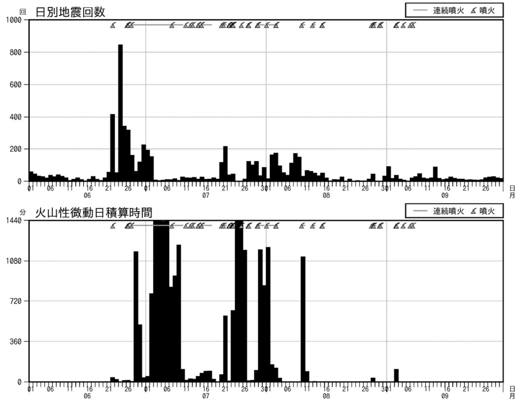
図3 霧島山（新燃岳） 火山性地震の日別回数（上段）及び火山性微動の日積算時間（下段） （2025年6月1日～9月30日）
