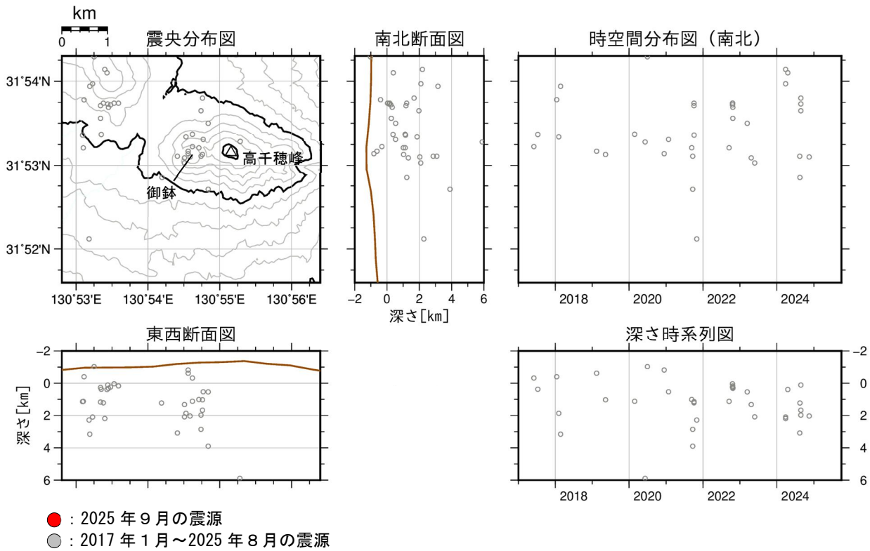
図2 霧島山（御鉢） 震源分布図（2017年1月～2025年9月）
