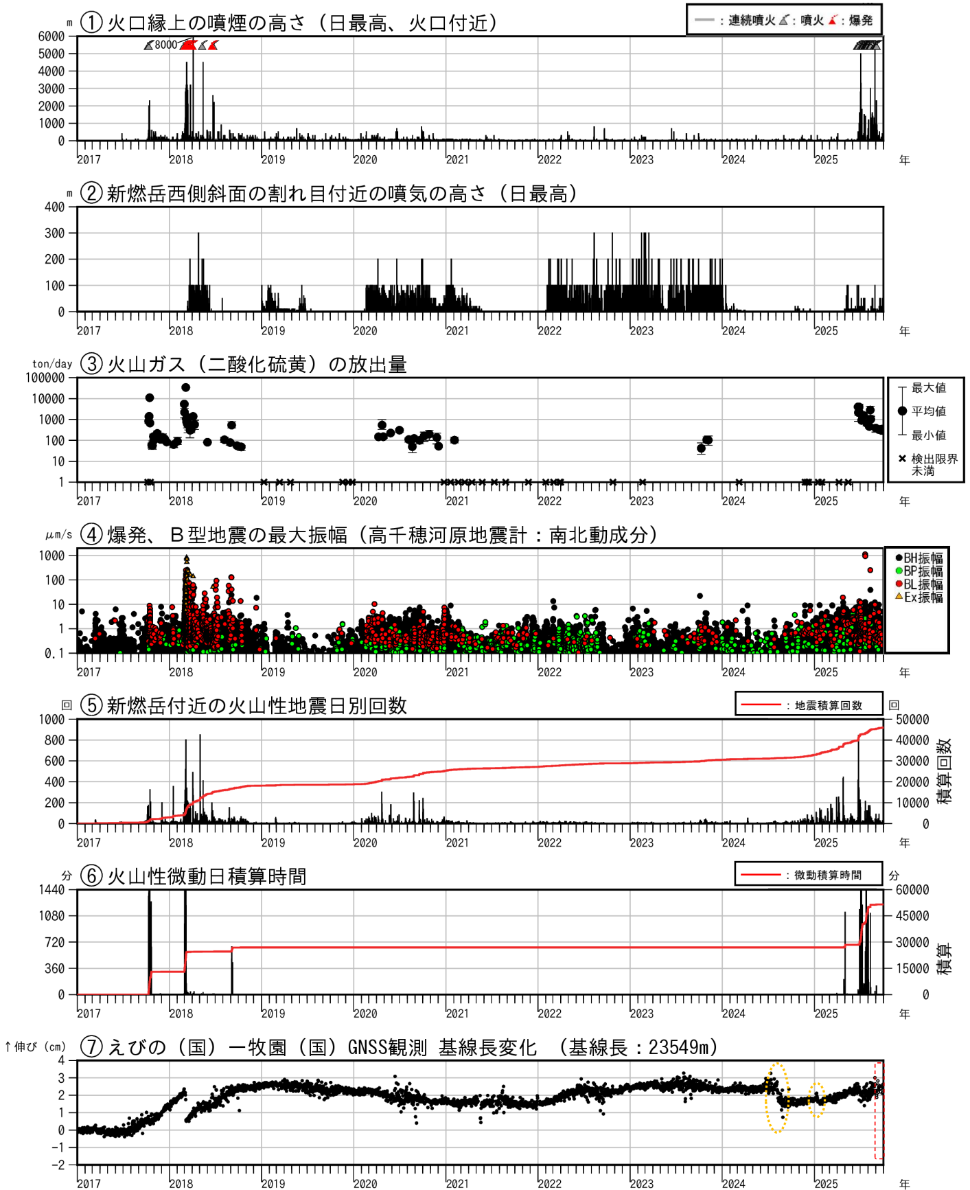
図 4-1 霧島山（新燃岳） 火山活動経過図（2017 年 1 月～2025 年 9 月）
