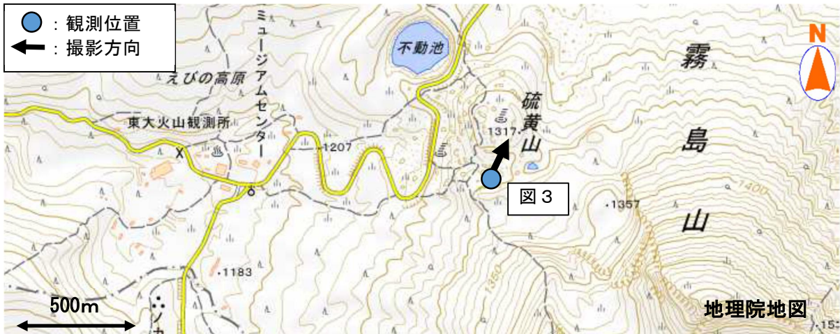
図2 霧島山（えびの高原（硫黄山）周辺）図3の観測位置及び撮影方向
