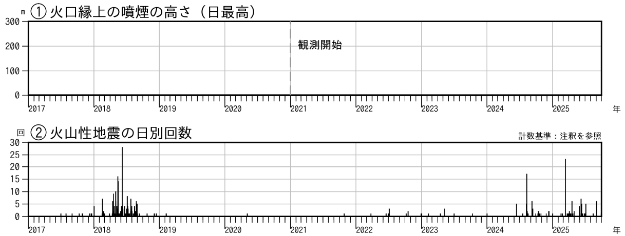
図2 霧島山（大幡池） 火山活動経過図（2017年1月～2025年9月）
