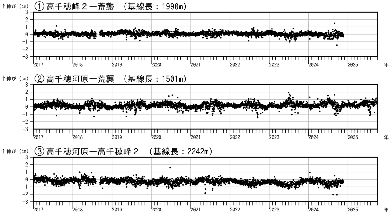
図4 霧島山（御鉢） GNSS 連続観測による基線長変化（2017年1月～2025年9月）
