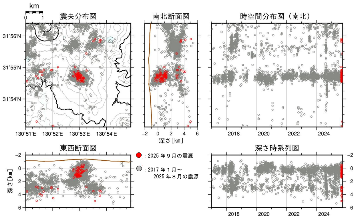
図 5 霧島山（新燃岳） 震源分布図（2017 年 1 月～2025 年 9 月）
