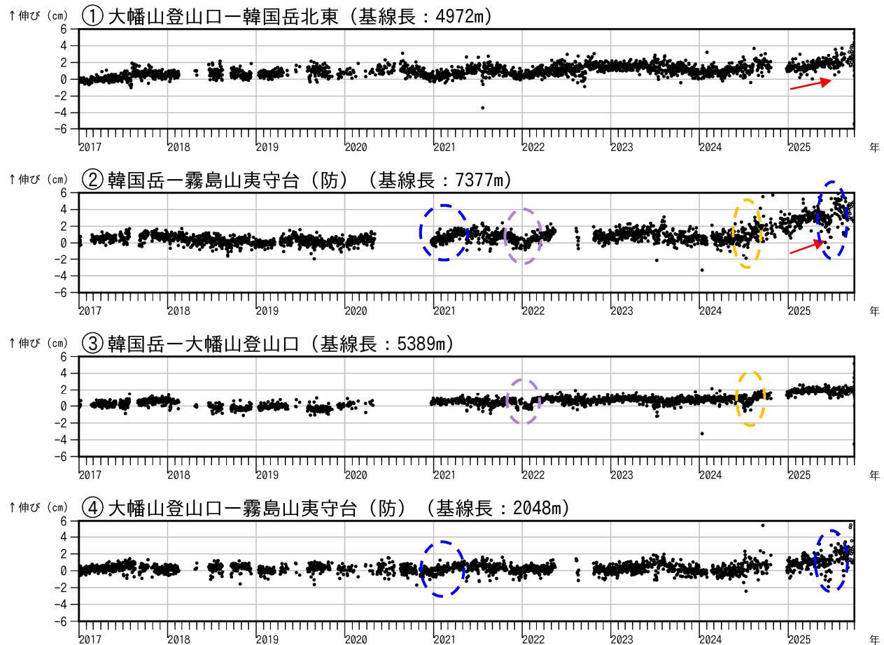
図4 霧島山（大幡池） GNSS 連続観測による基線長変化（2017年1月～2025年9月）
