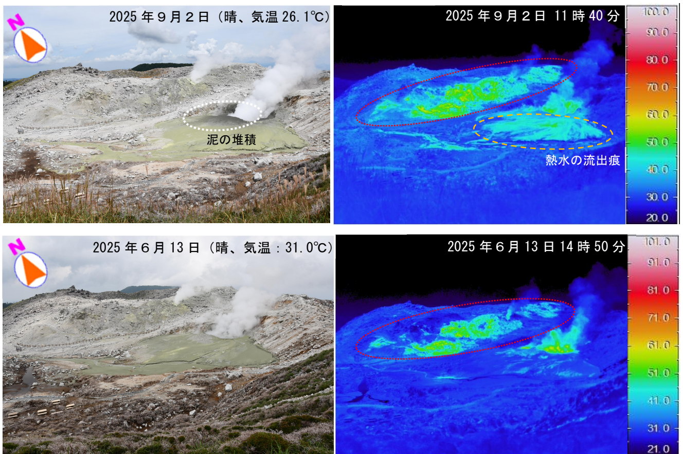
図3 霧島山（えびの高原（硫黄山）周辺）硫黄山の南側の噴気及び地熱域等の状況
