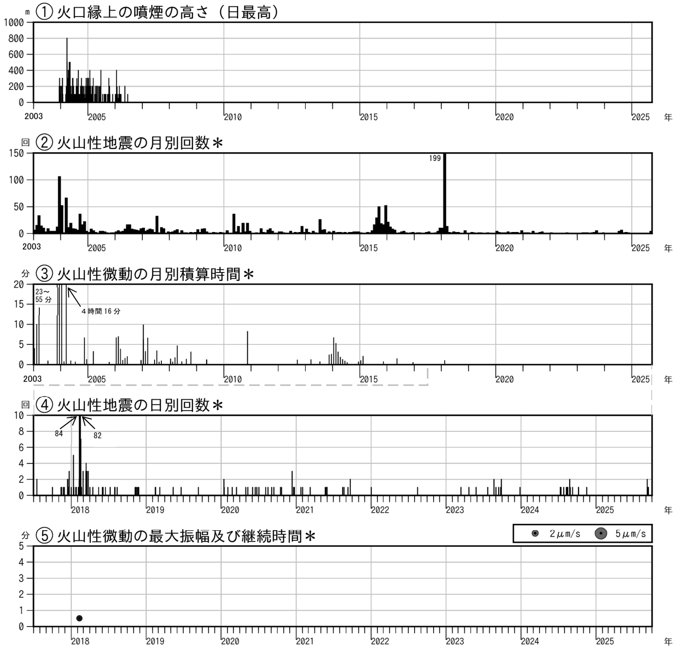
図3 霧島山（御鉢） 火山活動経過図（2003年1月～2025年9月）
