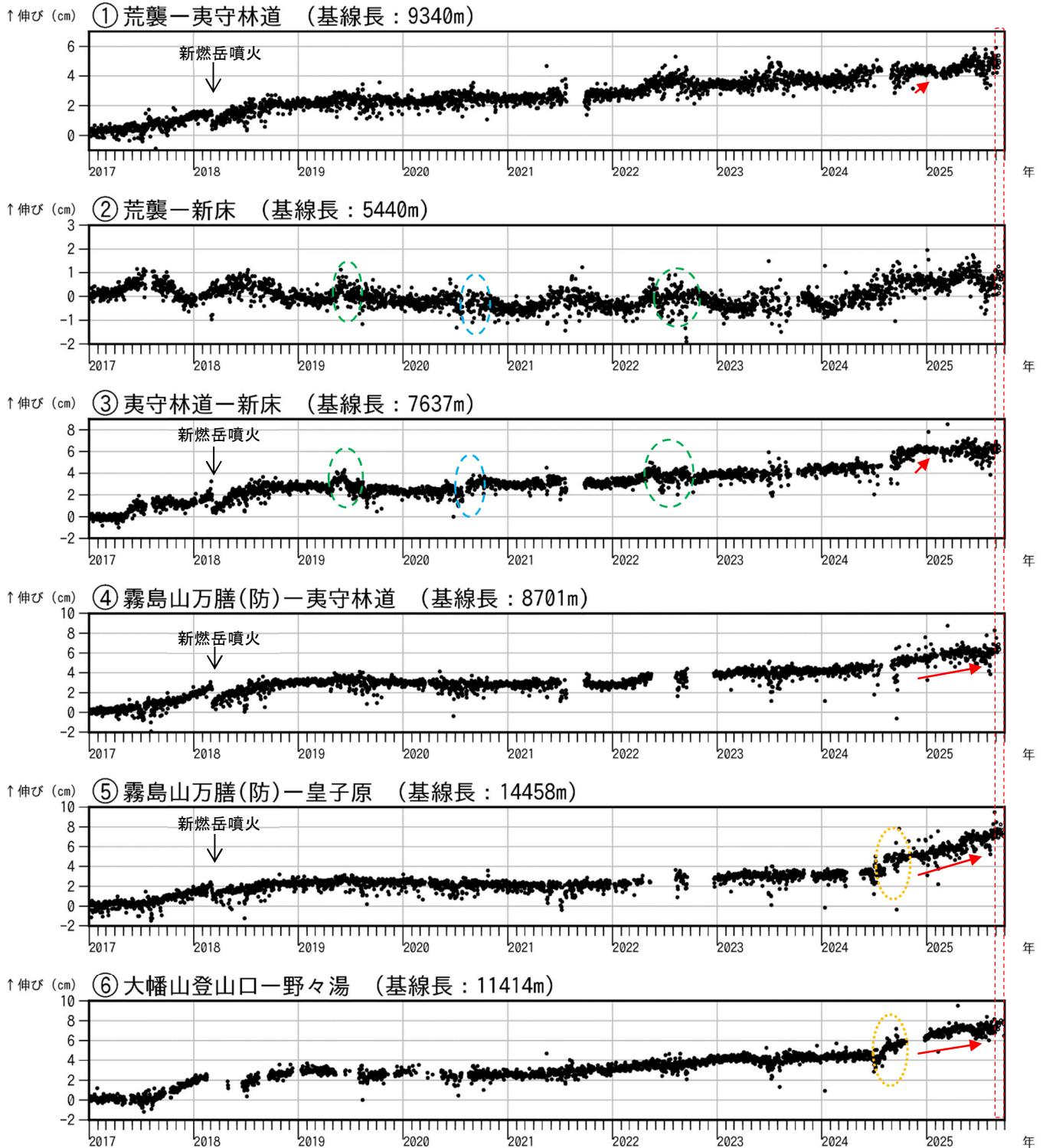
図7 霧島山（新燃岳） GNSS 連続観測による基線長変化（2017年1月～2025年9月）
