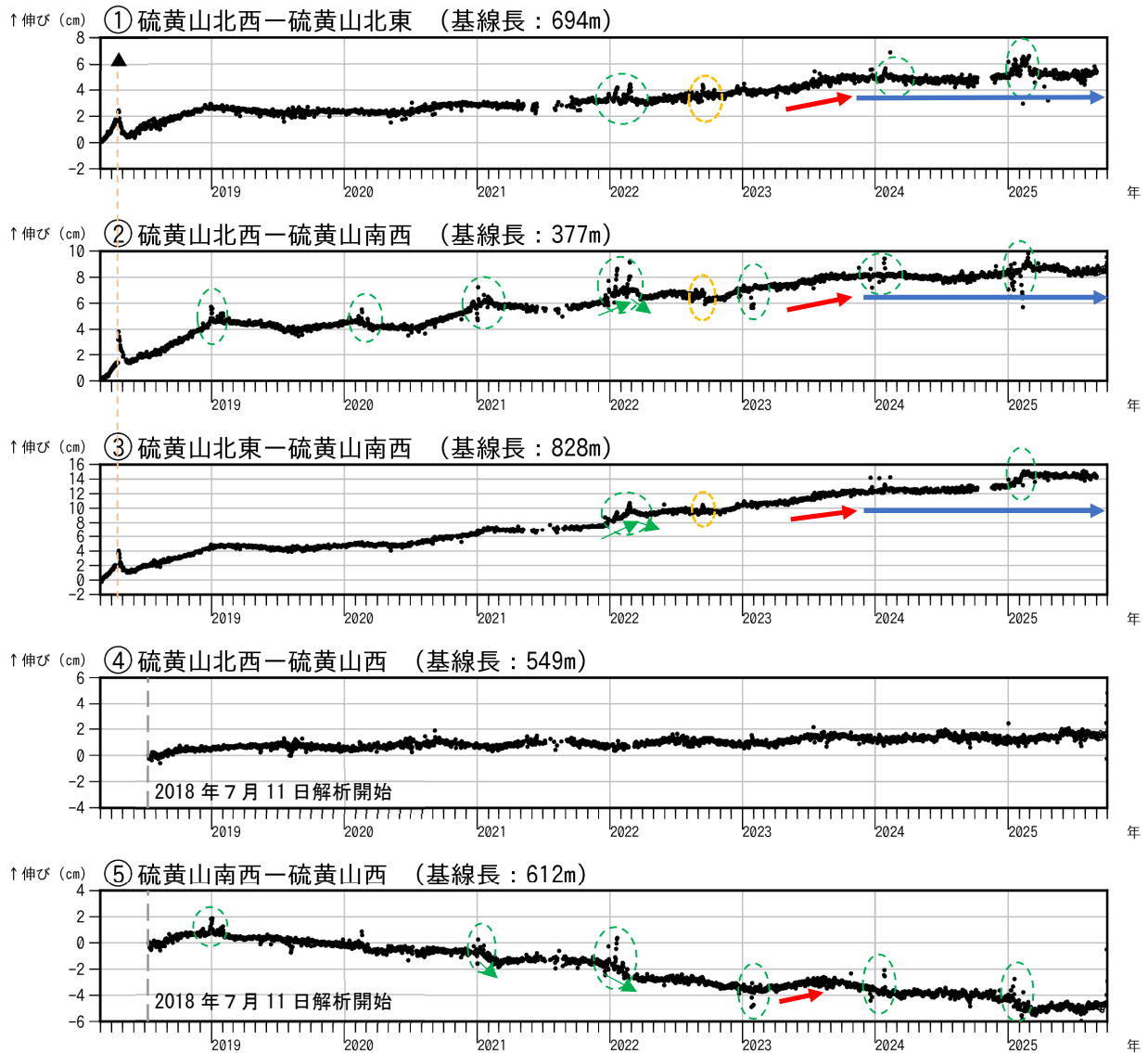
図6 霧島山（えびの高原（硫黄山）周辺） GNSS 連続観測による基線長変化（2018年3月～2025年9月）
