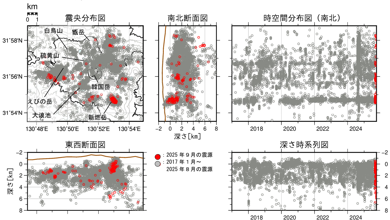
図5 霧島山（えびの高原（硫黄山）周辺）震源分布図（2017年1月～2025年9月）
